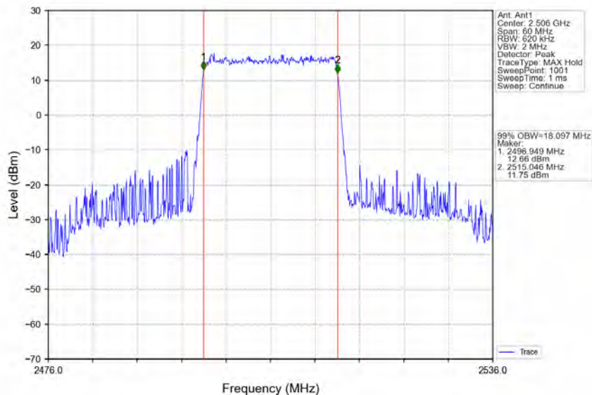
Band41_20MHz_QPSK_LCH_2506MHz_RB_100_0_NTNV
