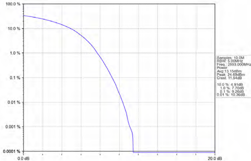
Band41_20MHz_16QAM_MCH_2593MHz_RB_100_0_NTNV
