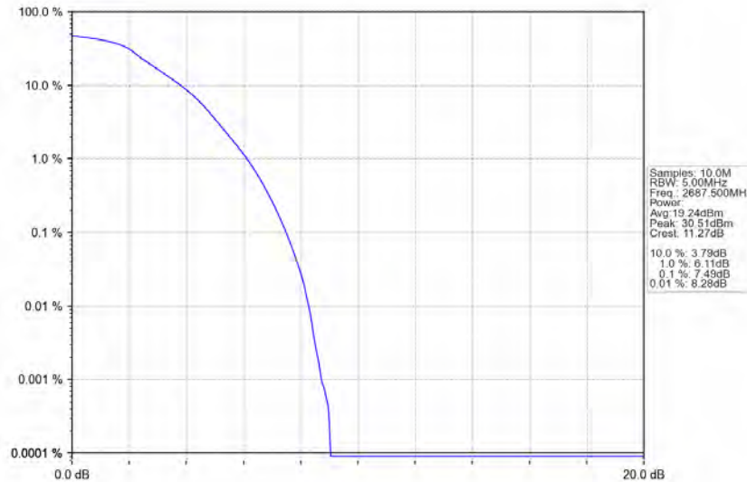
Band41_5MHz_QPSK_HCH_2687.5MHz_RB_25_0_NTNV
