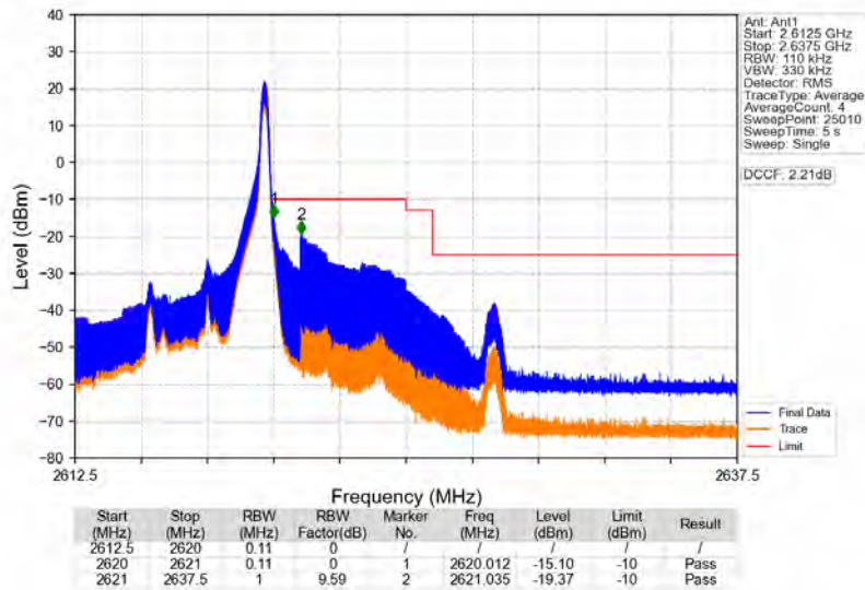
Band38_5MHz_QPSK_HCH_2617.5MHz_RB_1_24_NTNV
