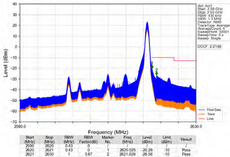
Band38_20MHz_16QAM_HCH_2610MHz_RB_1_99_NTNV
