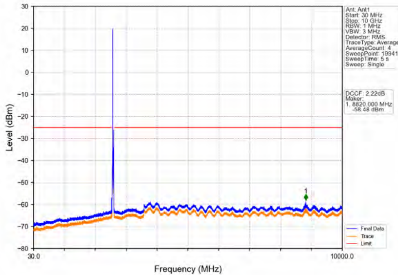
Band38_20MHz_16QAM_MCH_2595MHz_RB_1_0_NTV
