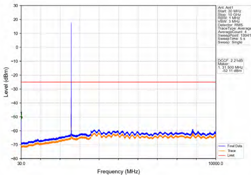
Band38_5MHz_QPSK_MCH_2595MHz_RB_1_0_NTNV
