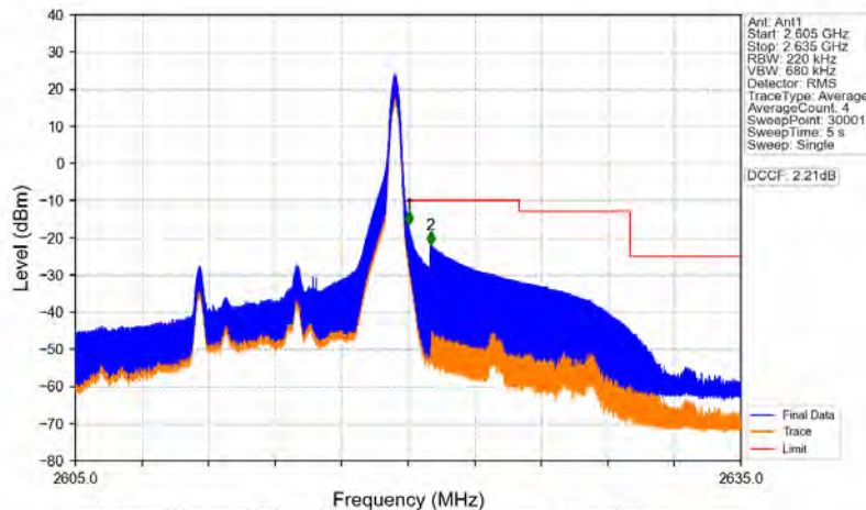
Band38_10MHz_QPSK_HCH_2615MHz_RB_1_49_NTNV
