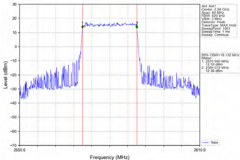
Band38_20MHz_QPSK_LCH_2580MHz_RB_100_0_NTNV
