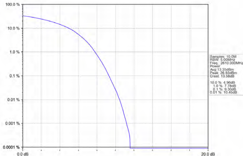
Band38_20MHz_16QAM_HCH_2610MHz_RB_100_0_NTNV
