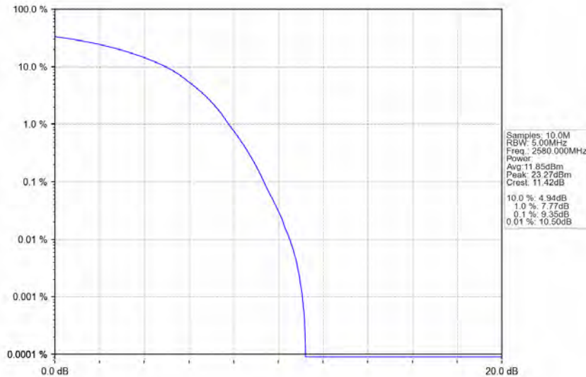
Band38_20MHz_64QAM_LCH_2580MHz_RB_100_0_NTNV
