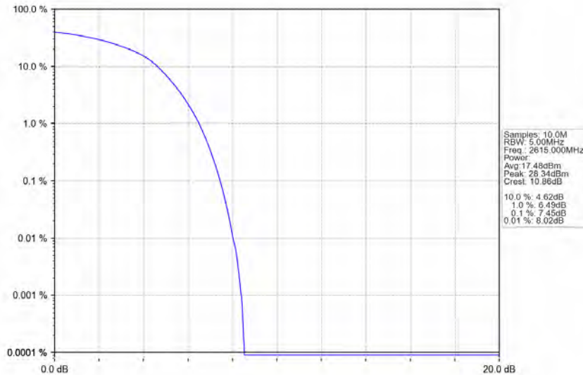
Band38_10MHz_QPSK_HCH_2615MHz_RB_50_0_NTNV
