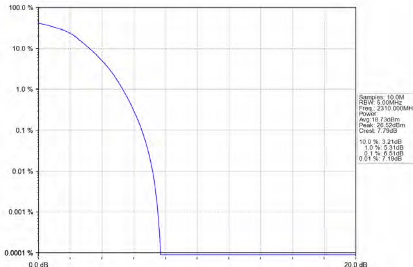
Band30_10MHz_16QAM_MCH_2310MHz_RB_50_0_NTNV
