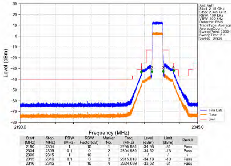
Band30_10MHz_16QAM_LCH_2310MHz_RB_1_0_NTNV
