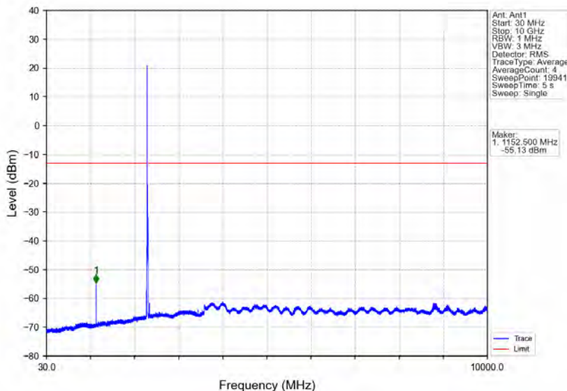
Band30_10MHz_16QAM_MCH_2310MHz_RB_1_0_NTNV
