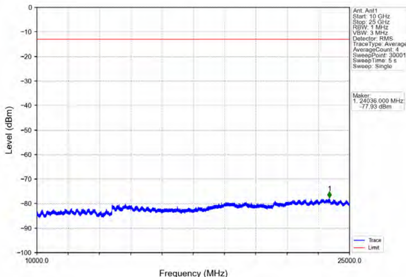
Band30_10MHz_QPSK_HCH_2310MHz_RB_1_0_NTNV
