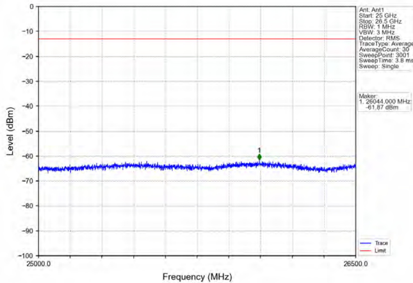
Band30_10MHz_QPSK_LCH_2310MHz_RB_1_0_NTNV
