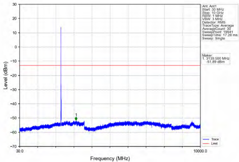
Band30_10MHz_16QAM_LCH_2310MHz_RB_1_0_NTNV
