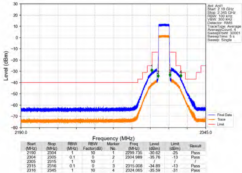
Band30_10MHz_16QAM_LCH_2310MHz_RB_50_0_NTNV
