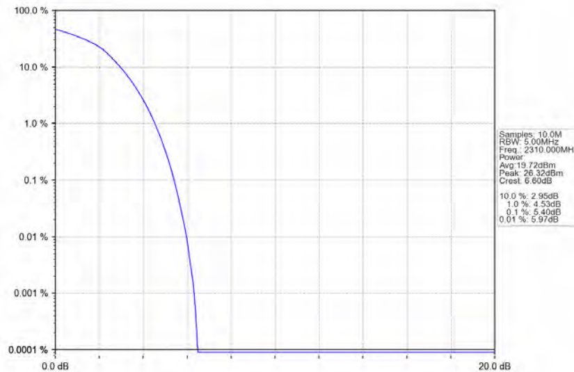
Band30_10MHz_QPSK_HCH_2310MHz_RB_50_0_NTNV
