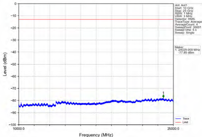
Band30_10MHz_QPSK_MCH_2310MHz_RB_1_0_NTNV
