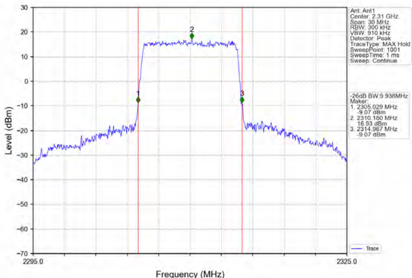
Band30_10MHz_QPSK_HCH_2310MHz_RB_50_0_NTNV
