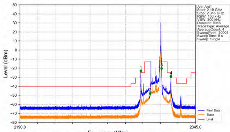
Band30_10MHz_QPSK_HCH_2310MHz_RB_1_49_NTNV
