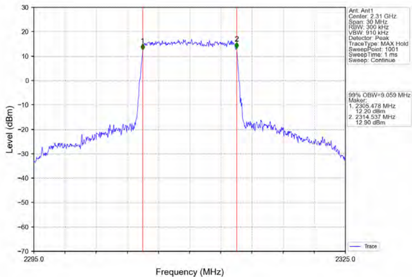
Band30_10MHz_QPSK_HCH_2310MHz_RB_50_0_NTNV
