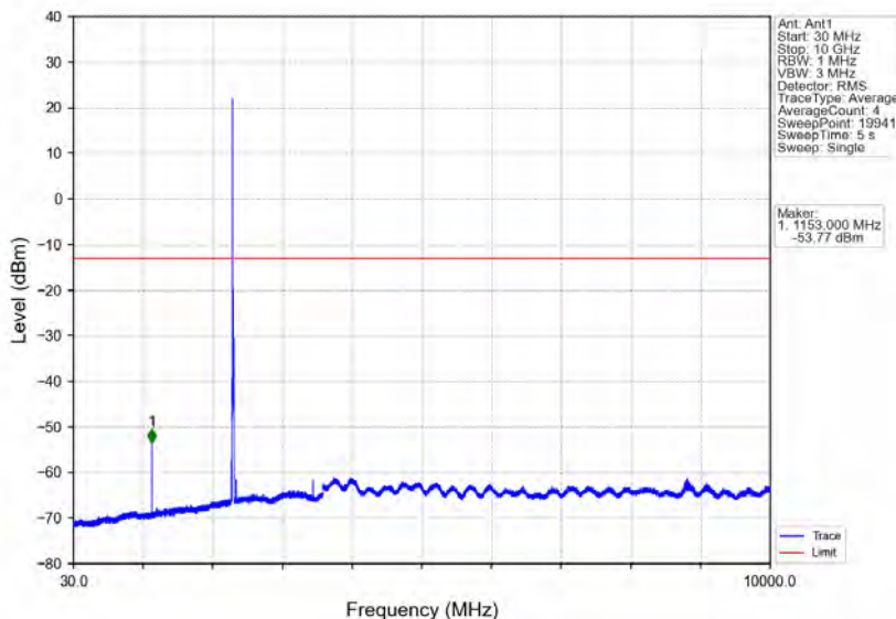
Band30_10MHz_QPSK_HCH_2310MHz_RB_1_0_NTNV
