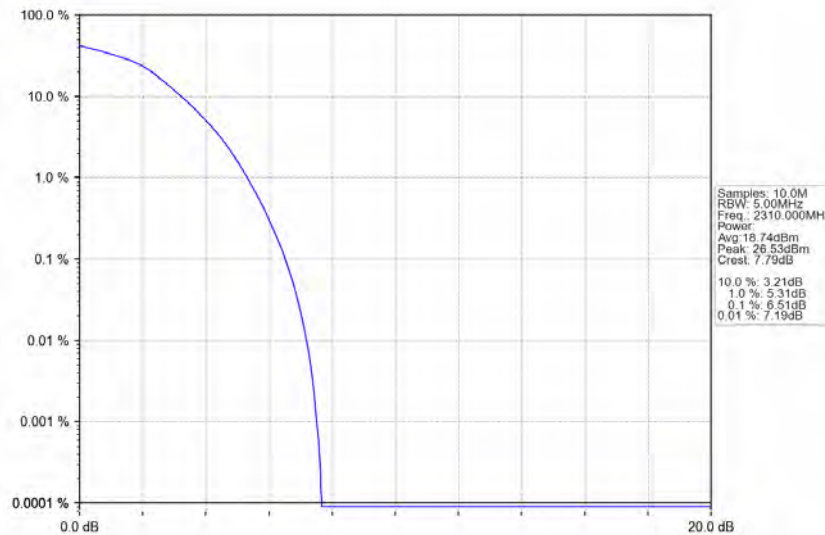
Band30_10MHz_16QAM_LCH_2310MHz_RB_50_0_NTNV
