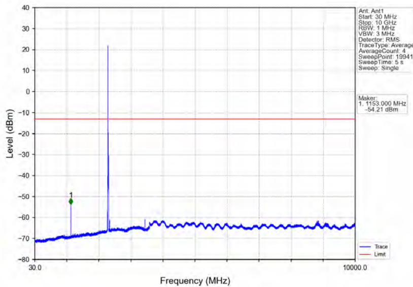
Band30_10MHz_QPSK_MCH_2310MHz_RB_1_0_NTNV
