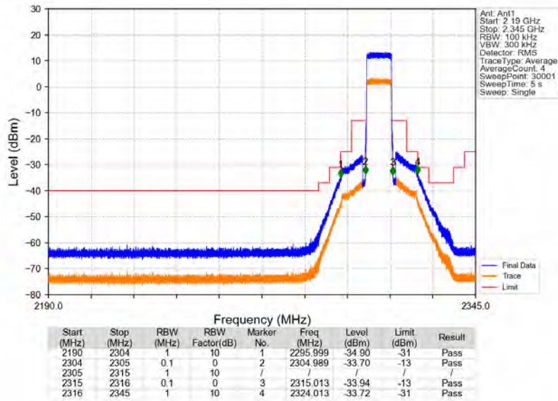
Band30_10MHz_QPSK_MCH_2310MHz_RB_1_0_NTNV
