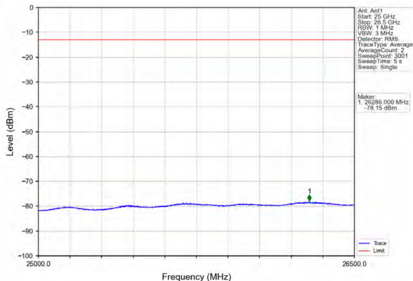
Band30_10MHz_QPSK_HCH_2310MHz_RB_1_49_NTNV
