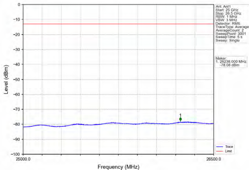
Band30_10MHz_QPSK_MCH_2310MHz_RB_1_0_NTNV
