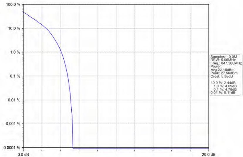
Band26b_3MHz_QPSK_HCH_847.5MHz_RB_15_0_NTNV
