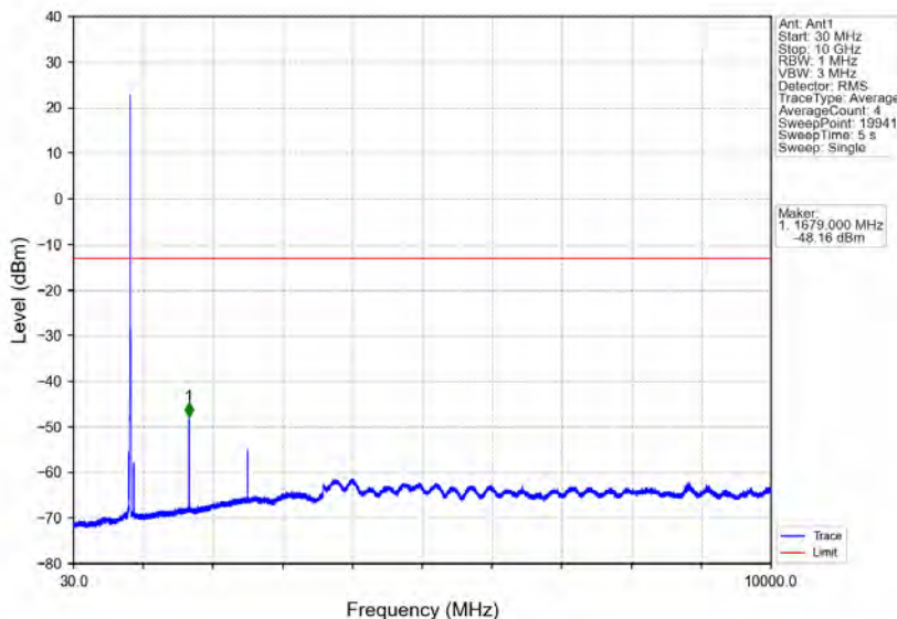
Band26b_10MHz_QPSK_HCH_844MHz_RB_1_49_NTNV
