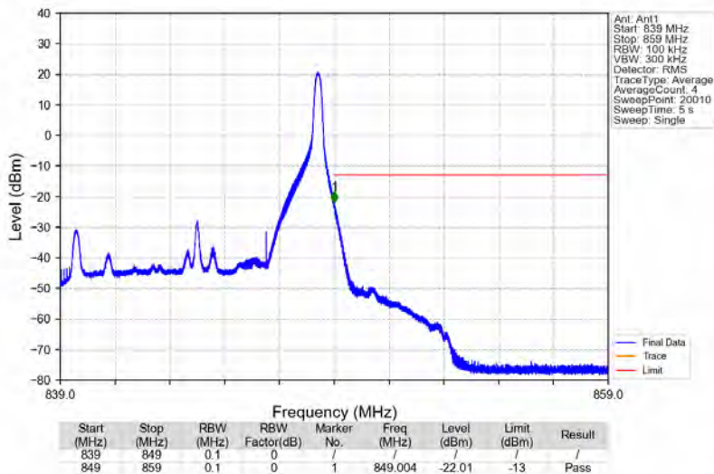
Band26b_10MHz_QPSK_HCH_844MHz_RB_1_49_NTNV
