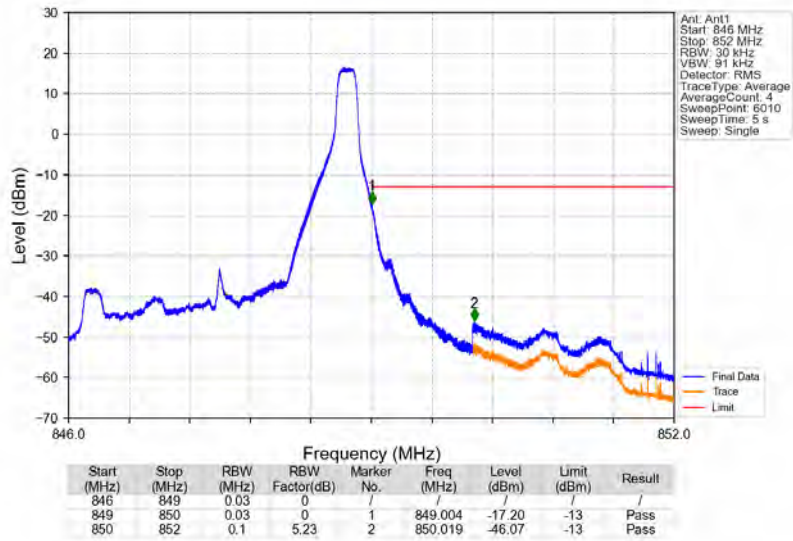
Band26b_3MHz_QPSK_HCH_847.5MHz_RB_1_14_NTNV
