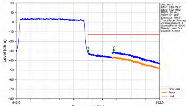
Band26b_3MHz_QPSK_HCH_847.5MHz_RB_15_0_NTNV
