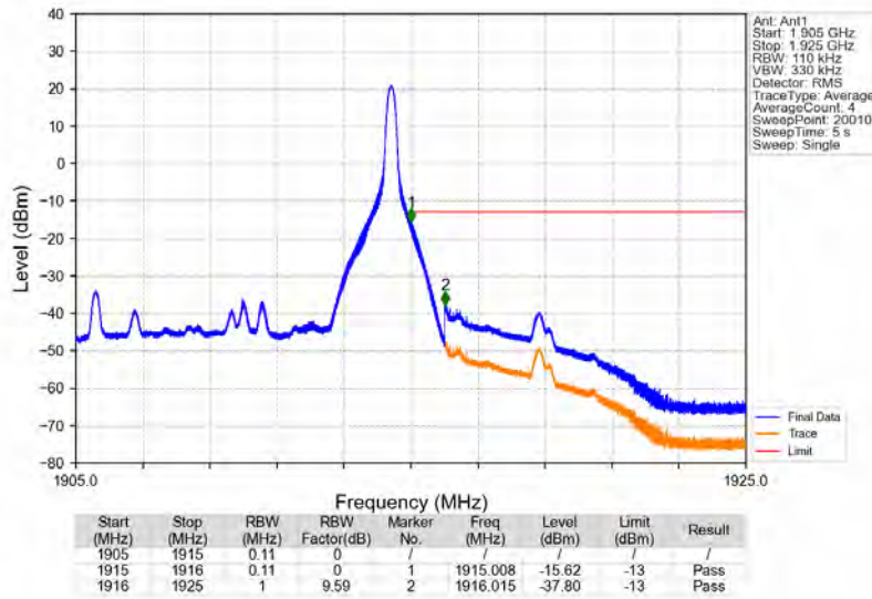
Band25_10MHz_QPSK_HCH_1910MHz_RB_1_49_NTV
