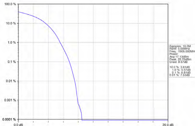
Band25_20MHz_QPSK_HCH_1905MHz_RB_100_0_NTNV
