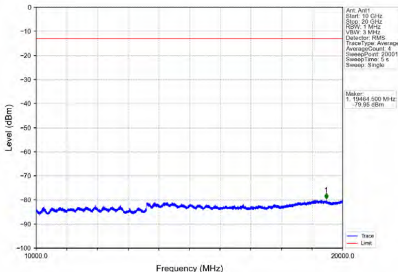
Band25_10MHz_QPSK_HCH_1910MHz_RB_1_0_NTNV
