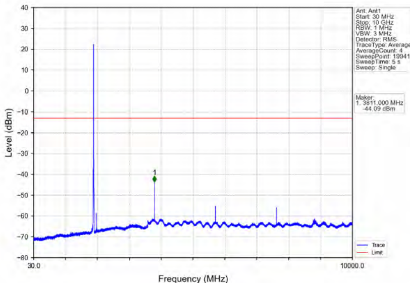
Band25_10MHz_QPSK_HCH_1910MHz_RB_1_0_NTNV
