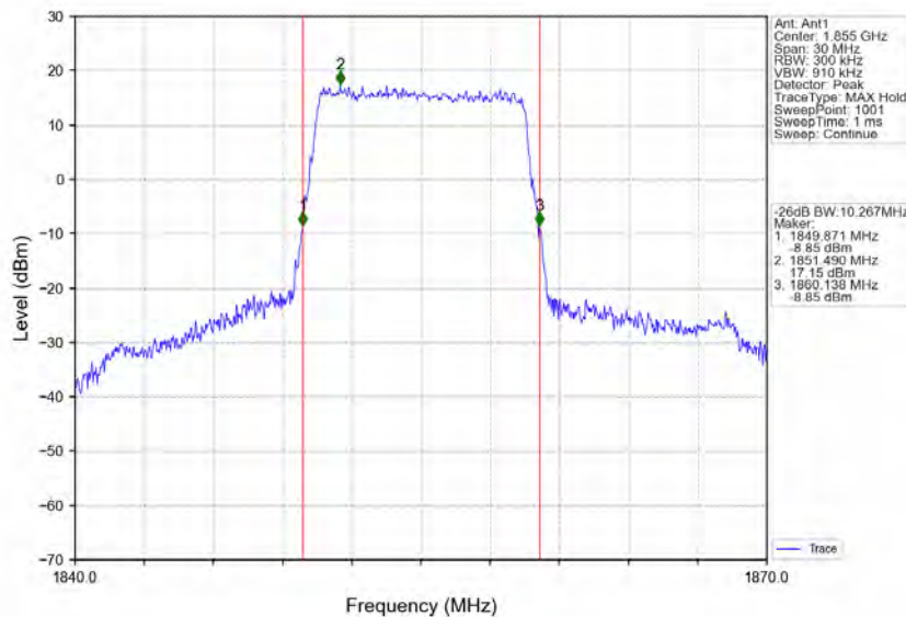
Band25_10MHz_QPSK_LCH_1855MHz_RB_50_0_NTNV
