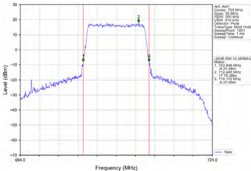
Band17_10MHz_QPSK_LCH_709MHz_RB_50_0_NTNV
