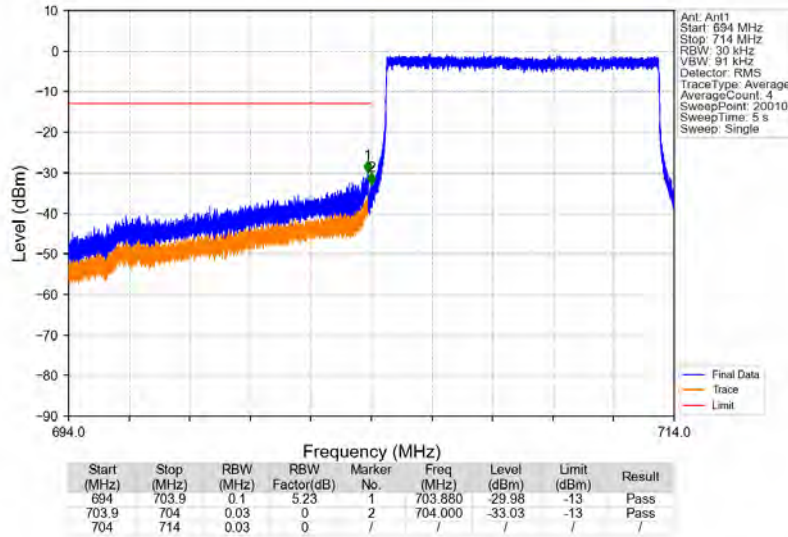
Band17_10MHz_QPSK_LCH_709MHz_RB_50_0_NTNV
