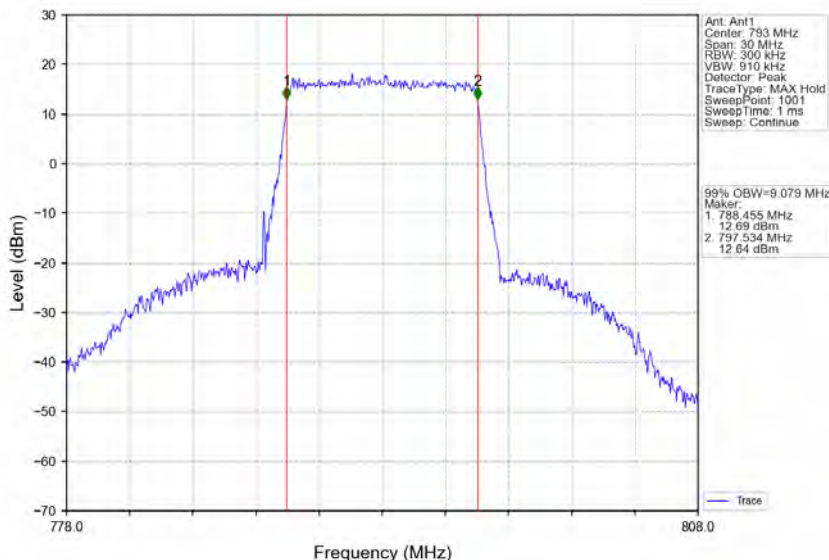
Band14_10MHz_QPSK_LCH_793MHz_RB_50_0_NTNV
