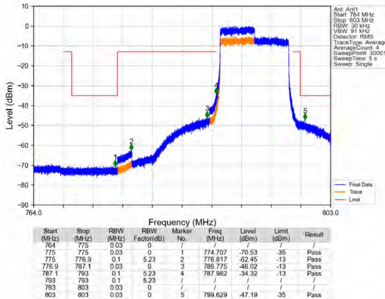
Band14_10MHz_QPSK_MCH_793MHz_RB_1_0_NTNV
