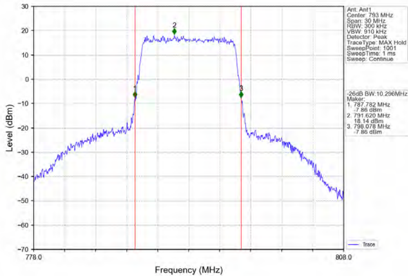
Band14_10MHz_QPSK_HCH_793MHz_RB_50_0_NTNV
