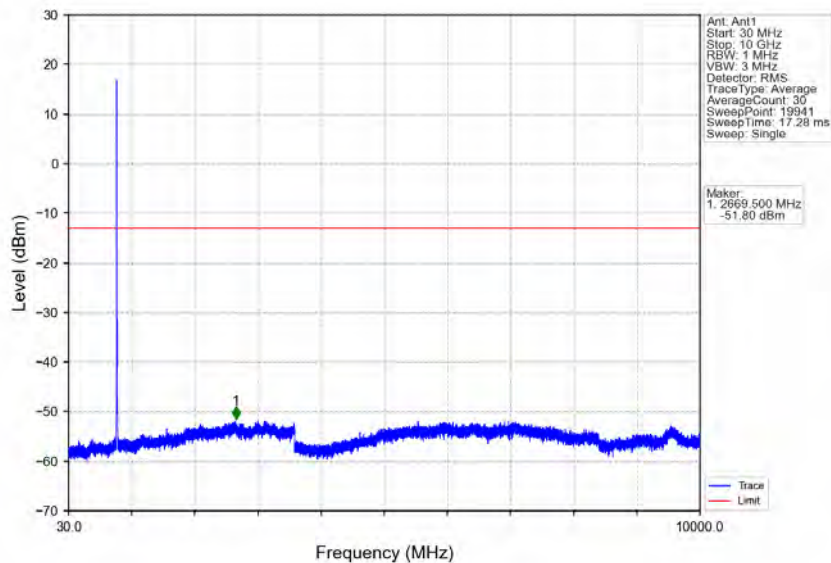
Band14_10MHz_QPSK_MCH_793MHz_RB_1_0_NTNV
