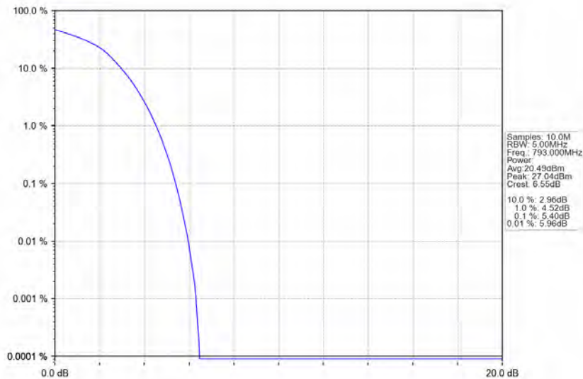
Band14_10MHz_QPSK_HCH_793MHz_RB_50_0_NTNV
