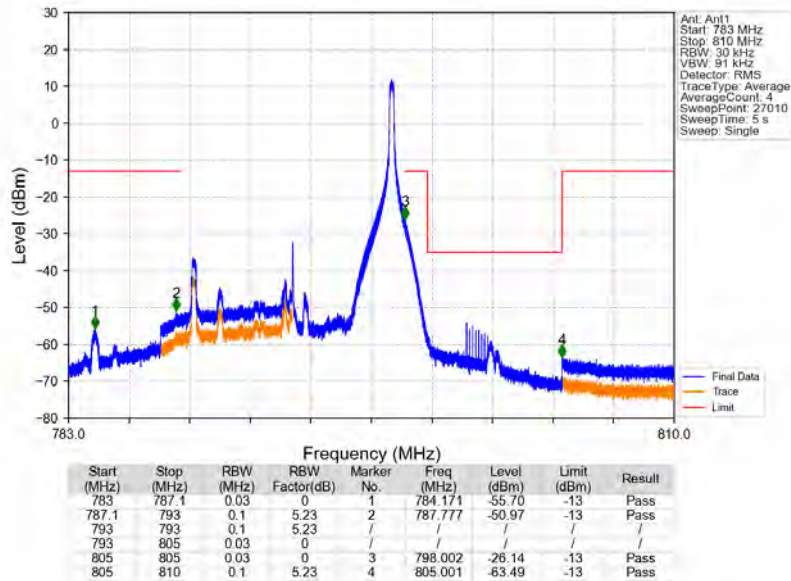
Band14_10MHz_QPSK_HCH_793MHz_RB_1_49_NTNV
