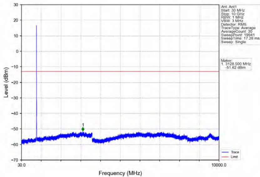
Band14_10MHz_QPSK_HCH_793MHz_RB_1_49_NTNV
