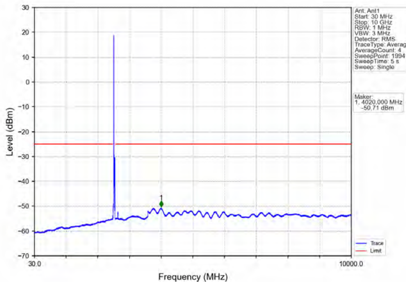
Band7_20MHz_64QAM_MCH_2535MHz_RB_1_0_NTNV
