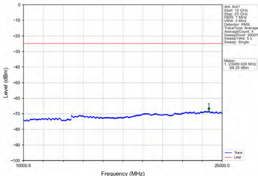
Band7_20MHz_16QAM_LCH_2510MHz_RB_1_0_NTNV
