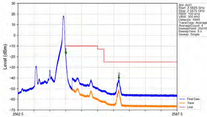
Band7_5MHz_QPSK_HCH_2567.5MHz_RB_1_24_NTNV
