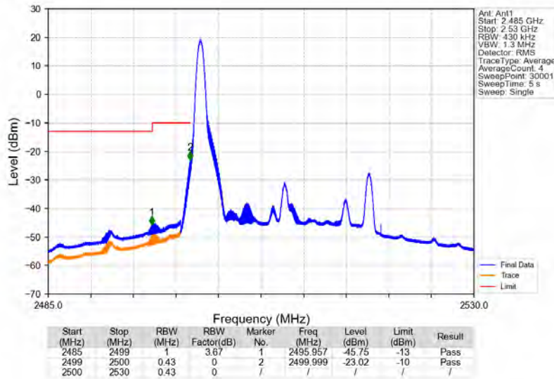
Band7_20MHz_64QAM_LCH_2510MHz_RB_1_0_NTNV
