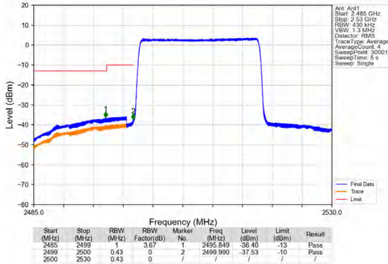
Band7_20MHz_64QAM_LCH_2510MHz_RB_100_0_NTNV
