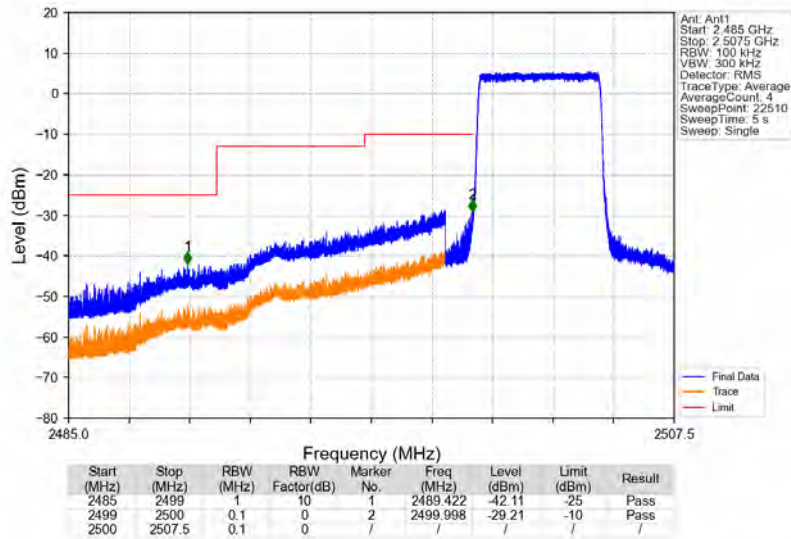
Band7_5MHz_QPSK_LCH_2502.5MHz_RB_25_0_NTNV
