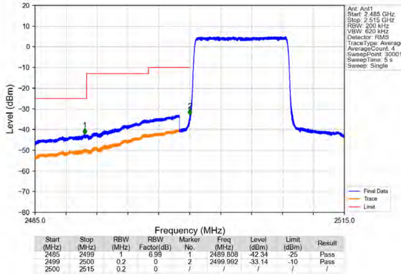
Band7_10MHz_QPSK_LCH_2505MHz_RB_50_0_NTNV
