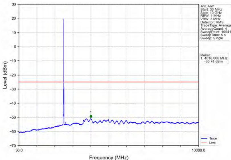
Band7_20MHz_16QAM_LCH_2510MHz_RB_1_0_NTNV
