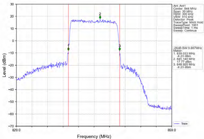
Band5_10MHz_QPSK_HCH_844MHz_RB_50_0_NTNV
