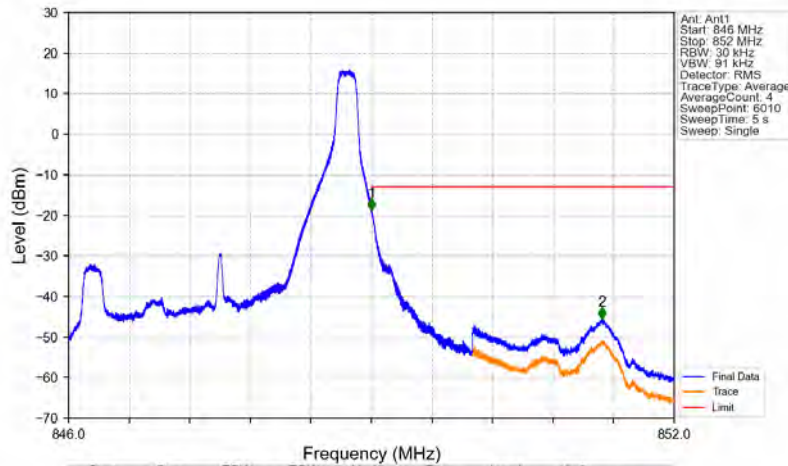
Band5_3MHz_QPSK_HCH_847.5MHz_RB_1_14_NTNV
