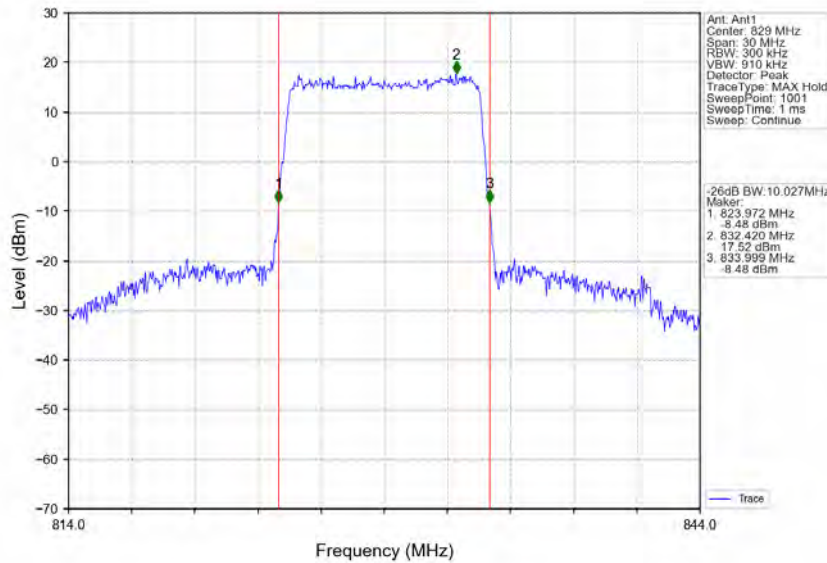
Band5_10MHz_QPSK_LCH_829MHz_RB_50_0_NTNV
