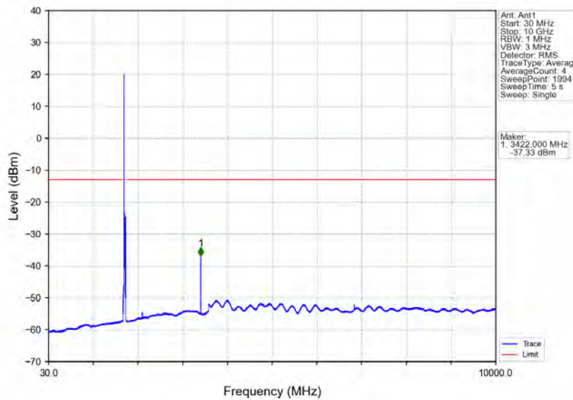
Band4_20MHz_16QAM_LCH_1720MHz_RB_1_0_NTNV
