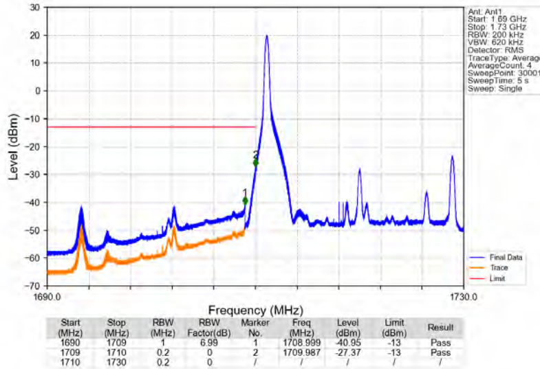
Band4_20MHz_16QAM_LCH_1720MHz_RB_1_0_NTNV
