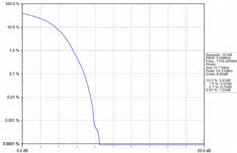
Band4_20MHz_QPSK_HCH_1745MHz_RB_100_0_NTNV
