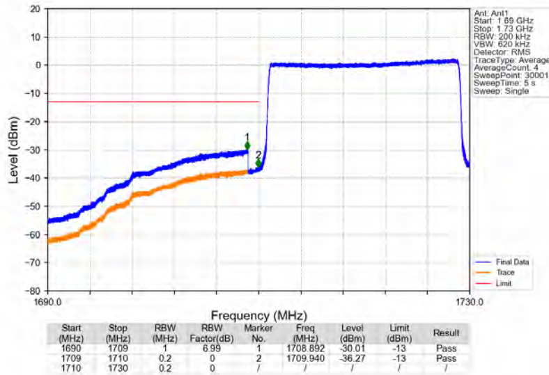
Band4_20MHz_16QAM_LCH_1720MHz_RB_100_0_NTNV
