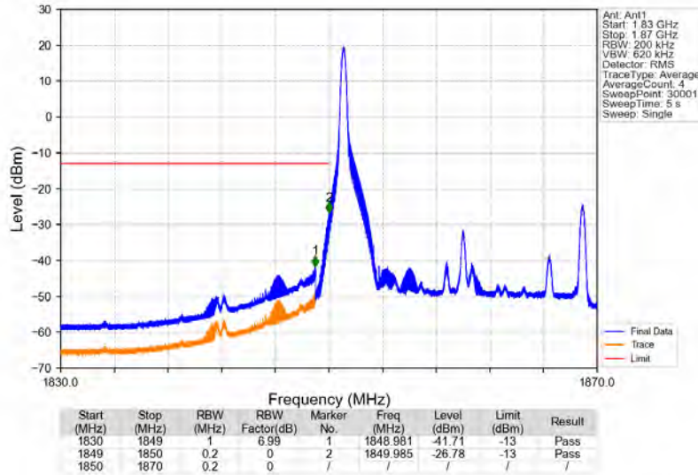
Band2_20MHz_64QAM_LCH_1860MHz_RB_1_0_NTNV
