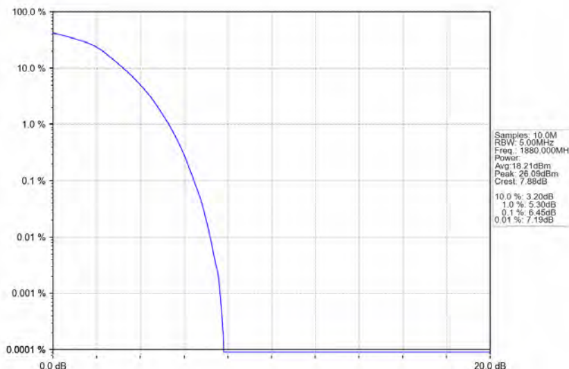
Band2_10MHz_16QAM_MCH_1880MHz_RB_50_0_NTNV
