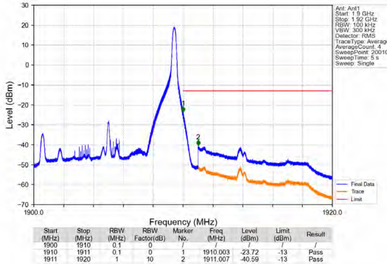
Band2_10MHz_16QAM_HCH_1905MHz_RB_1_49_NTNV
