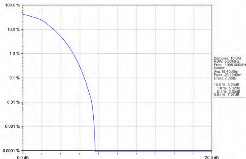
Band2_10MHz_16QAM_HCH_1905MHz_RB_50_0_NTNV
