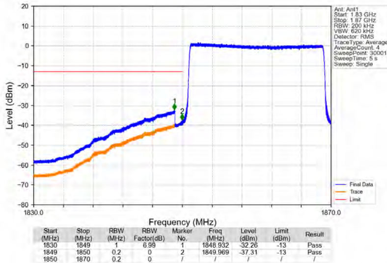
Band2_20MHz_64QAM_LCH_1860MHz_RB_100_0_NTNV
