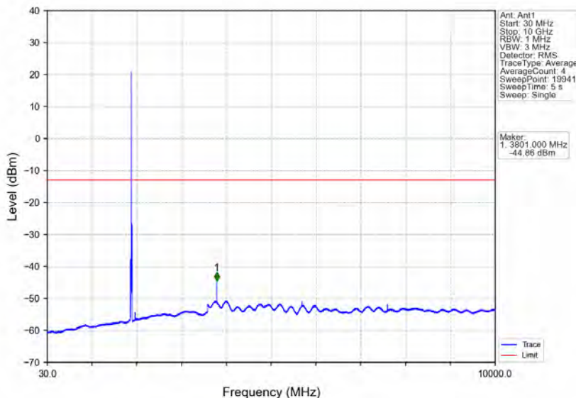
Band2_10MHz_16QAM_HCH_1905MHz_RB_1_0_NTNV
