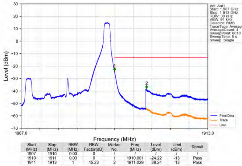
Band2_3MHz_QPSK_HCH_1908.5MHz_RB_1_14_NTNV
