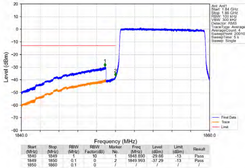
Band2_10MHz_64QAM_LCH_1855MHz_RB_50_0_NTV
