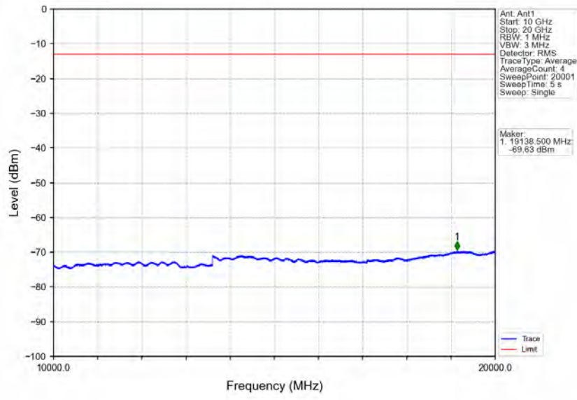
Band2_20MHz_16QAM_MCH_1880MHz_RB_1_0_NTNV
