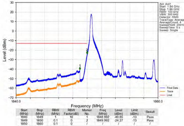
Band2_10MHz_64QAM_LCH_1855MHz_RB_1_0_NTNV
