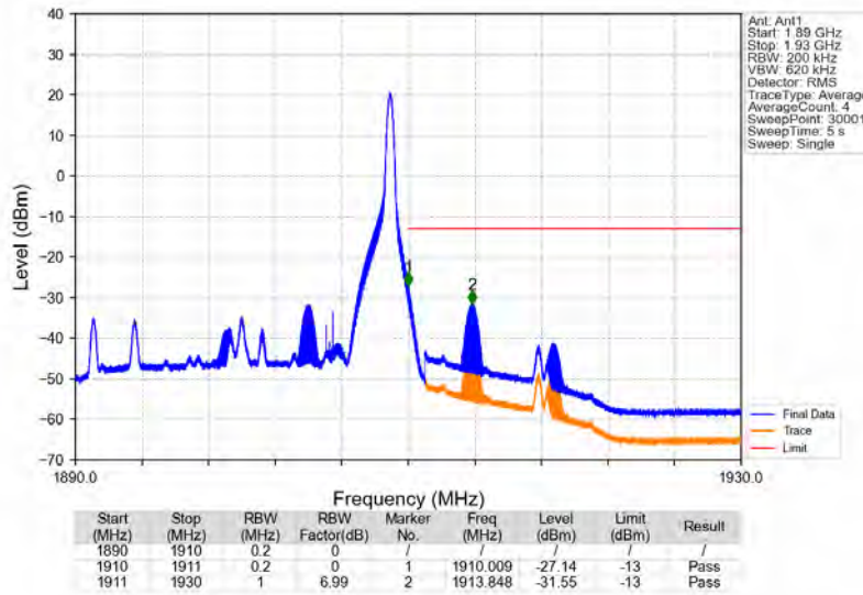
Band2_20MHz_16QAM_HCH_1900MHz_RB_1_99_NTNV
