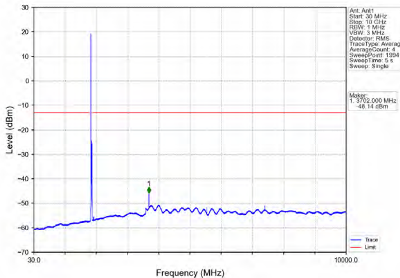
Band2_20MHz_64QAM_LCH_1860MHz_RB_1_0_NTNV
