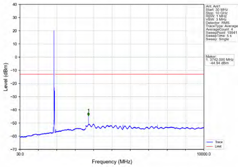
Band2_20MHz_16QAM_MCH_1880MHz_RB_1_0_NTNV
