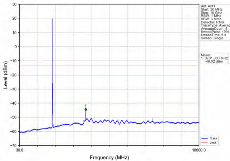
Band2_10MHz_64QAM_LCH_1855MHz_RB_1_0_NTNV
