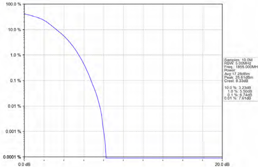
Band2_10MHz_64QAM_LCH_1855MHz_RB_50_0_NTNV
