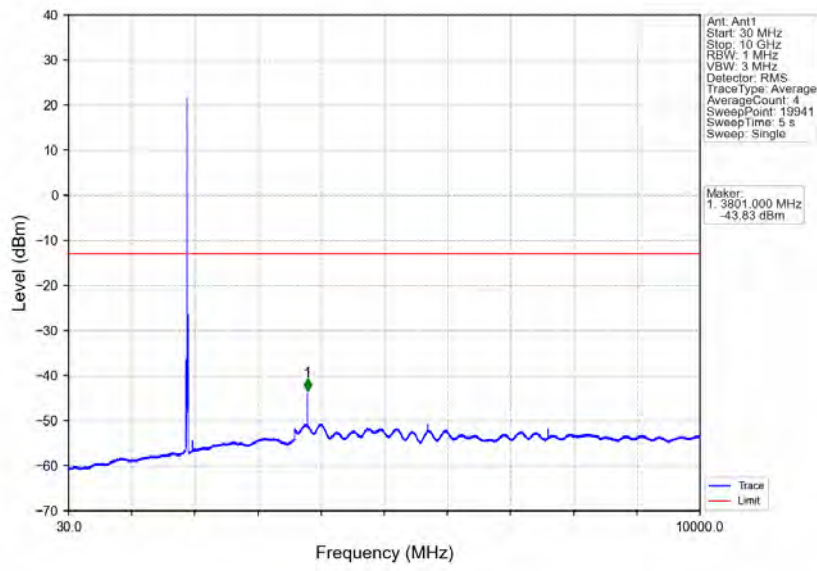
Band2_10MHz_QPSK_HCH_1905MHz_RB_1_0_NTNV
