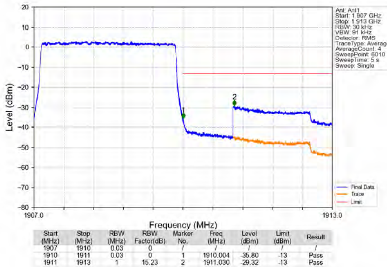
Band2_3MHz_QPSK_HCH_1908.5MHz_RB_15_0_NTNV
