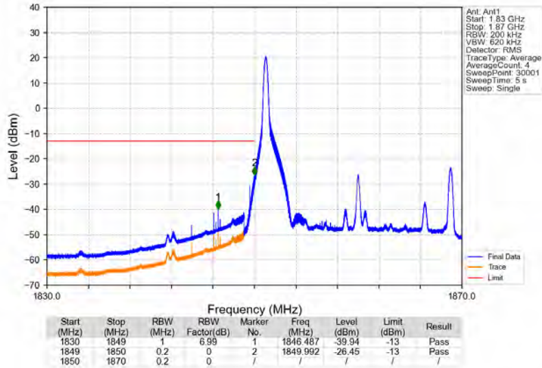
Band2_20MHz_16QAM_LCH_1860MHz_RB_1_0_NTNV
