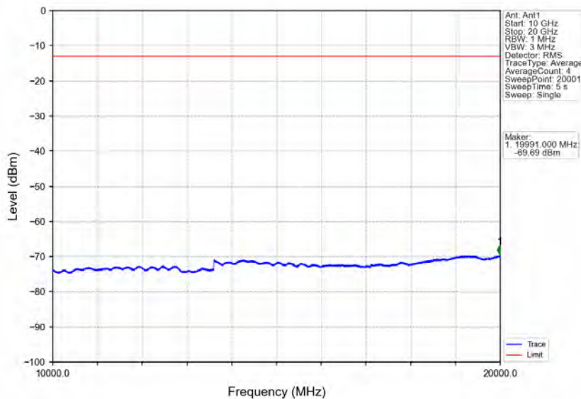
Band2_10MHz_16QAM_HCH_1905MHz_RB_1_0_NTNV
