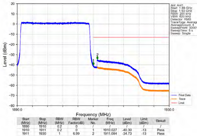
Band2_20MHz_16QAM_HCH_1900MHz_RB_100_0_NTNV
