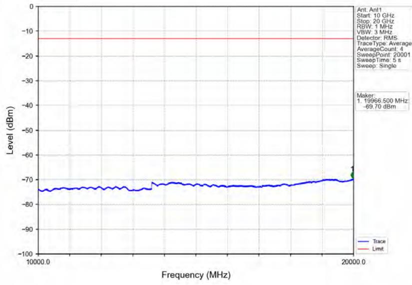
Band2_10MHz_QPSK_HCH_1905MHz_RB_1_0_NTNV
