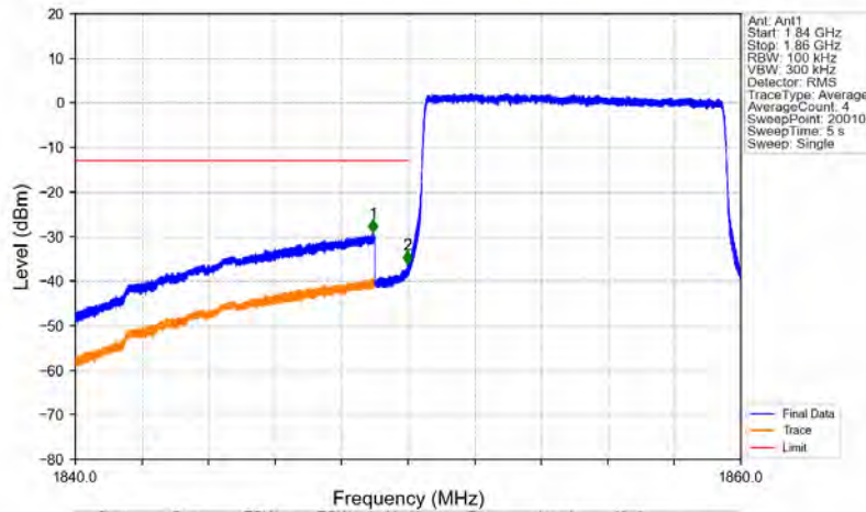
Band2_10MHz_16QAM_LCH_1855MHz_RB_50_0_NTV
