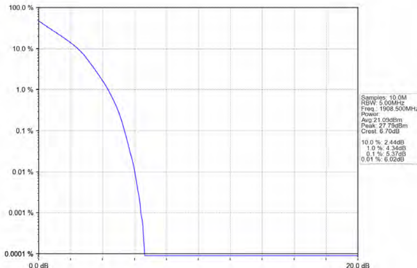
Band2_3MHz_QPSK_HCH_1908.5MHz_RB_15_0_NTNV
