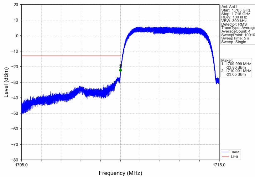
Band4_HSUPA_LCH_1712.4MHz_Subtest 1_NTNV
