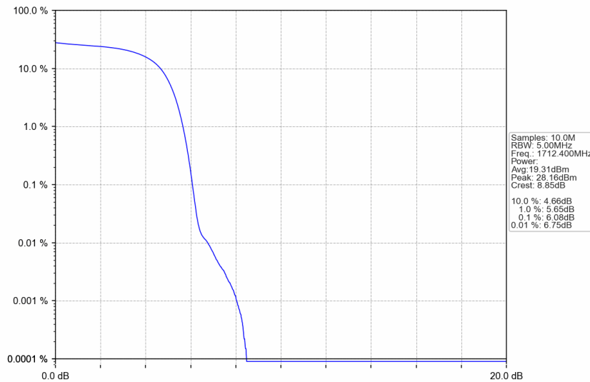
Band4_HSUPA_LCH_1712.4MHz_Subtest 1_NTNV
