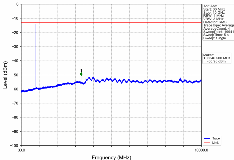
GSM850_GSM_HCH_848.8MHz_GSM_NTNV
