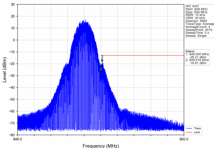
GSM850_GSM_HCH_848.8MHz_GSM_NTNV
