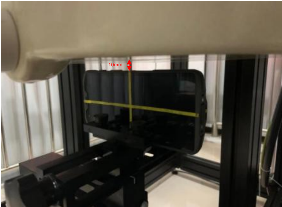
Body-Right(10mm)
