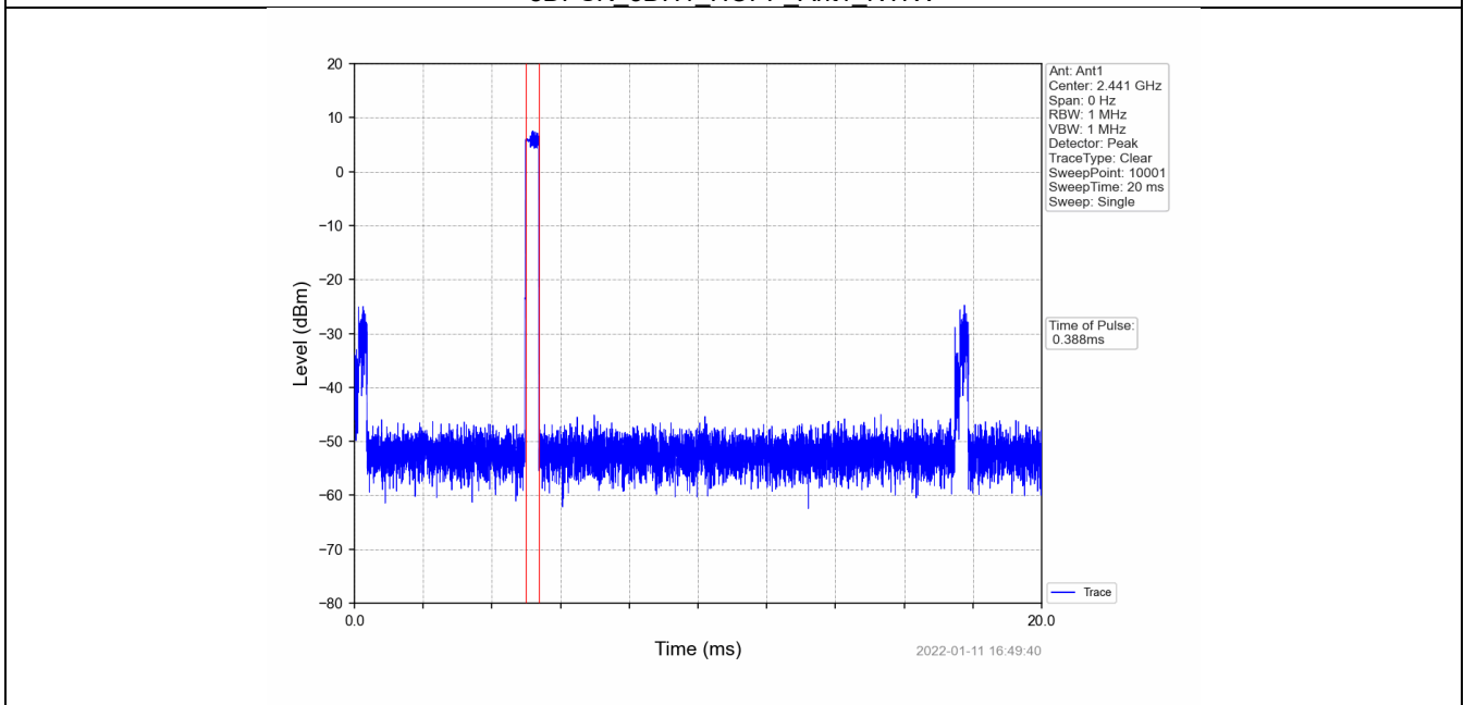
8DPSK_3DH1_HOPP_Ant1_NTNV
