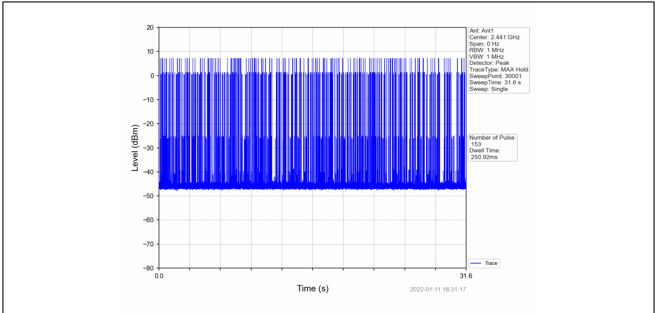
Pi/4DQPSK_2DH5_HOPP_Ant1_NTNV
