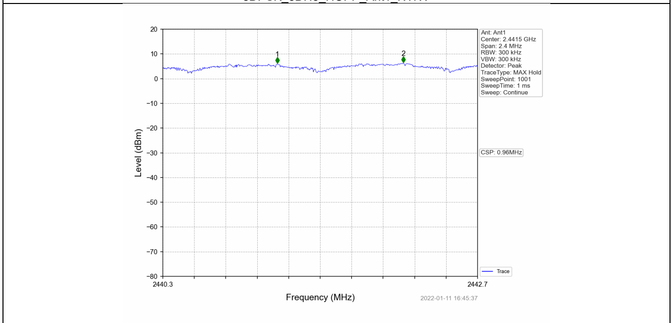
8DPSK_3DH5_HOPP_Ant1_NTNV
