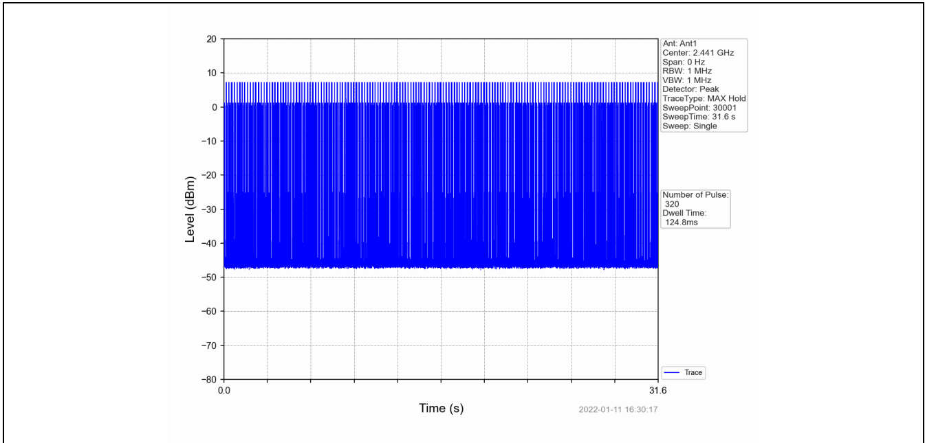
Pi/4DQPSK_2DH3_HOPP_Ant1_NTNV
