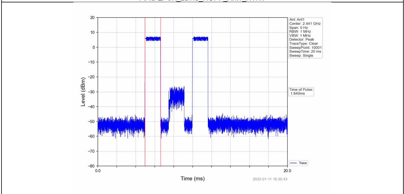
Pi/4DQPSK_2DH3_HOPP_Ant1_NTNV
