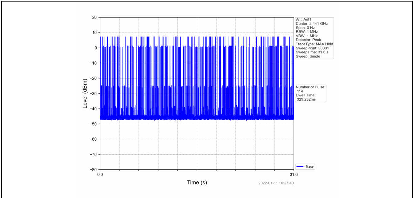
8DPSK_3DH1_HOPP_Ant1_NTNV
