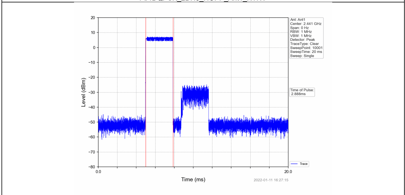
Pi/4DQPSK_2DH5_HOPP_Ant1_NTNV
