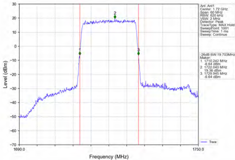
Band66_20MHz_QPSK_LCH_1720MHz_RB_100_0_NTNV
