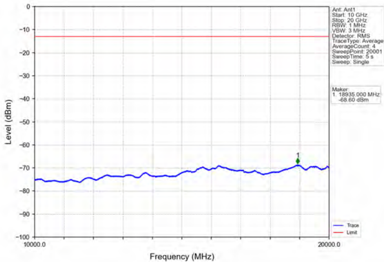
Band66_20MHz_QPSK_HCH_1770MHz_RB_1_0_NTNV
