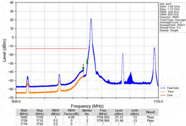
Band66_20MHz_16QAM_LCH_1720MHz_RB_1_0_NTNV
