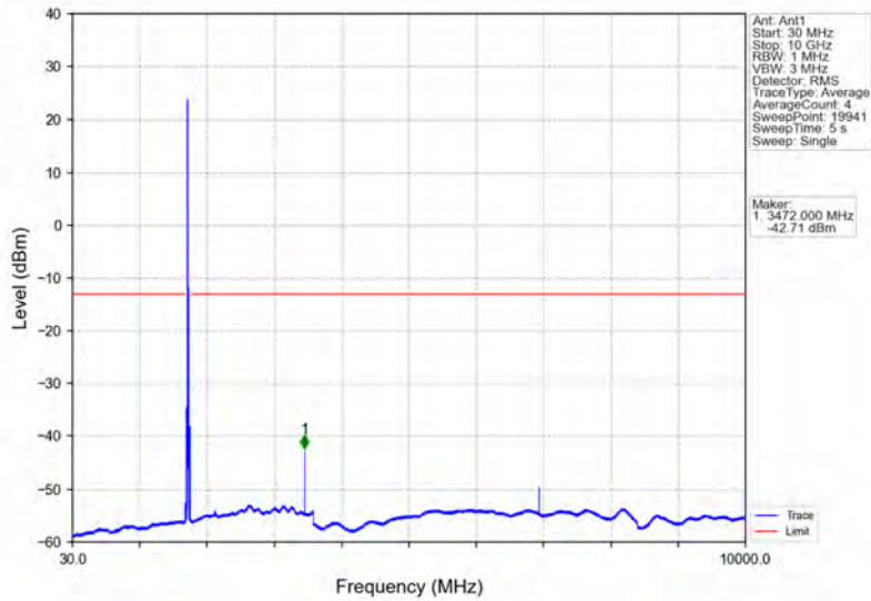
Band66_20MHz_QPSK_MCH_1745MHz_RB_1_0_NTNV
