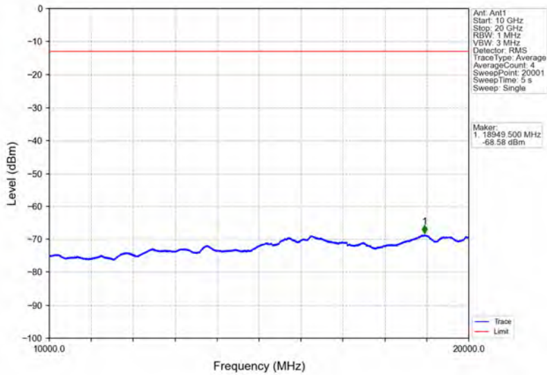
Band66_20MHz_QPSK_LCH_1720MHz_RB_100_0_NTNV
