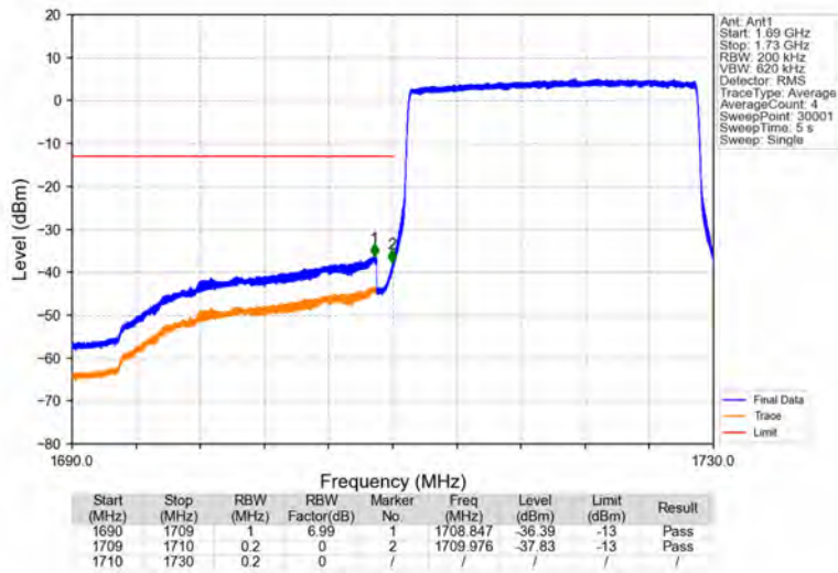
Band66_20MHz_QPSK_LCH_1720MHz_RB_100_0_NTNV
