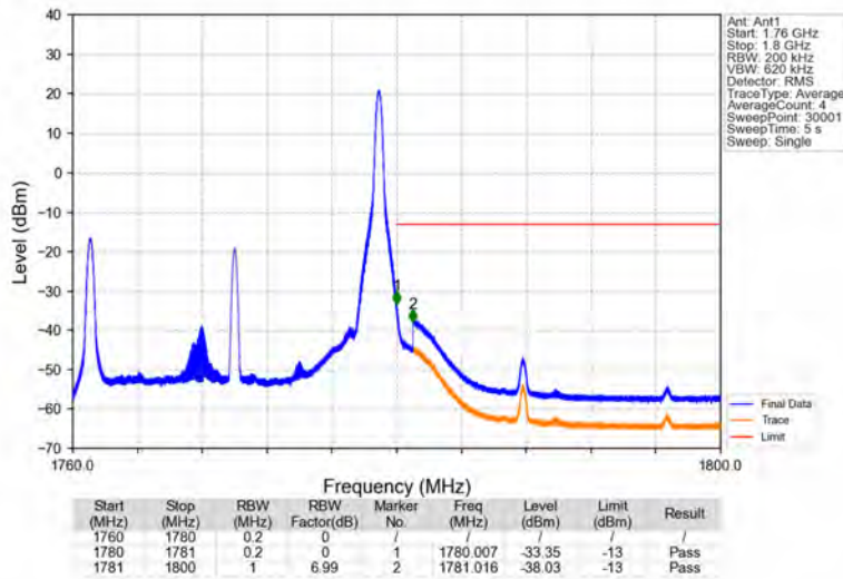
Band66_20MHz_QPSK_HCH_1770MHz_RB_1_99_NTNV
