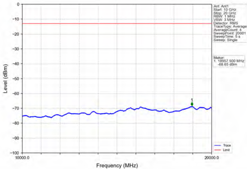
Band66_20MHz_QPSK_MCH_1745MHz_RB_1_0_NTNV
