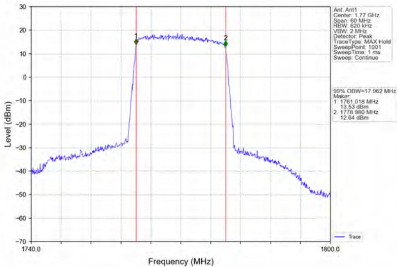
Band66_20MHz_QPSK_HCH_1770MHz_RB_100_0_NTNV
