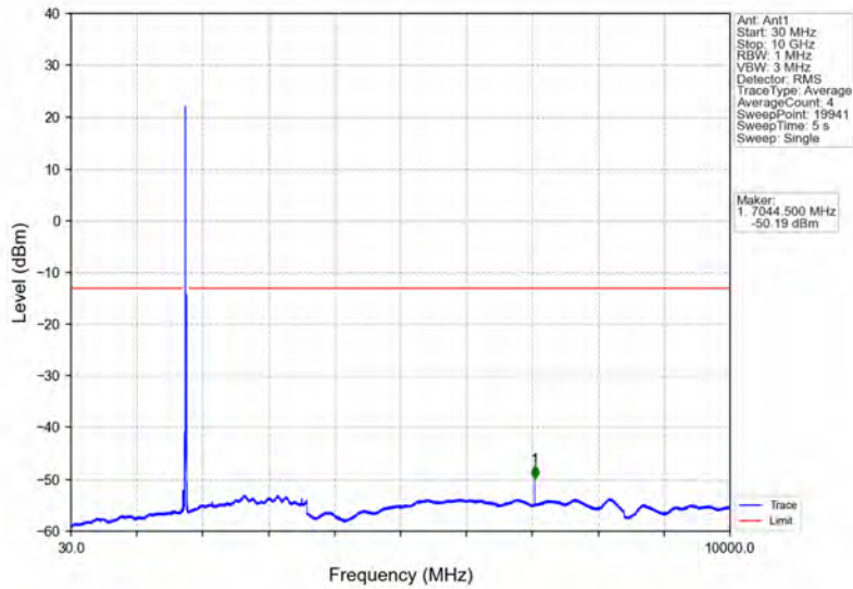
Band66_20MHz_QPSK_HCH_1770MHz_RB_1_0_NTNV
