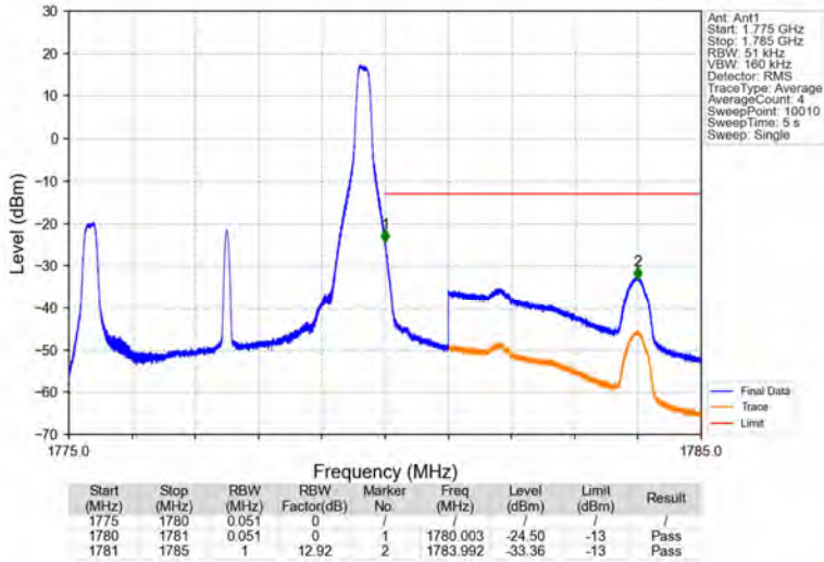
Band66_5MHz_QPSK_HCH_1777.5MHz_RB_1_24_NTNV
