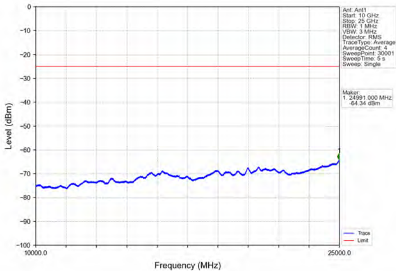
Band41_10MHz_QPSK_HCH_2685MHz_RB_1_0_NTNV
