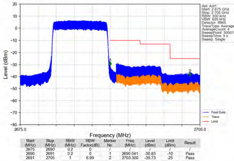
Band41_10MHz_QPSK_HCH_2685MHz_RB_50_0_NTNV
