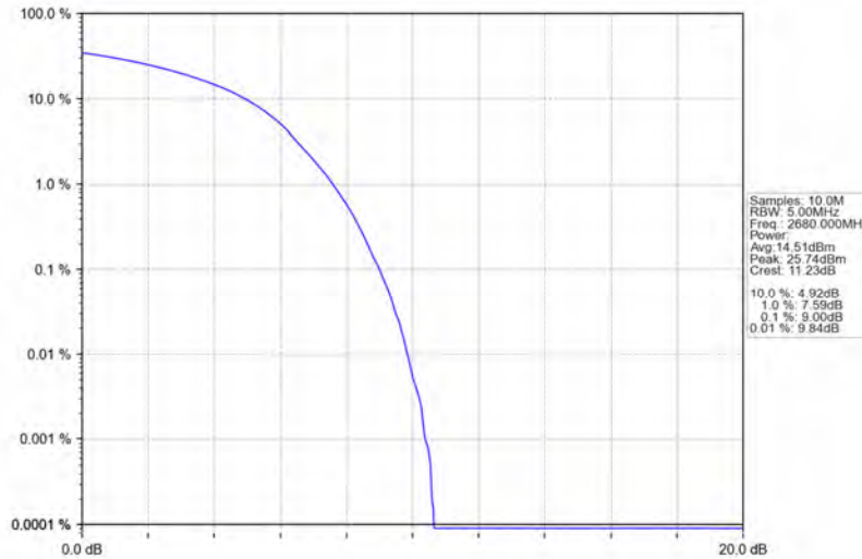
Band41_20MHz_QPSK_HCH_2680MHz_RB_100_0_NTNV
