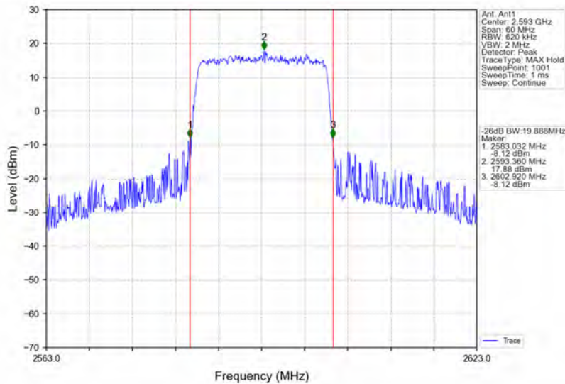
Band41_20MHz_16QAM_MCH_2593MHz_RB_100_0_NTNV
