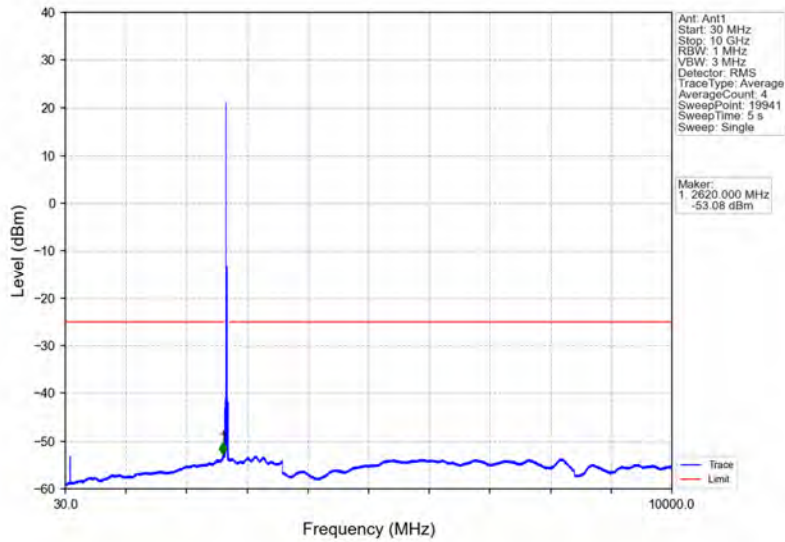
Band41_20MHz_QPSK_HCH_2680MHz_RB_1_0_NTNV
