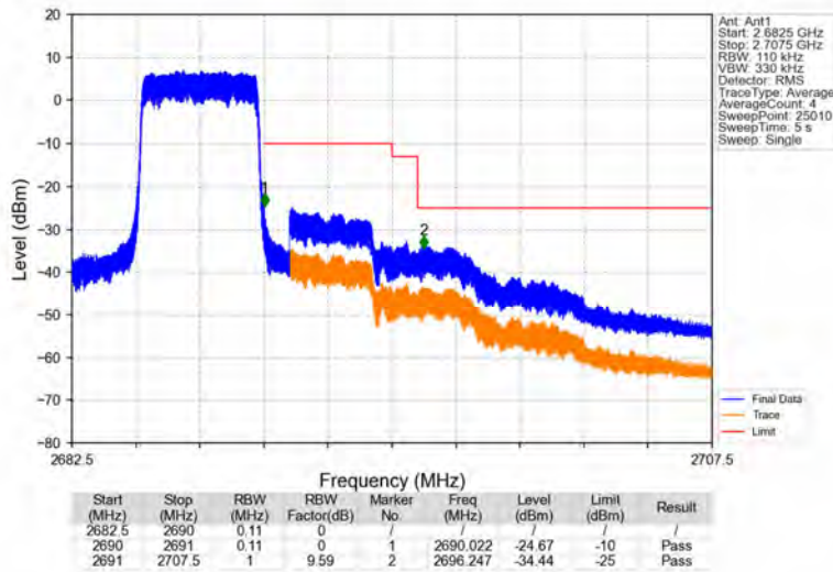
Band41_5MHz_QPSK_HCH_2687.5MHz_RB_25_0_NTNV
