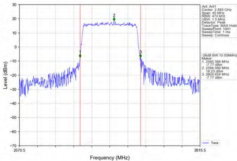
Band41_15MHz_QPSK_MCH_2593MHz_RB_75_0_NTNV
