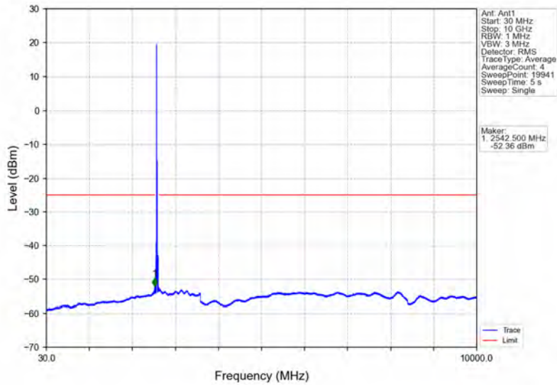
Band41_20MHz_16QAM_MCH_2593MHz_RB_1_0_NTNV
