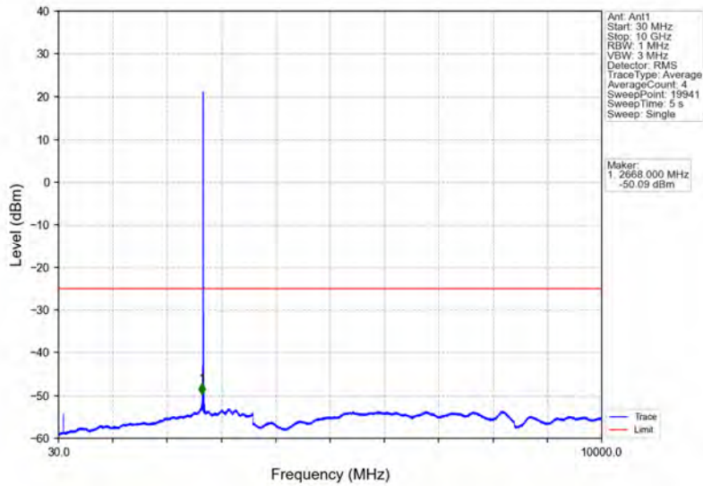
Band41_5MHz_QPSK_HCH_2687.5MHz_RB_1_0_NTNV
