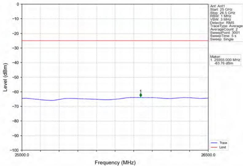
Band41_20MHz_QPSK_LCH_2506MHz_RB_1_0_NTNV
