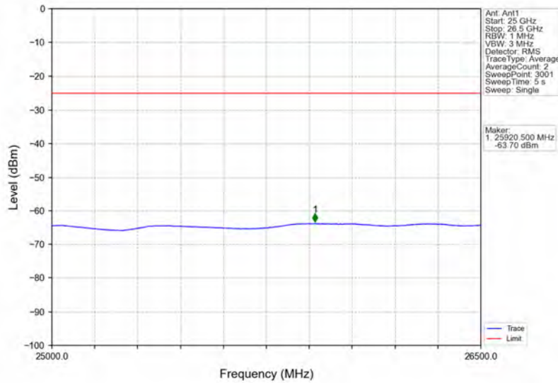
Band41_5MHz_QPSK_HCH_2687.5MHz_RB_1_24_NTNV
