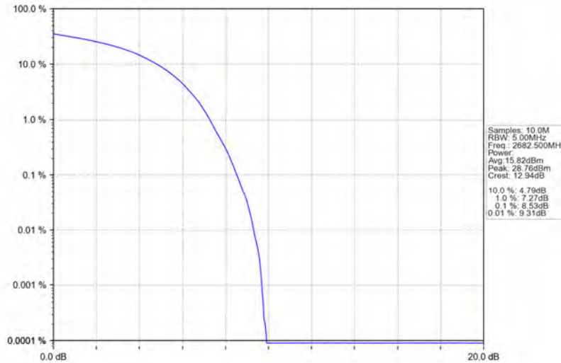
Band41_15MHz_QPSK_HCH_2682.5MHz_RB_75_0_NTNV
