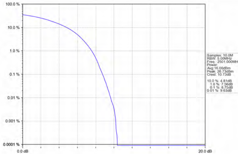
Band41_10MHz_16QAM_LCH_2501MHz_RB_50_0_NTNV
