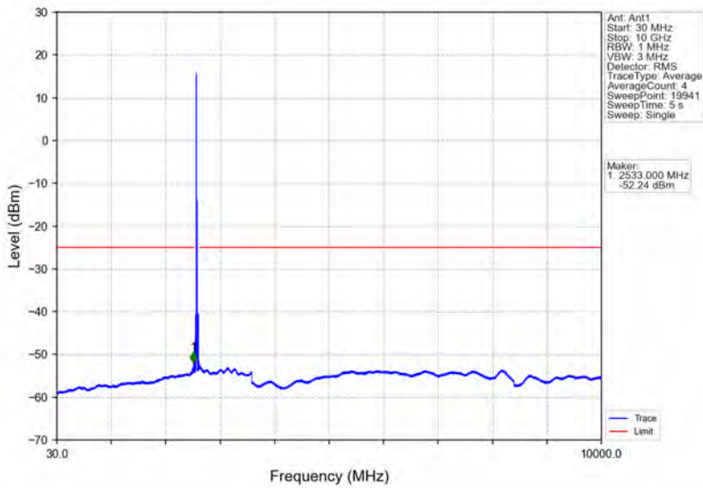
Band41_20MHz_QPSK_MCH_2593MHz_RB_1_0_NTNV
