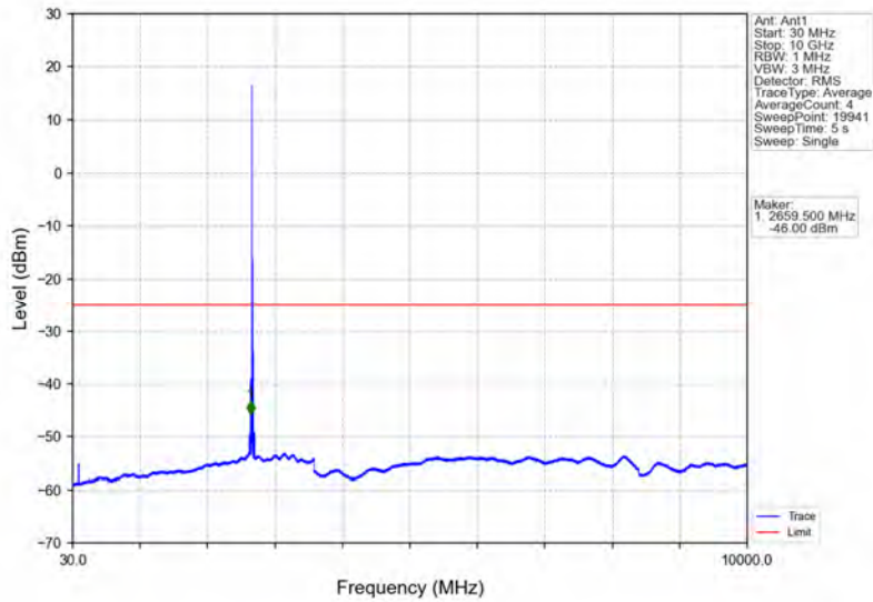
Band41_10MHz_QPSK_HCH_2685MHz_RB_1_0_NTNV
