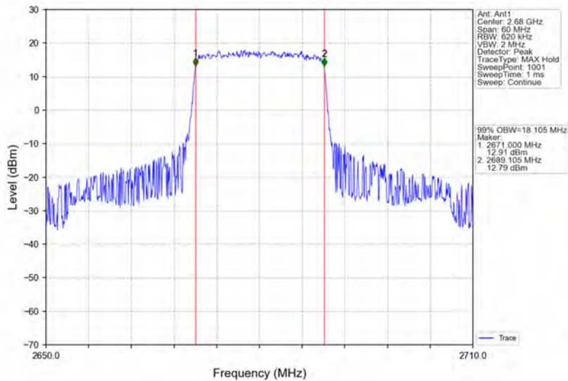
Band41_20MHz_QPSK_HCH_2680MHz_RB_100_0_NTNV
