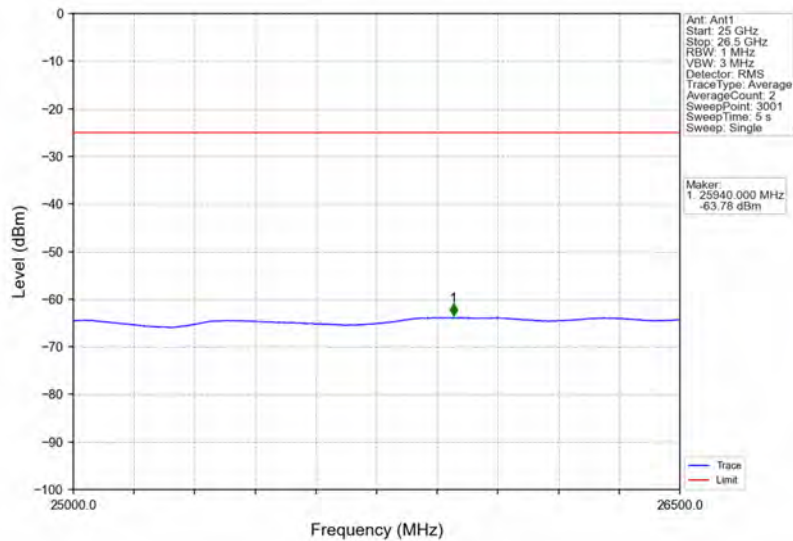
Band41_20MHz_QPSK_MCH_2593MHz_RB_1_0_NTNV
