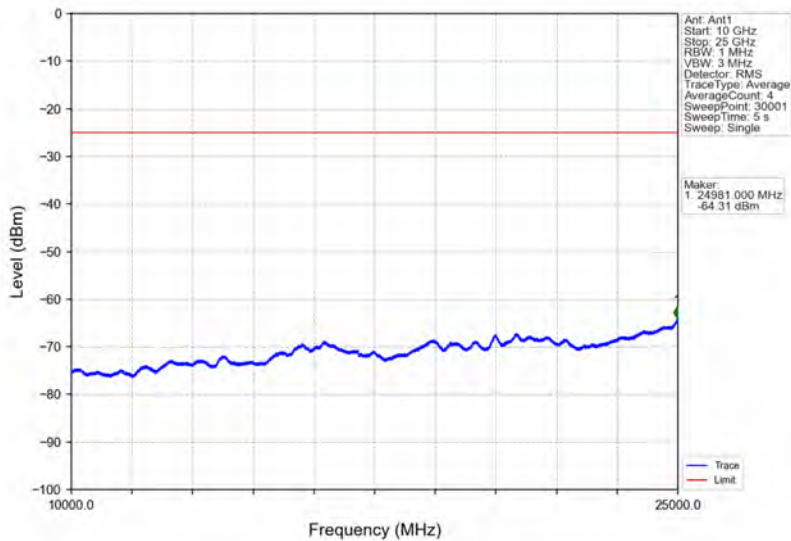
Band41_15MHz_QPSK_HCH_2682.5MHz_RB_1_0_NTNV
