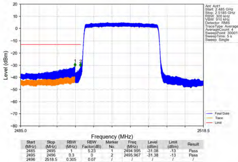
Band41_15MHz_QPSK_LCH_2503.5MHz_RB_75_0_NTNV
