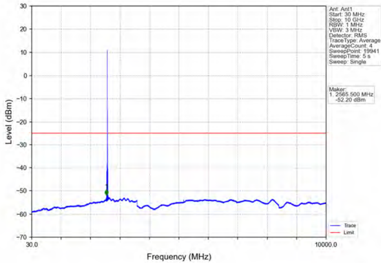
Band41_10MHz_16QAM_MCH_2593MHz_RB_1_0_NTNV
