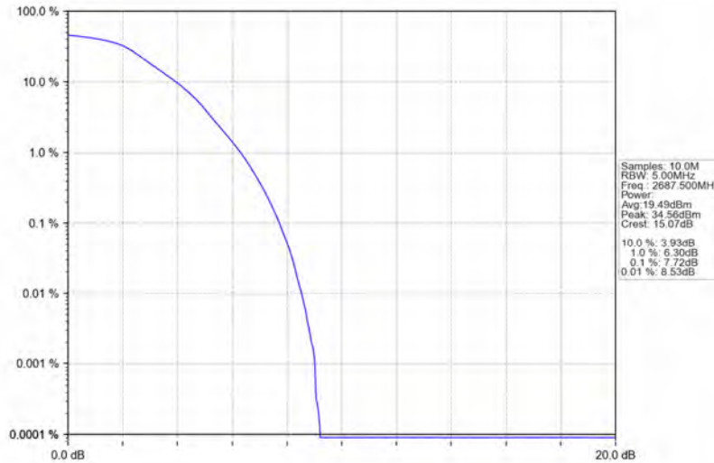
Band41_5MHz_QPSK_HCH_2687.5MHz_RB_25_0_NTNV
