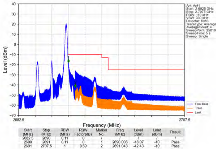
Band41_5MHz_QPSK_HCH_2687.5MHz_RB_1_24_NTNV
