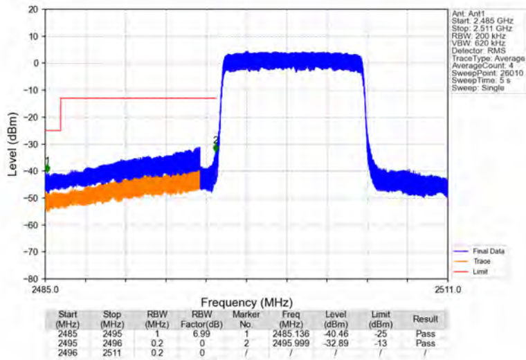
Band41_10MHz_16QAM_LCH_2501MHz_RB_50_0_NTNV
