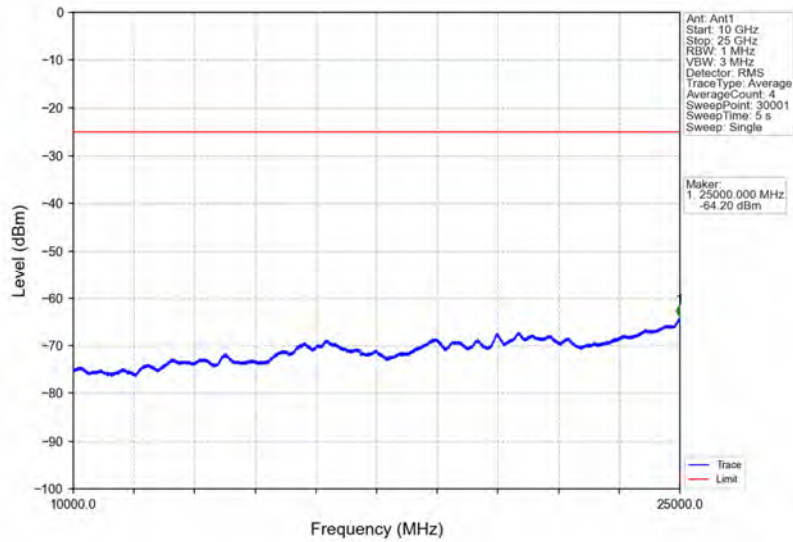
Band41_10MHz_QPSK_MCH_2593MHz_RB_1_0_NTNV
