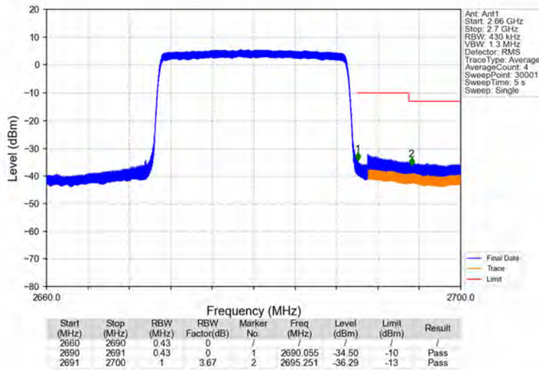
Band41_20MHz_QPSK_HCH_2680MHz_RB_100_0_NTNV
