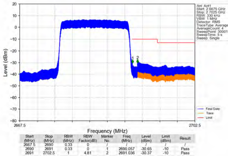
Band41_15MHz_QPSK_HCH_2682.5MHz_RB_75_0_NTNV
