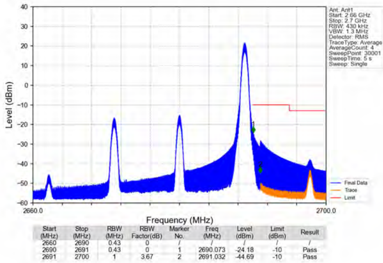
Band41_20MHz_QPSK_HCH_2680MHz_RB_1_99_NTNV
