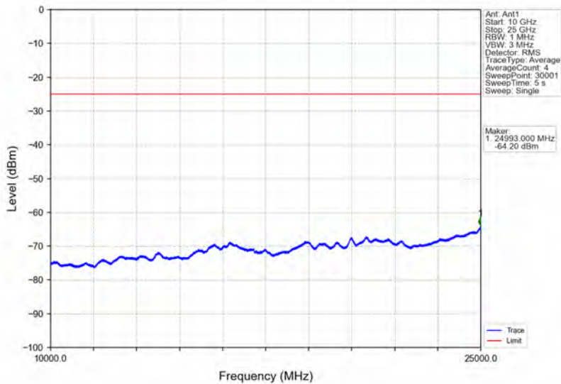
Band41_20MHz_16QAM_MCH_2593MHz_RB_1_0_NTNV
