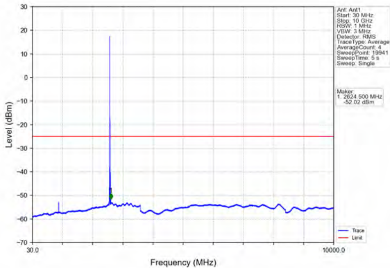
Band41_10MHz_QPSK_MCH_2593MHz_RB_1_0_NTNV
