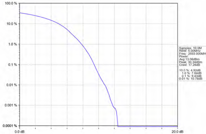
Band41_20MHz_16QAM_MCH_2593MHz_RB_100_0_NTNV
