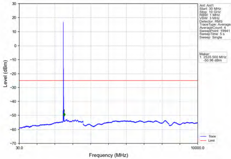
Band41_10MHz_16QAM_LCH_2501MHz_RB_1_0_NTNV
