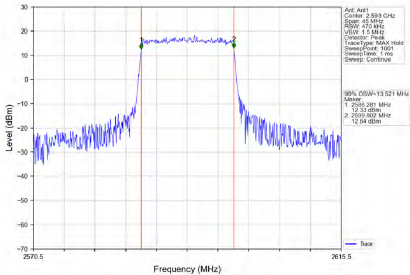
Band41_15MHz_QPSK_MCH_2593MHz_RB_75_0_NTNV
