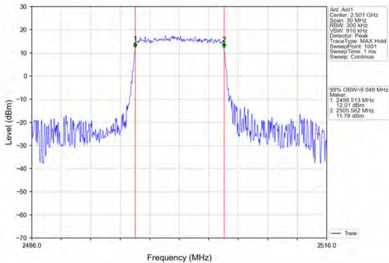
Band41_10MHz_QPSK_LCH_2501MHz_RB_50_0_NTNV
