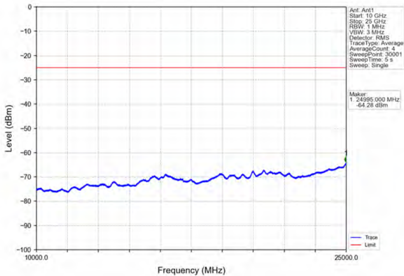
Band41_20MHz_QPSK_HCH_2680MHz_RB_1_0_NTNV
