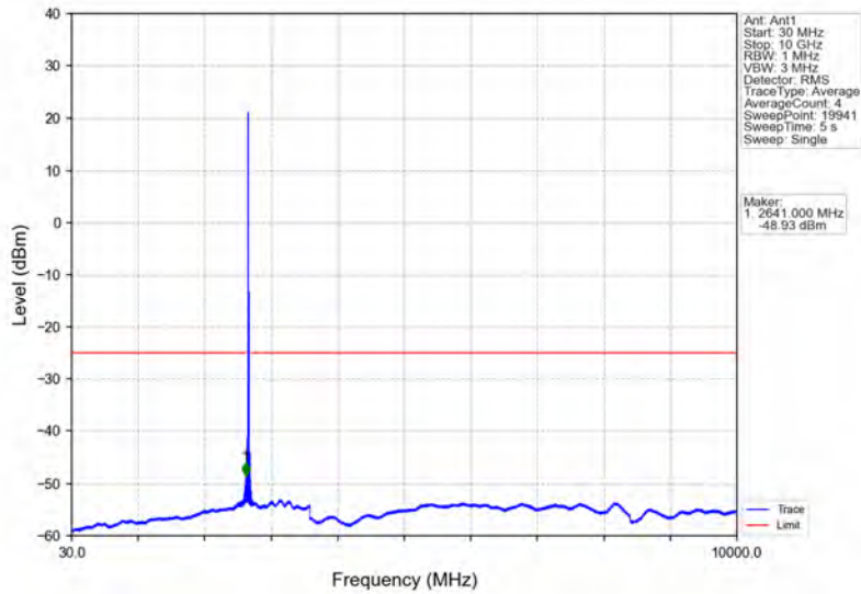
Band41_15MHz_QPSK_HCH_2682.5MHz_RB_1_0_NTNV
