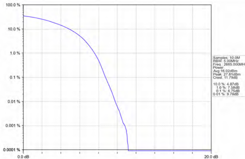
Band41_10MHz_16QAM_HCH_2685MHz_RB_50_0_NTNV
