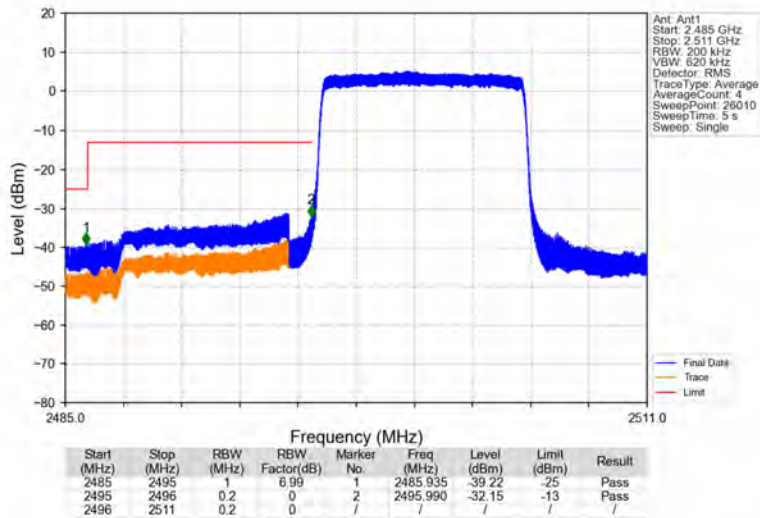
Band41_10MHz_QPSK_LCH_2501MHz_RB_50_0_NTNV
