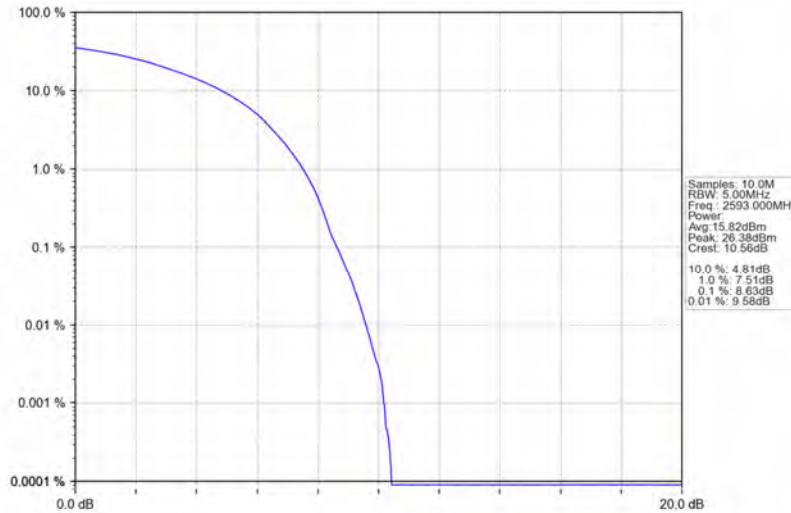
Band41_10MHz_16QAM_MCH_2593MHz_RB_50_0_NTNV
