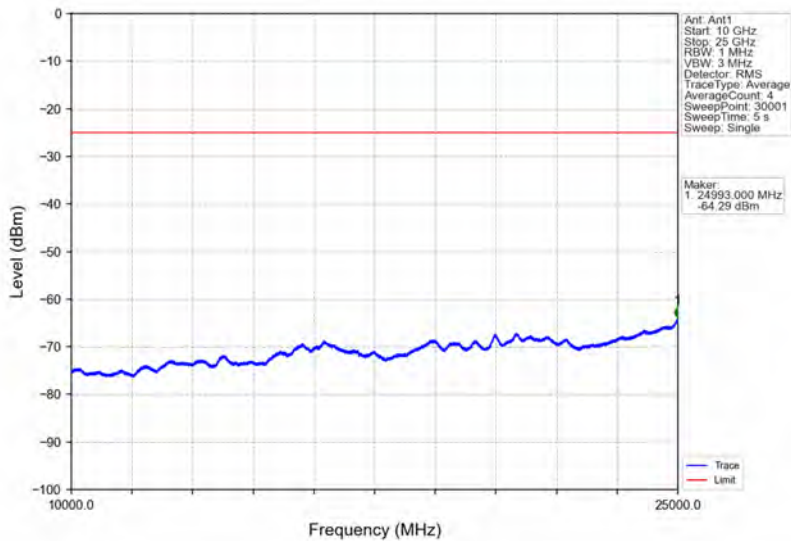
Band41_10MHz_16QAM_MCH_2593MHz_RB_1_0_NTNV
