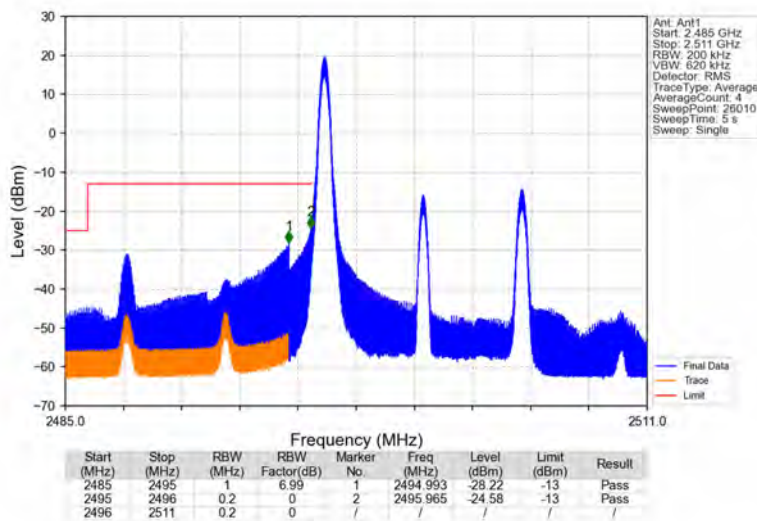
Band41_10MHz_16QAM_LCH_2501MHz_RB_1_0_NTNV
