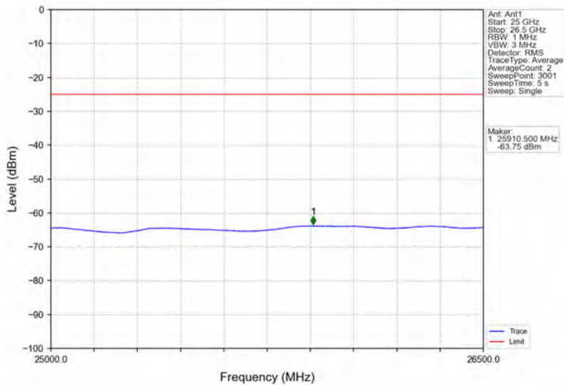
Band41_10MHz_16QAM_HCH_2685MHz_RB_1_0_NTNV
