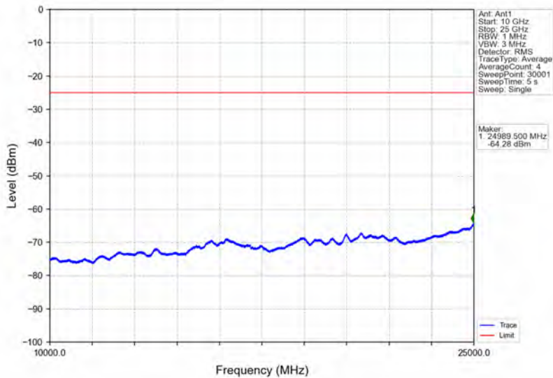
Band41_10MHz_16QAM_LCH_2501MHz_RB_1_0_NTNV
