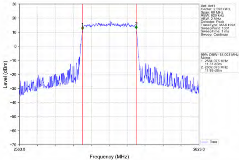
Band41_20MHz_16QAM_MCH_2593MHz_RB_100_0_NTNV
