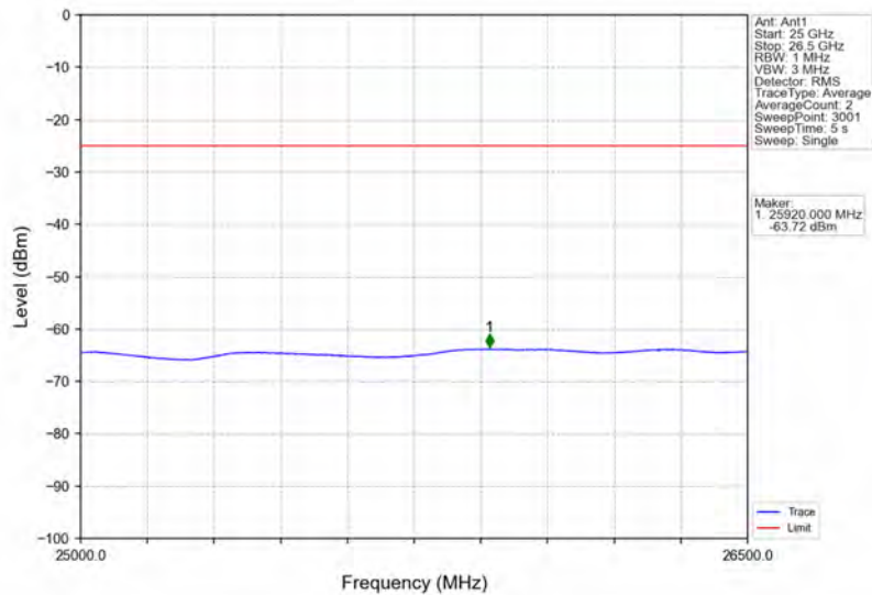
Band41_5MHz_QPSK_MCH_2593MHz_RB_1_0_NTNV
