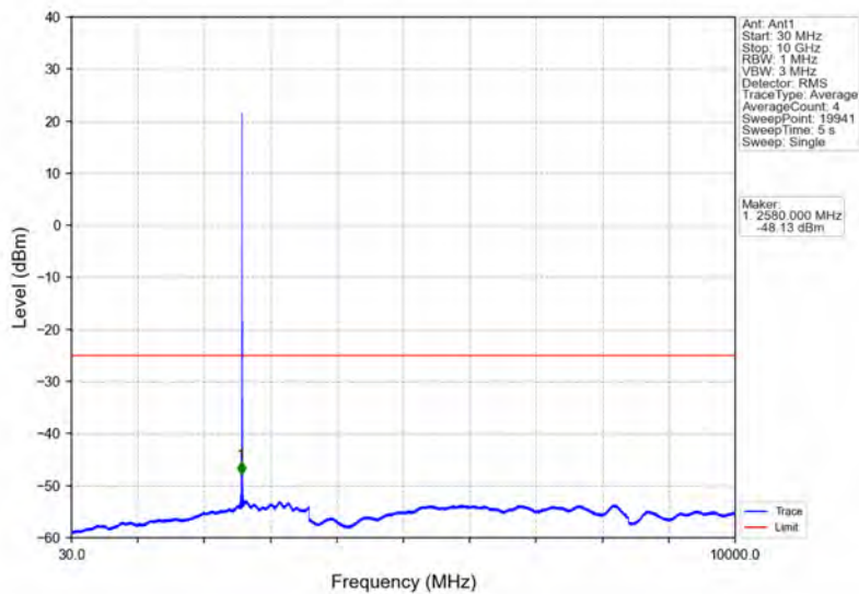
Band41_5MHz_QPSK_MCH_2593MHz_RB_1_0_NTNV
