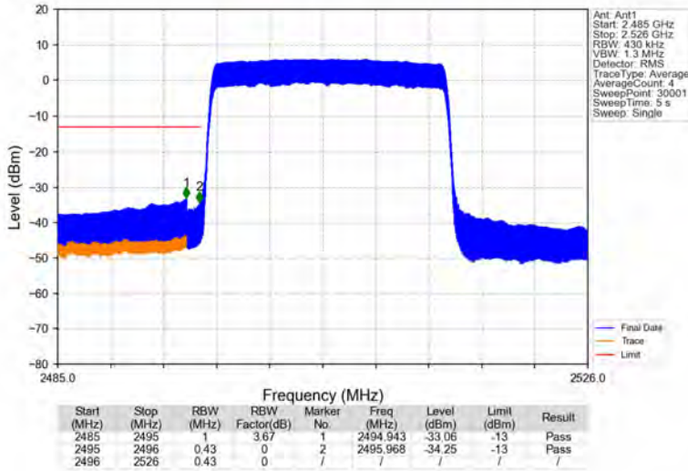
Band41_20MHz_QPSK_LCH_2506MHz_RB_100_0_NTNV
