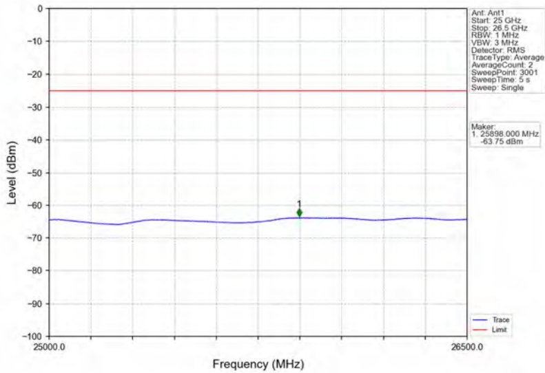
Band41_10MHz_16QAM_LCH_2501MHz_RB_50_0_NTNV
