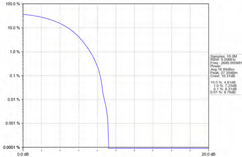
Band41_10MHz_QPSK_HCH_2685MHz_RB_50_0_NTNV
