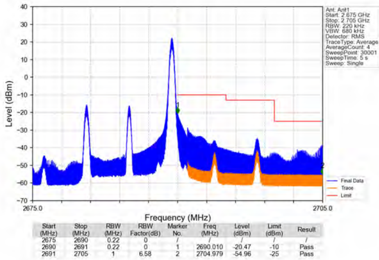
Band41_10MHz_QPSK_HCH_2685MHz_RB_1_49_NTNV
