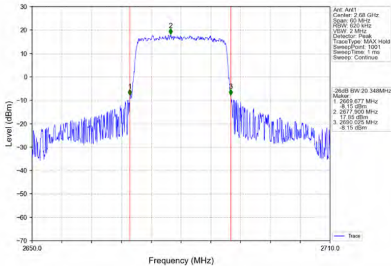
Band41_20MHz_QPSK_HCH_2680MHz_RB_100_0_NTNV
