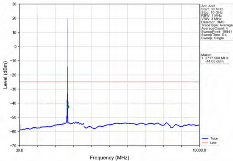
Band41_10MHz_16QAM_HCH_2685MHz_RB_1_0_NTNV
