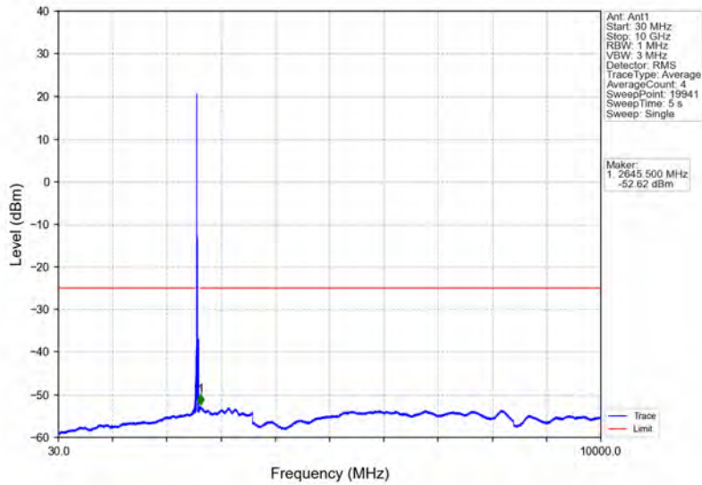
Band38_20MHz_16QAM_LCH_2580MHz_RB_1_0_NTNV
