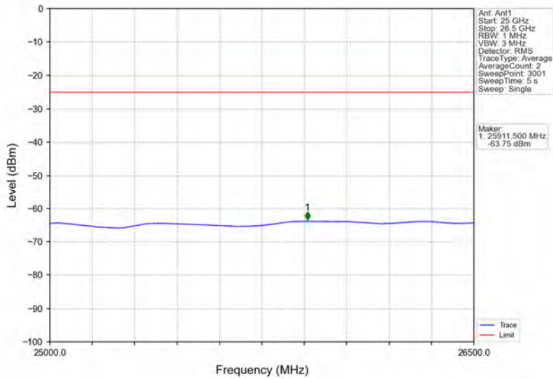
Band38_20MHz_QPSK_HCH_2610MHz_RB_1_99_NTNV
