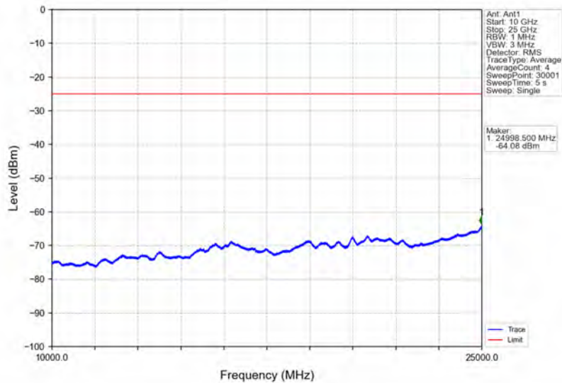
Band38_20MHz_16QAM_MCH_2595MHz_RB_1_0_NTNV
