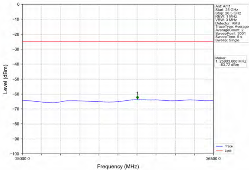
Band38_20MHz_QPSK_LCH_2580MHz_RB_1_0_NTNV
