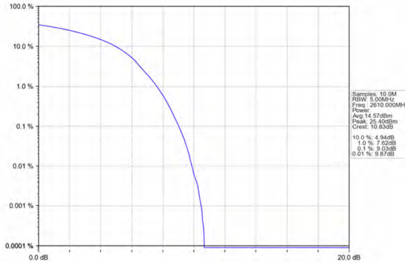
Band38_20MHz_QPSK_HCH_2610MHz_RB_100_0_NTNV
