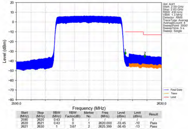
Band38_20MHz_QPSK_HCH_2610MHz_RB_100_0_NTNV
