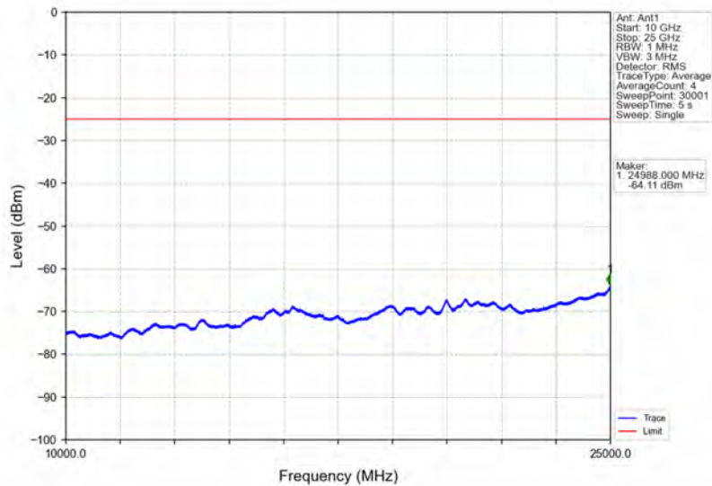
Band38_10MHz_QPSK_HCH_2615MHz_RB_1_0_NTNV
