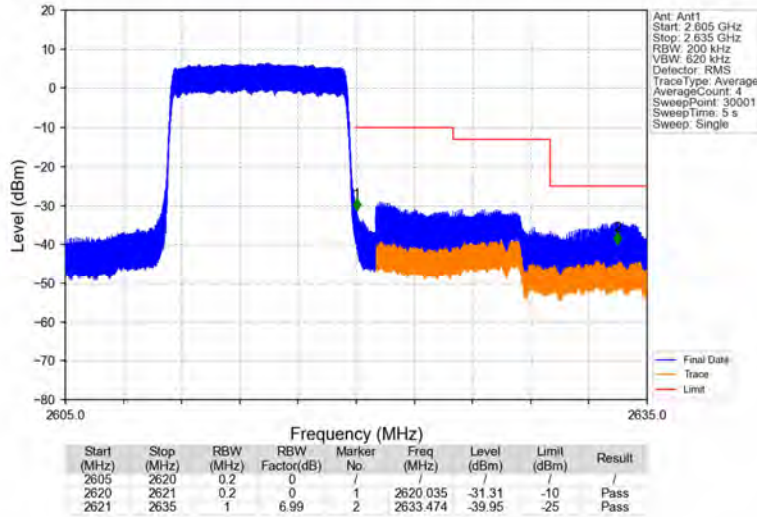
Band38_10MHz_QPSK_HCH_2615MHz_RB_50_0_NTNV
