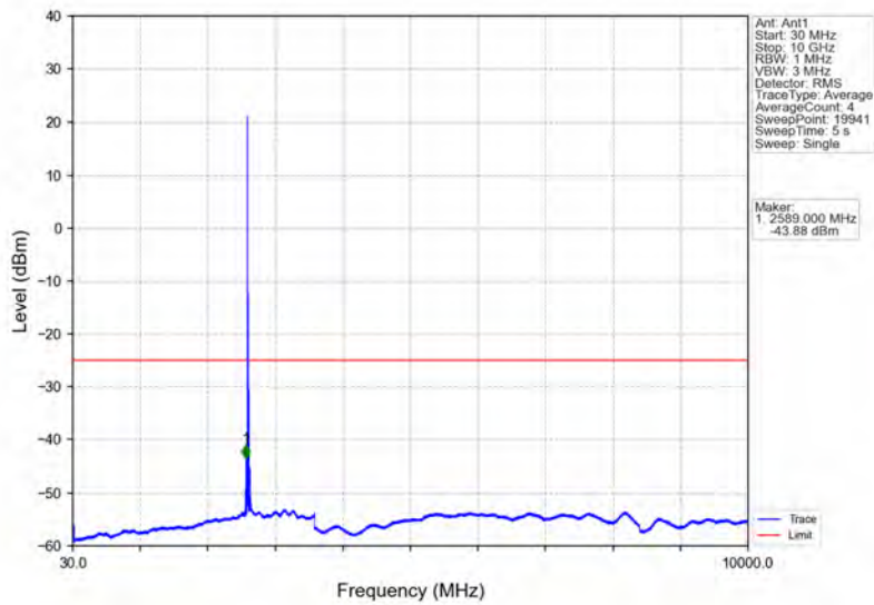
Band38_10MHz_QPSK_HCH_2615MHz_RB_1_0_NTNV
