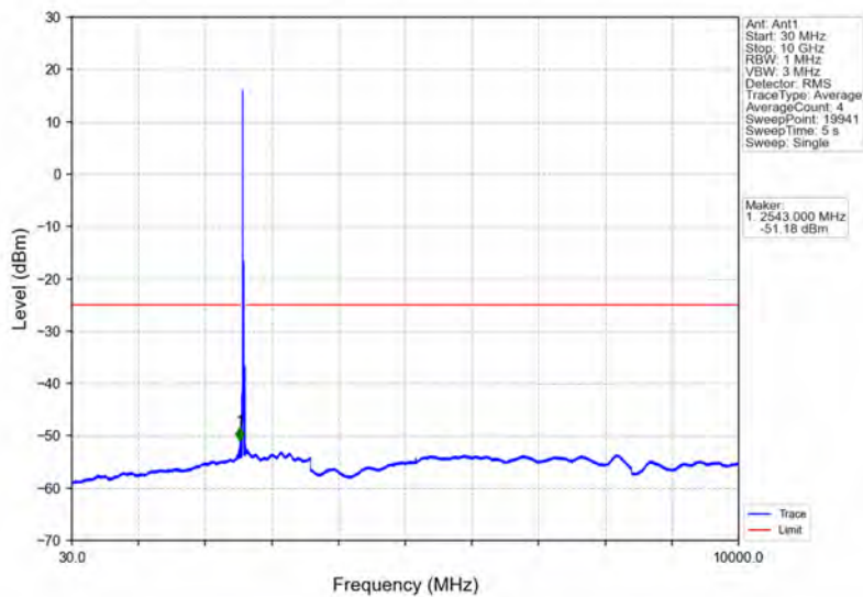
Band38_20MHz_QPSK_MCH_2595MHz_RB_1_0_NTNV
