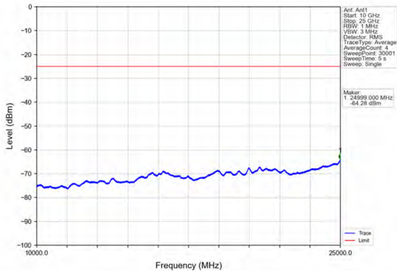
Band38_20MHz_16QAM_LCH_2580MHz_RB_1_0_NTNV
