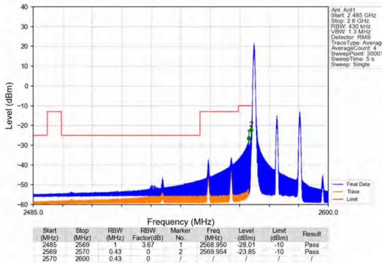
Band38_20MHz_16QAM_LCH_2580MHz_RB_1_0_NTNV
