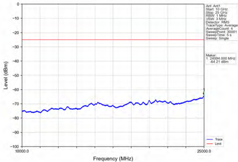
Band38_20MHz_QPSK_HCH_2610MHz_RB_1_0_NTNV
