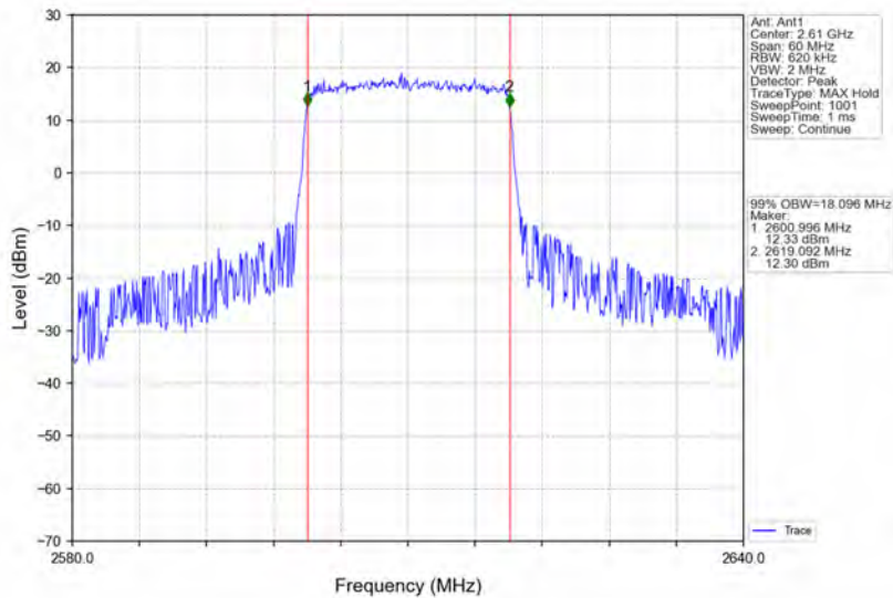
Band38_20MHz_QPSK_HCH_2610MHz_RB_100_0_NTNV
