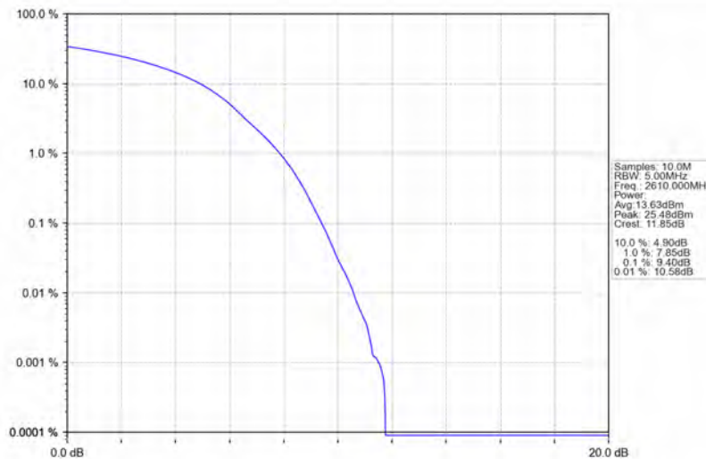
Band38_20MHz_16QAM_HCH_2610MHz_RB_100_0_NTNV
