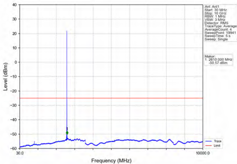
Band38_5MHz_QPSK_MCH_2595MHz_RB_1_0_NTNV
