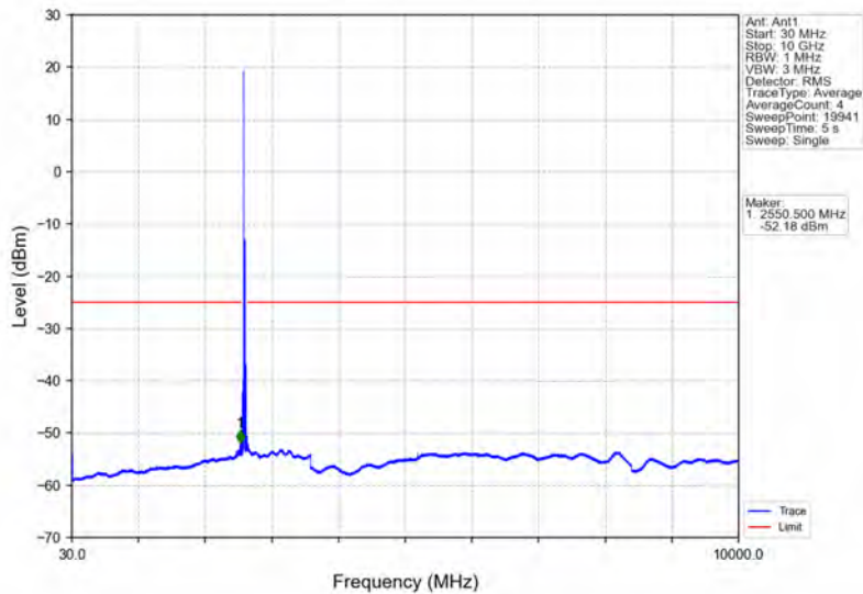
Band38_20MHz_16QAM_HCH_2610MHz_RB_1_0_NTNV
