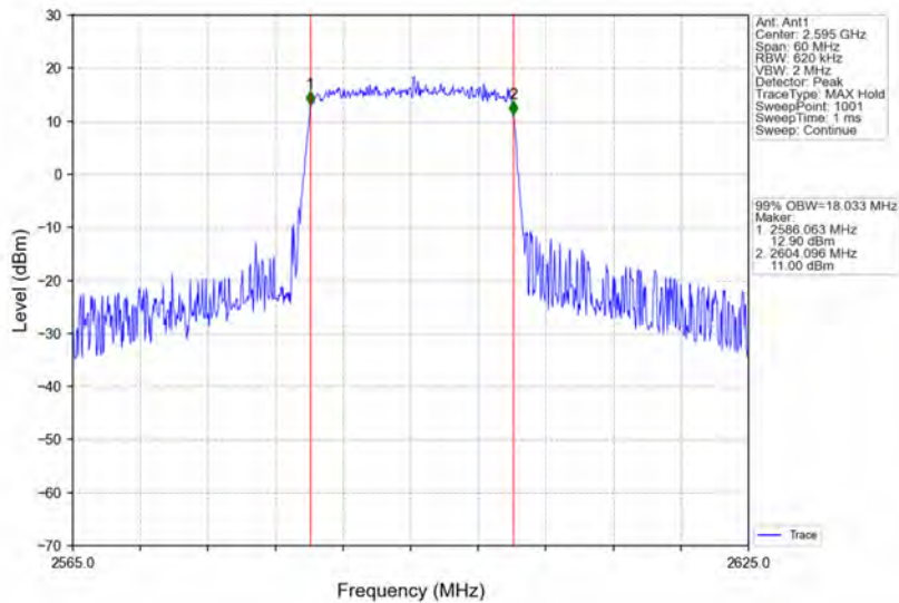
Band38_20MHz_16QAM_MCH_2595MHz_RB_100_0_NTNV
