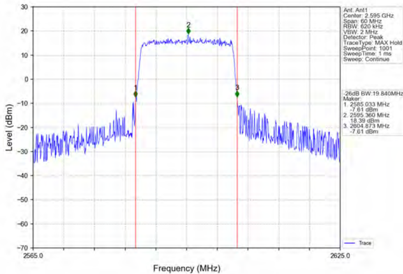
Band38_20MHz_16QAM_MCH_2595MHz_RB_100_0_NTNV
