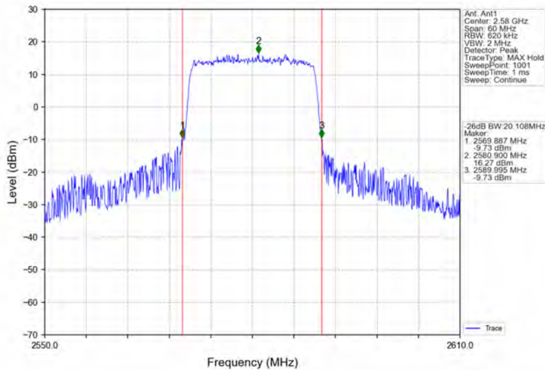
Band38_20MHz_64QAM_LCH_2580MHz_RB_100_0_NTNV
