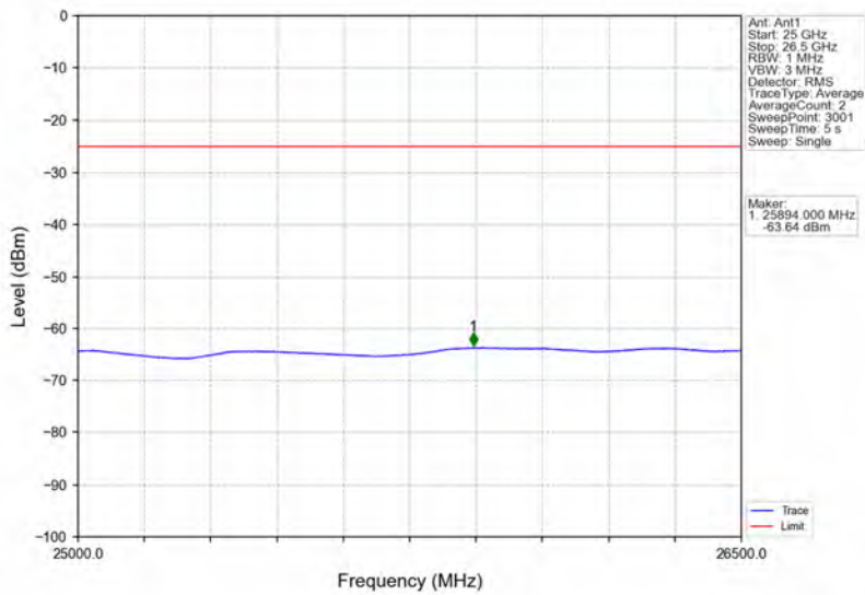
Band38_10MHz_QPSK_HCH_2615MHz_RB_1_49_NTNV
