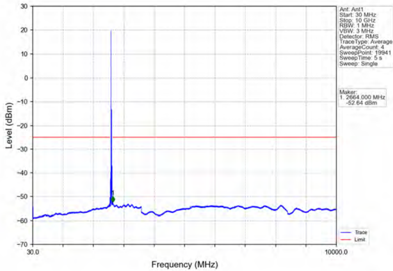
Band38_20MHz_QPSK_HCH_2610MHz_RB_1_0_NTNV
