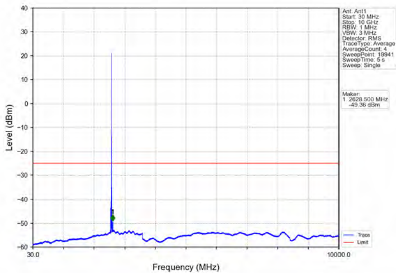
Band38_10MHz_QPSK_MCH_2595MHz_RB_1_0_NTNV
