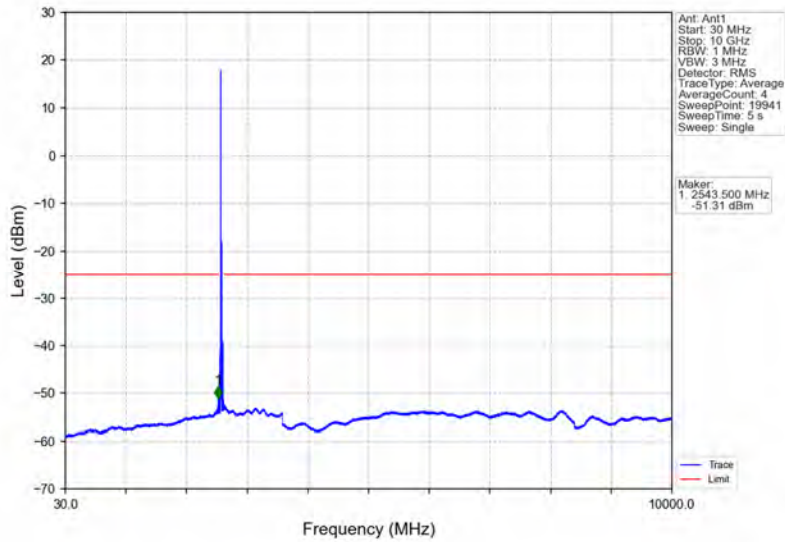
Band38_20MHz_16QAM_MCH_2595MHz_RB_1_0_NTNV
