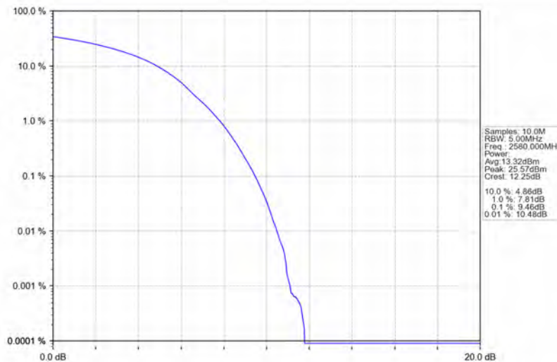
Band38_20MHz_16QAM_LCH_2580MHz_RB_100_0_NTNV
