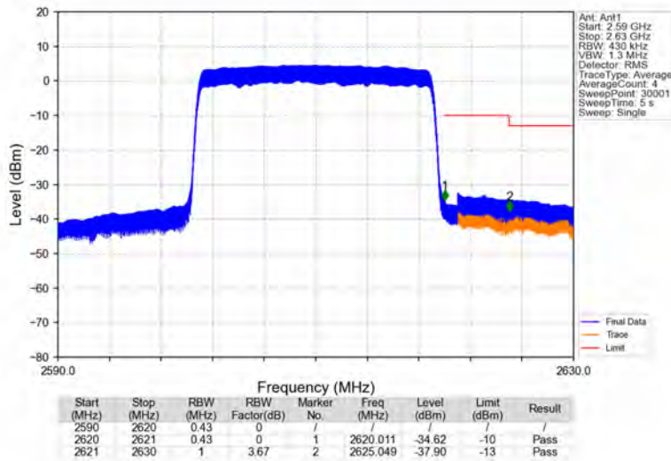
Band38_20MHz_16QAM_HCH_2610MHz_RB_100_0_NTNV
