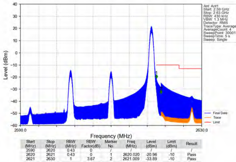
Band38_20MHz_16QAM_HCH_2610MHz_RB_1_99_NTNV
