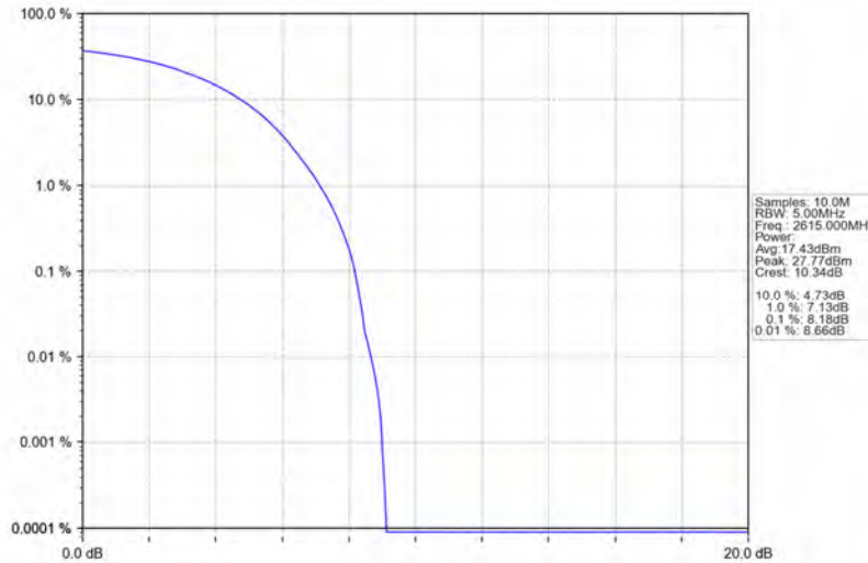
Band38_10MHz_QPSK_HCH_2615MHz_RB_50_0_NTNV
