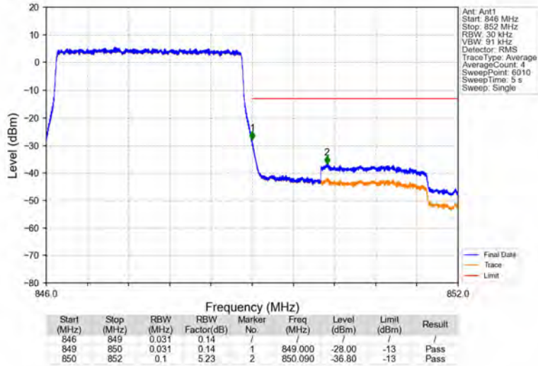
Band26b_3MHz_QPSK_HCH_847.5MHz_RB_15_0_NTNV
