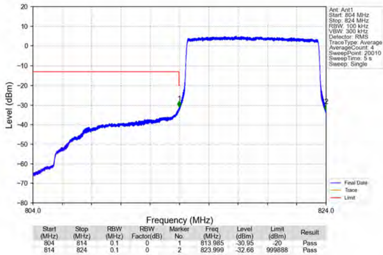
Band26a_10MHz_QPSK_LCH_819MHz_RB_50_0_NTNV
