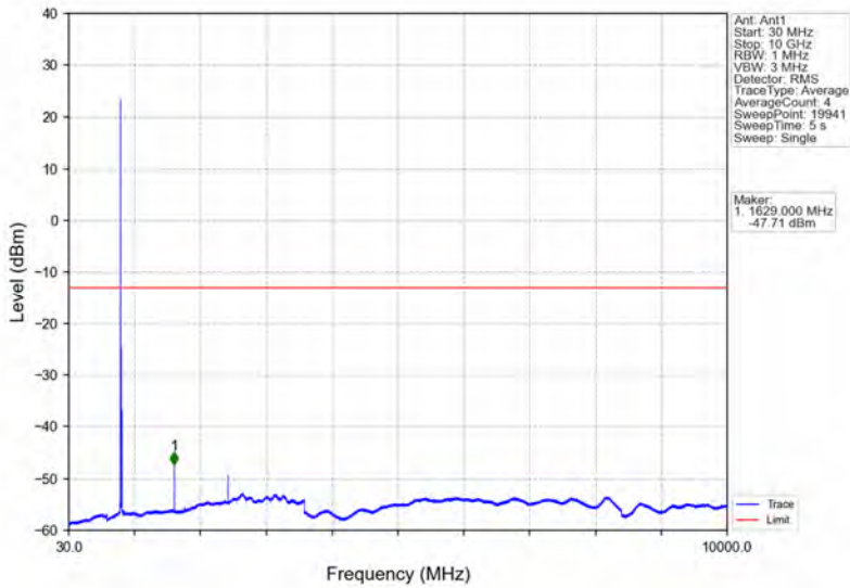
Band26a_10MHz_QPSK_HCH_819MHz_RB_1_49_NTNV
