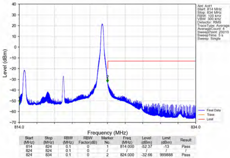
Band26a_10MHz_QPSK_HCH_819MHz_RB_1_49_NTNV
