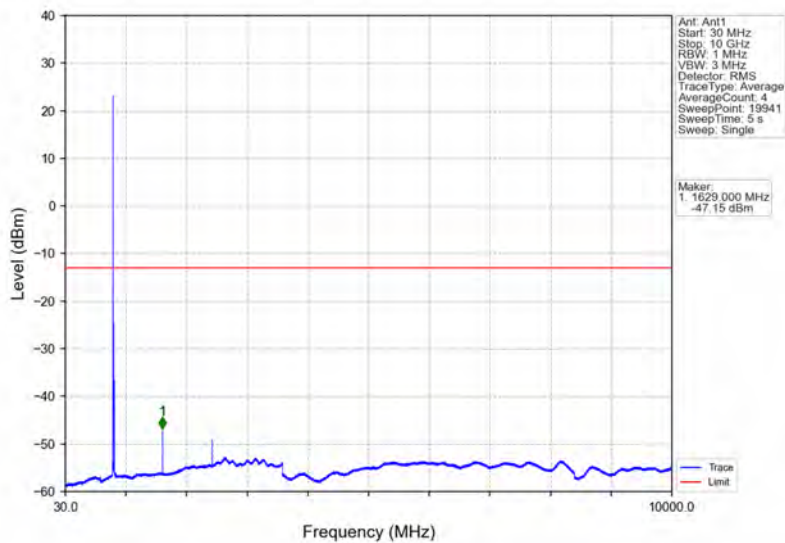
Band26a_10MHz_QPSK_MCH_819MHz_RB_1_0_NTNV
