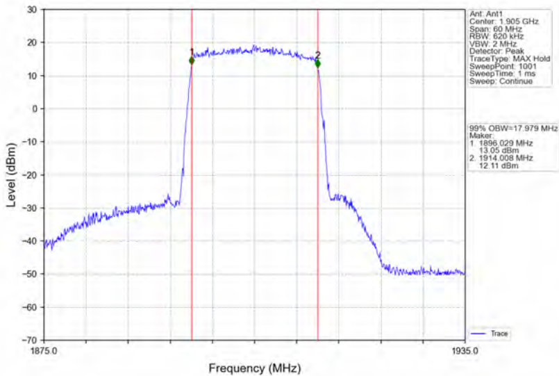
Band25_20MHz_QPSK_HCH_1905MHz_RB_100_0_NTNV
