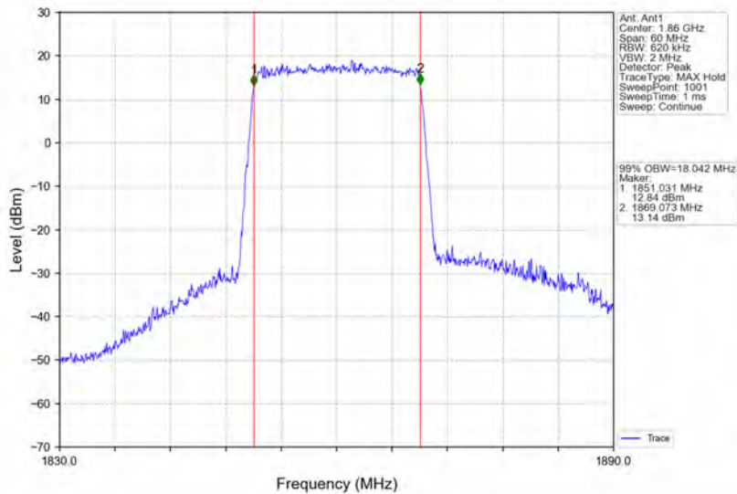
Band25_20MHz_QPSK_LCH_1860MHz_RB_100_0_NTNV
