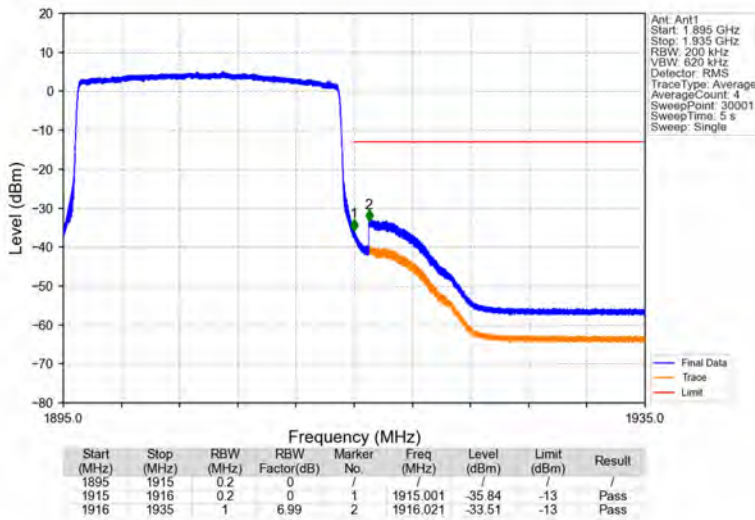
Band25_20MHz_QPSK_HCH_1905MHz_RB_100_0_NTNV
