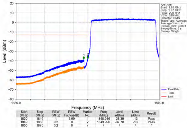
Band25_20MHz_QPSK_LCH_1860MHz_RB_100_0_NTNV
