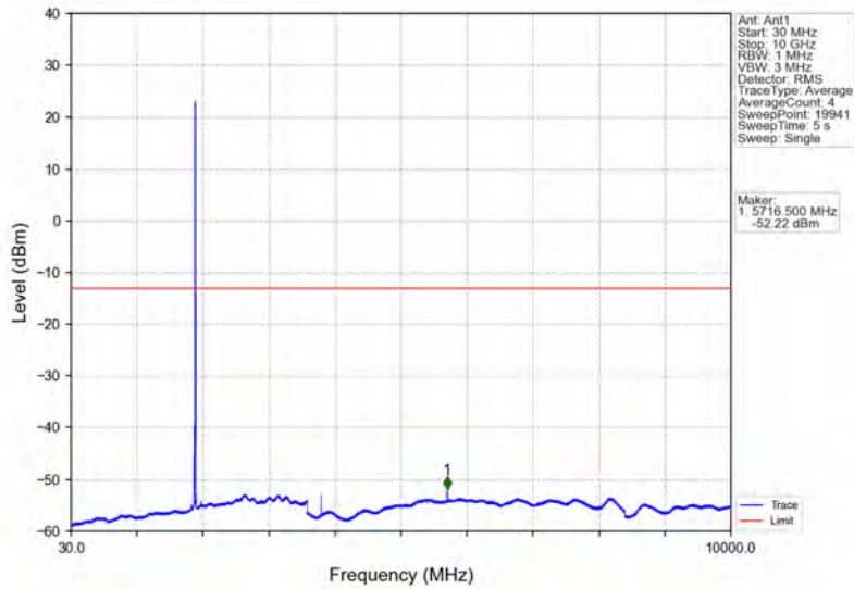
Band25_10MHz_QPSK_HCH_1910MHz_RB_1_0_NTNV
