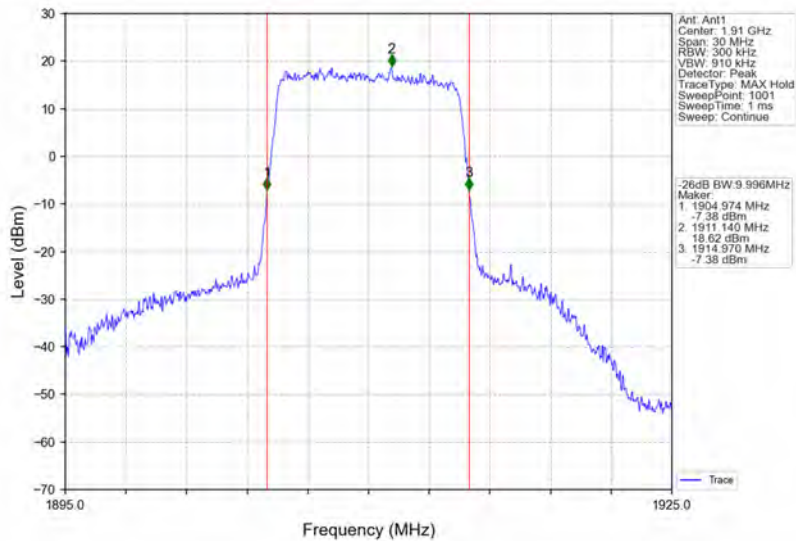
Band25_10MHz_QPSK_HCH_1910MHz_RB_50_0_NTNV
