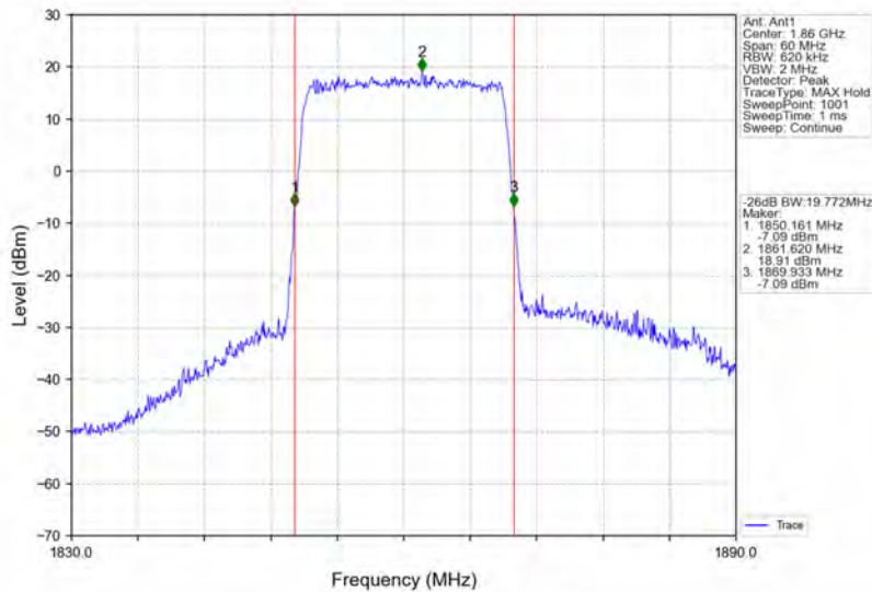
Band25_20MHz_QPSK_LCH_1860MHz_RB_100_0_NTNV
