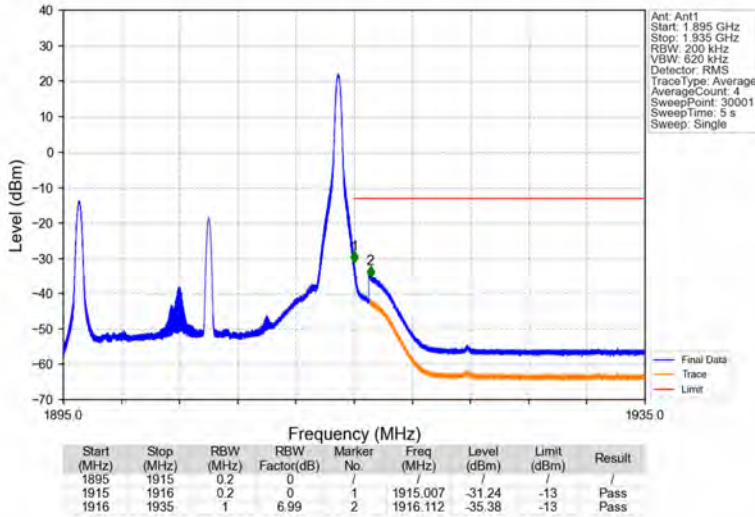
Band25_20MHz_QPSK_HCH_1905MHz_RB_1_99_NTNV
