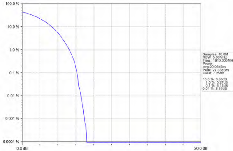
Band25_10MHz_QPSK_HCH_1910MHz_RB_50_0_NTNV
