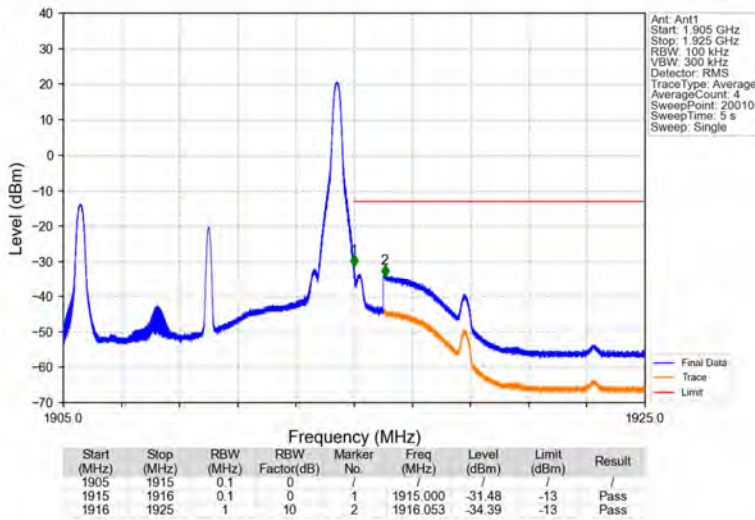
Band25_10MHz_QPSK_HCH_1910MHz_RB_1_49_NTNV
