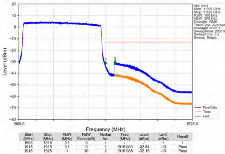
Band25_10MHz_QPSK_HCH_1910MHz_RB_50_0_NTNV
