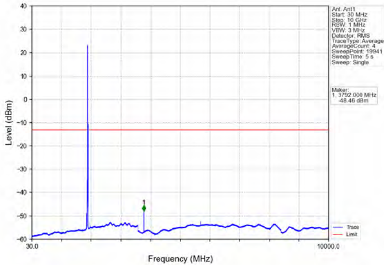
Band25_20MHz_QPSK_HCH_1905MHz_RB_1_0_NTNV
