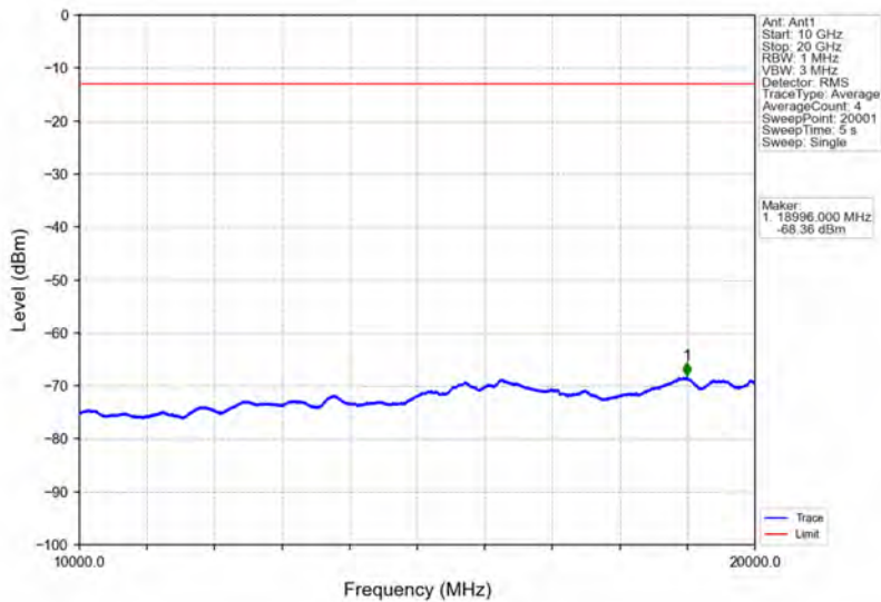
Band25_10MHz_QPSK_HCH_1910MHz_RB_1_0_NTNV
