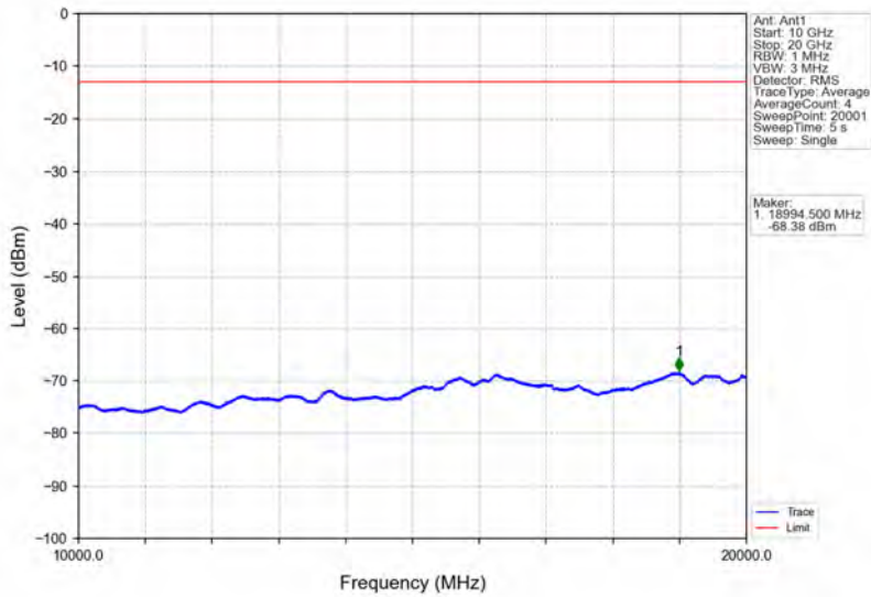
Band25_20MHz_QPSK_LCH_1860MHz_RB_100_0_NTNV
