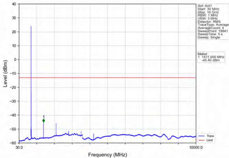
Band17_10MHz_QPSK_MCH_710MHz_RB_1_0_NTNV
