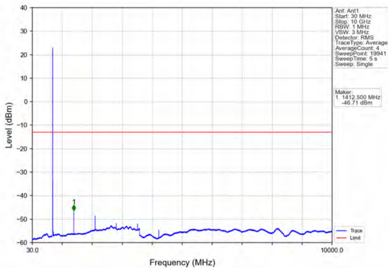
Band12_3MHz_QPSK_MCH_707.5MHz_RB_1_0_NTNV
