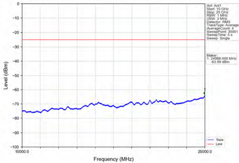
Band7_10MHz_QPSK_LCH_2505MHz_RB_1_0_NTNV
