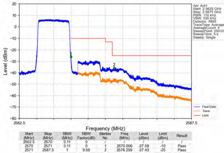
Band7_5MHz_QPSK_HCH_2567.5MHz_RB_25_0_NTNV
