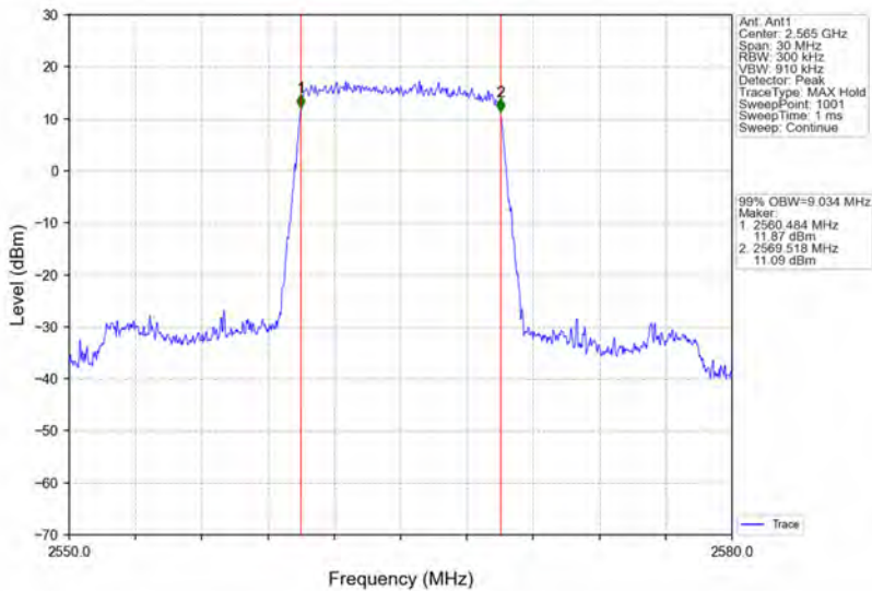
Band7_10MHz_QPSK_HCH_2565MHz_RB_50_0_NTNV
