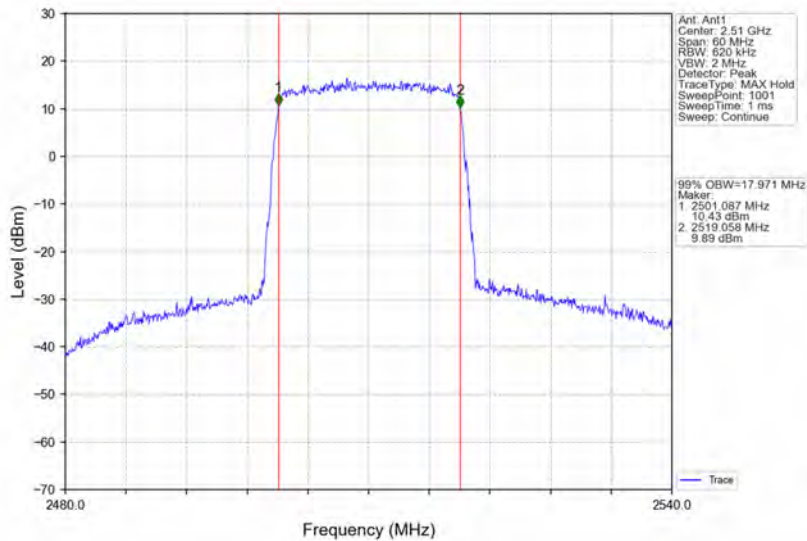
Band7_20MHz_64QAM_LCH_2510MHz_RB_100_0_NTNV
