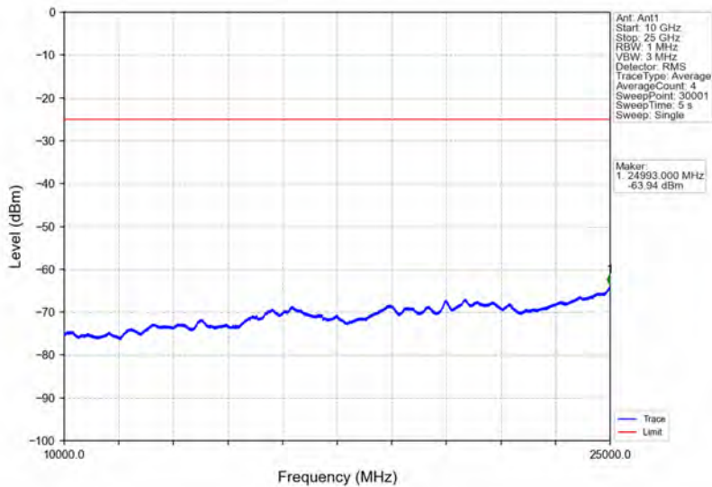
Band7_10MHz_QPSK_HCH_2565MHz_RB_1_0_NTNV
