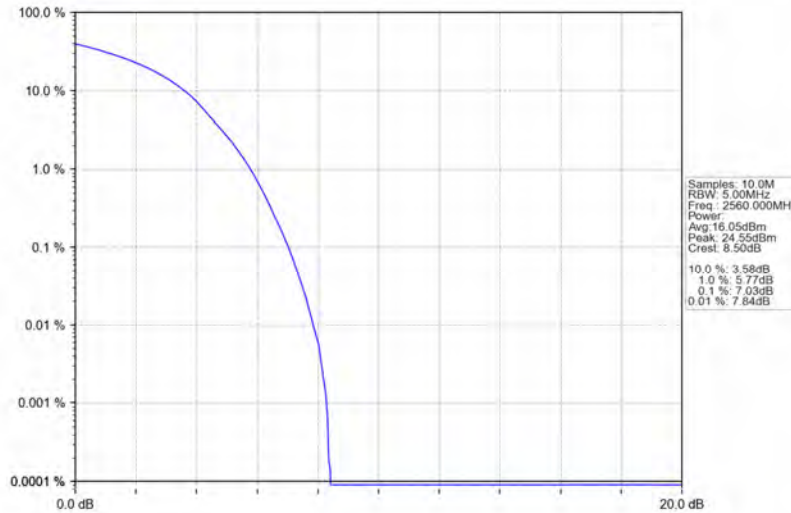
Band7_20MHz_QPSK_HCH_2560MHz_RB_100_0_NTNV
