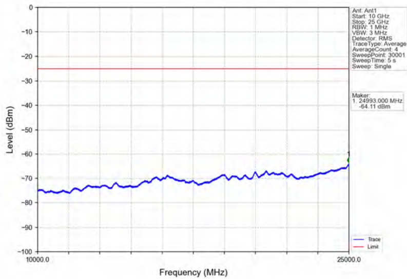
Band7_20MHz_16QAM_HCH_2560MHz_RB_1_0_NTNV
