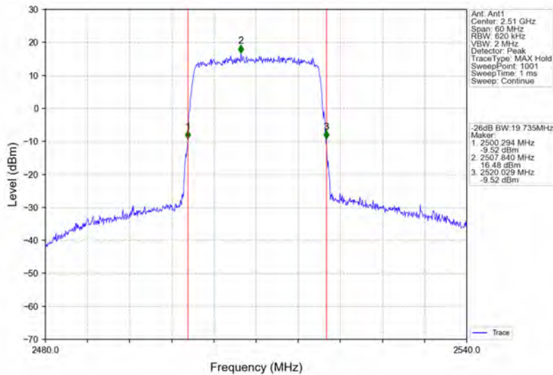
Band7_20MHz_64QAM_LCH_2510MHz_RB_100_0_NTNV
