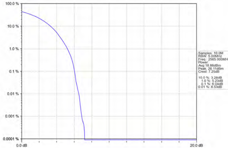
Band7_10MHz_QPSK_HCH_2565MHz_RB_50_0_NTNV
