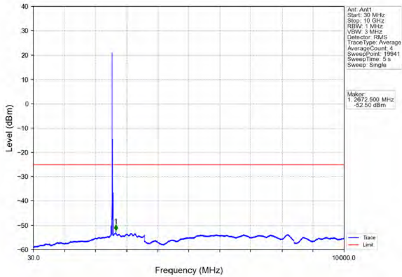
Band7_20MHz_QPSK_HCH_2560MHz_RB_1_0_NTNV
