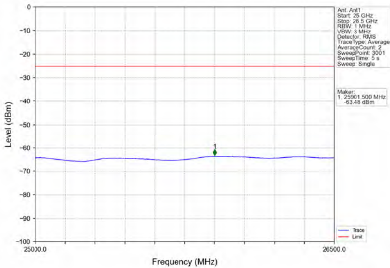
Band7_20MHz_QPSK_HCH_2560MHz_RB_1_99_NTNV
