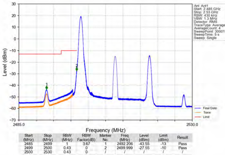
Band7_20MHz_64QAM_LCH_2510MHz_RB_1_0_NTNV
