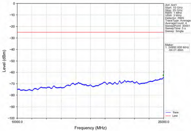
Band7_20MHz_QPSK_MCH_2535MHz_RB_1_0_NTNV
