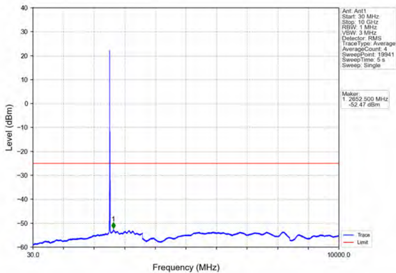
Band7_10MHz_QPSK_MCH_2535MHz_RB_1_0_NTNV
