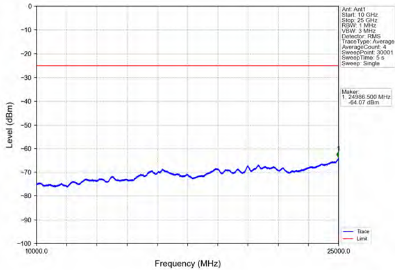
Band7_20MHz_64QAM_MCH_2535MHz_RB_1_0_NTNV
