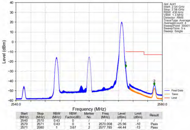
Band7_20MHz_16QAM_HCH_2560MHz_RB_1_99_NTNV
