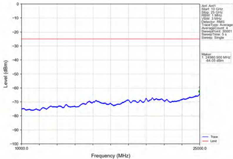
Band7_20MHz_16QAM_LCH_2510MHz_RB_1_0_NTNV
