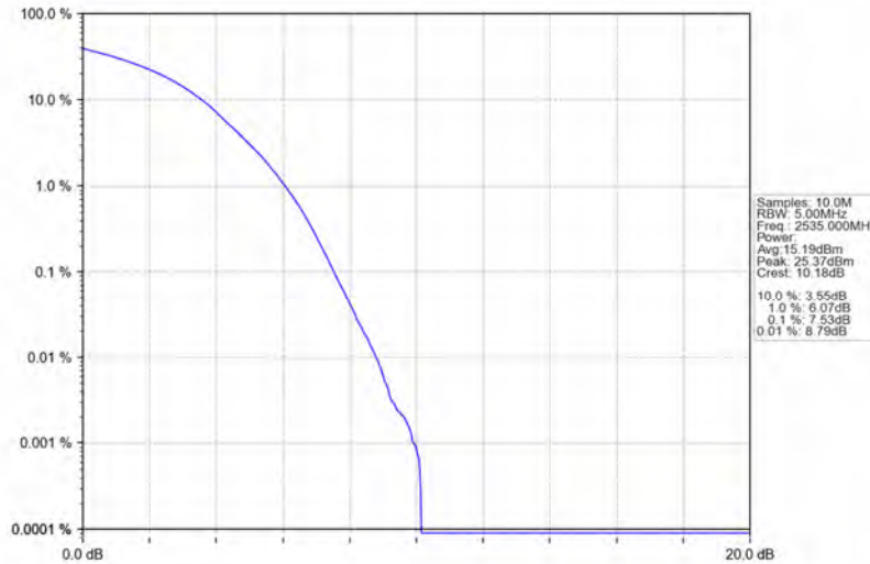
Band7_20MHz_16QAM_MCH_2535MHz_RB_100_0_NTNV
