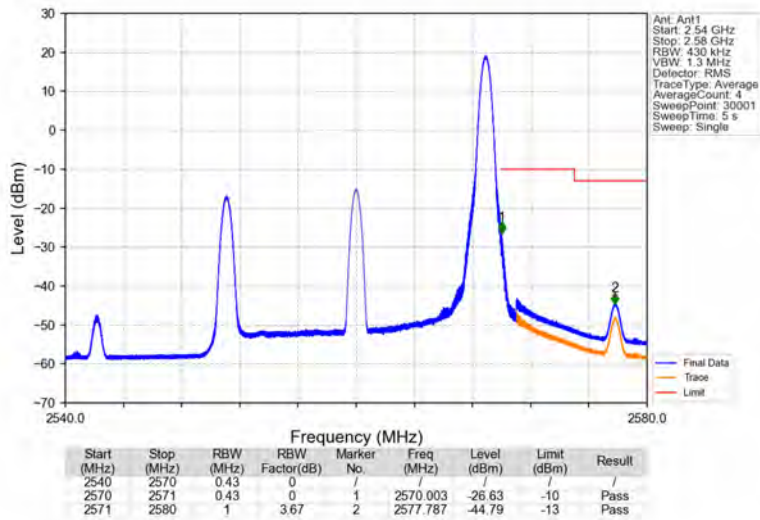
Band7_20MHz_64QAM_HCH_2560MHz_RB_1_99_NTNV
