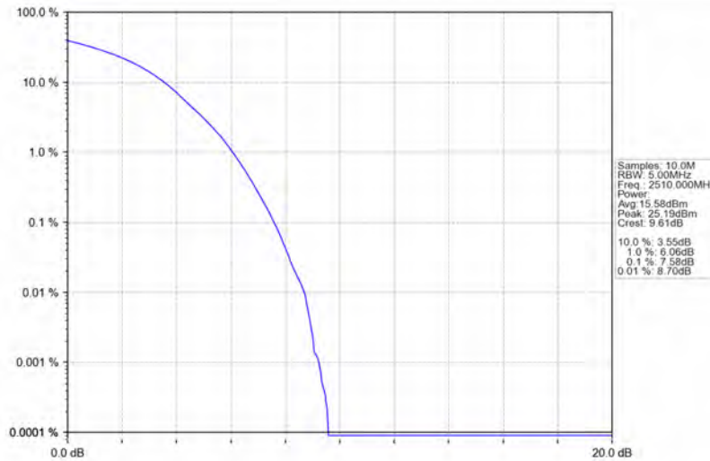
Band7_20MHz_16QAM_LCH_2510MHz_RB_100_0_NTNV
