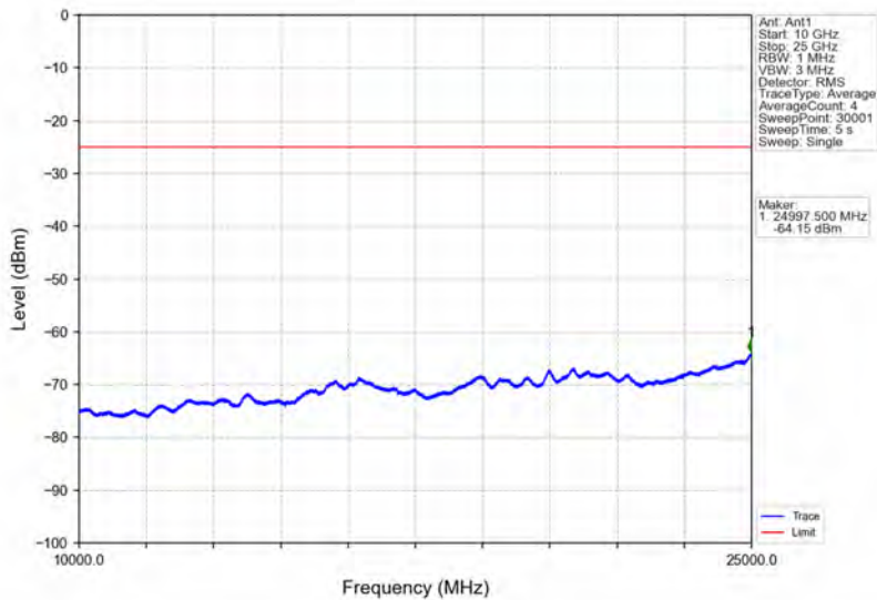
Band7_5MHz_QPSK_HCH_2567.5MHz_RB_1_0_NTNV
