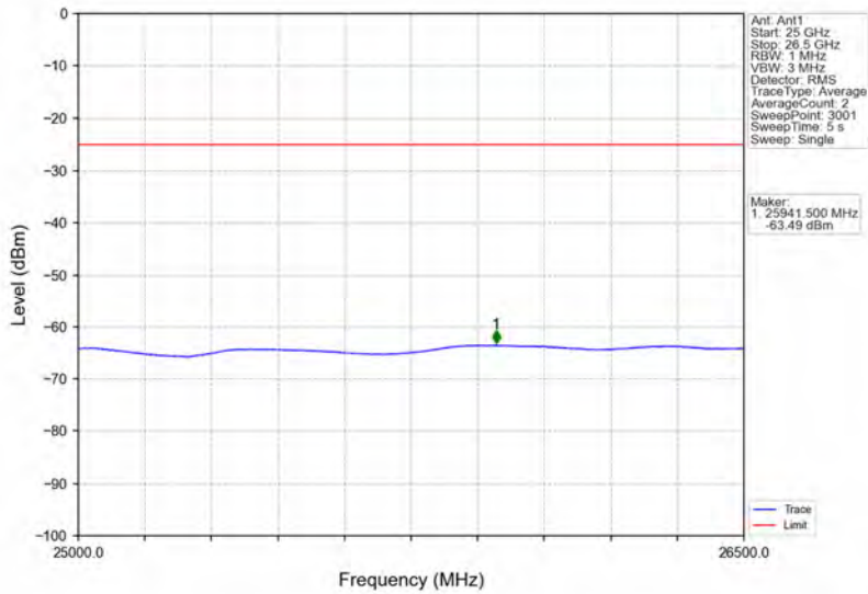
Band7_5MHz_QPSK_HCH_2567.5MHz_RB_1_24_NTNV
