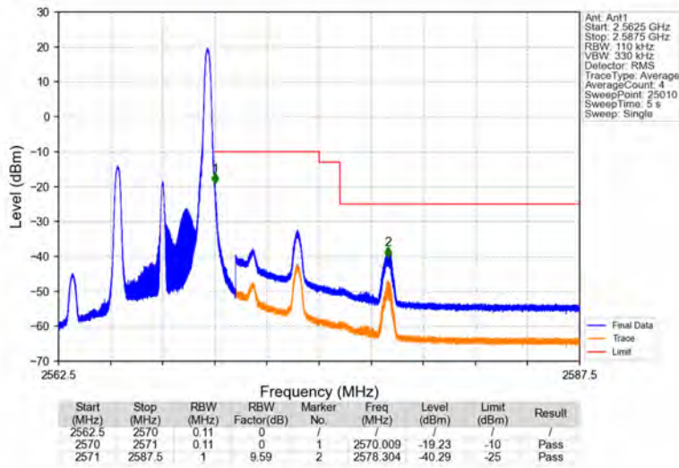
Band7_5MHz_QPSK_HCH_2567.5MHz_RB_1_24_NTNV
