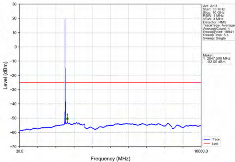
Band7_20MHz_64QAM_MCH_2535MHz_RB_1_0_NTNV
