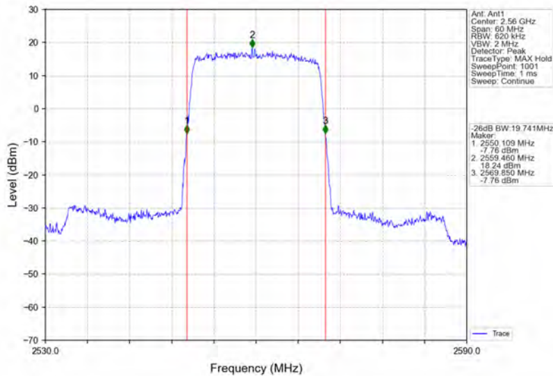
Band7_20MHz_QPSK_HCH_2560MHz_RB_100_0_NTNV
