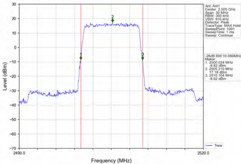
Band7_10MHz_QPSK_LCH_2505MHz_RB_50_0_NTNV
