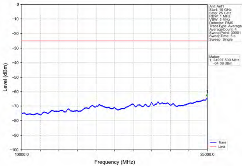
Band7_20MHz_64QAM_LCH_2510MHz_RB_1_0_NTNV
