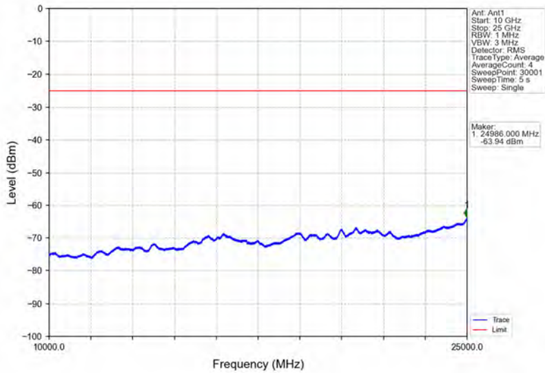
Band7_10MHz_QPSK_MCH_2535MHz_RB_1_0_NTNV
