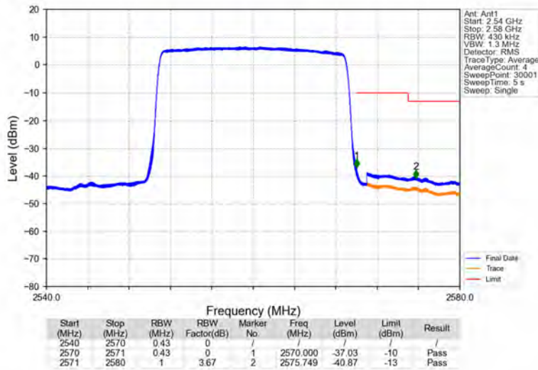
Band7_20MHz_QPSK_HCH_2560MHz_RB_100_0_NTNV
