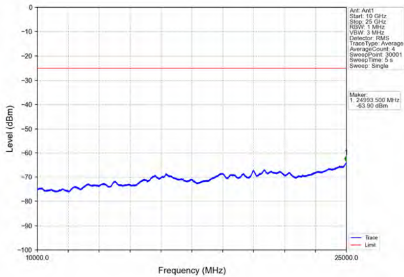
Band7_5MHz_QPSK_MCH_2535MHz_RB_1_0_NTNV
