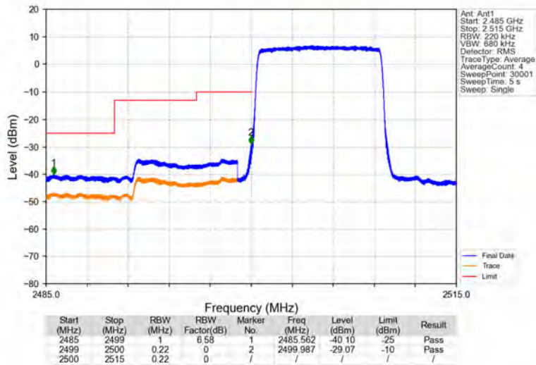
Band7_10MHz_QPSK_LCH_2505MHz_RB_50_0_NTNV
