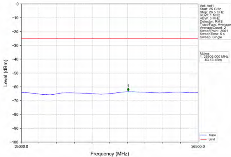
Band7_20MHz_64QAM_MCH_2535MHz_RB_1_0_NTNV
