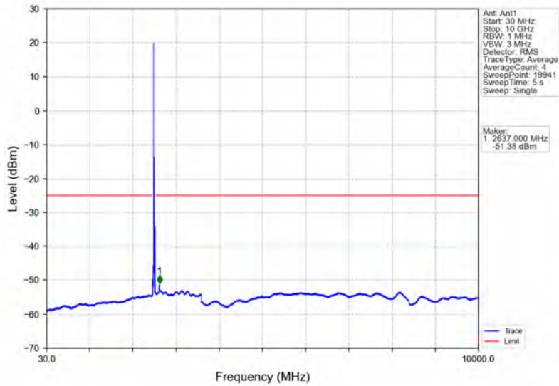
Band7_20MHz_16QAM_LCH_2510MHz_RB_1_0_NTNV
