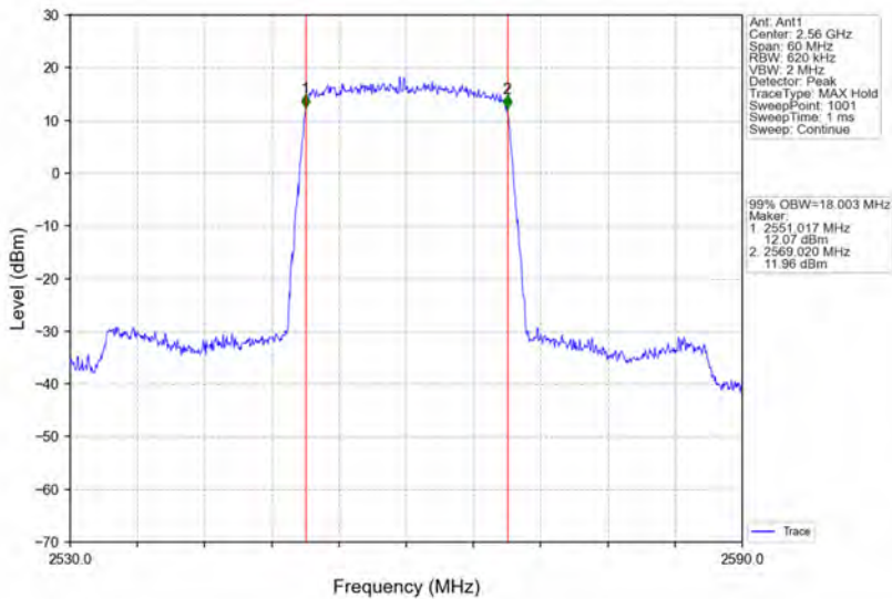
Band7_20MHz_QPSK_HCH_2560MHz_RB_100_0_NTNV
