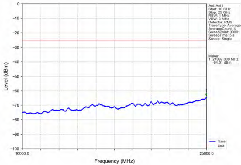
Band7_20MHz_QPSK_LCH_2510MHz_RB_1_0_NTNV
