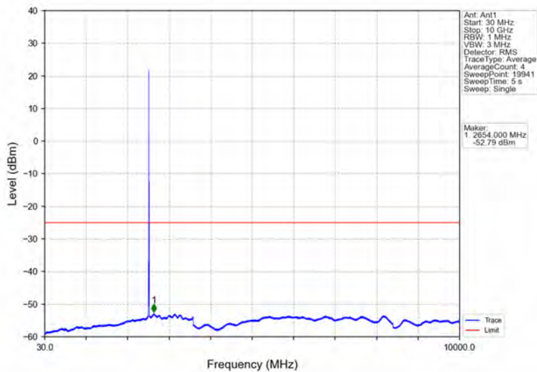
Band7_5MHz_QPSK_MCH_2535MHz_RB_1_0_NTNV
