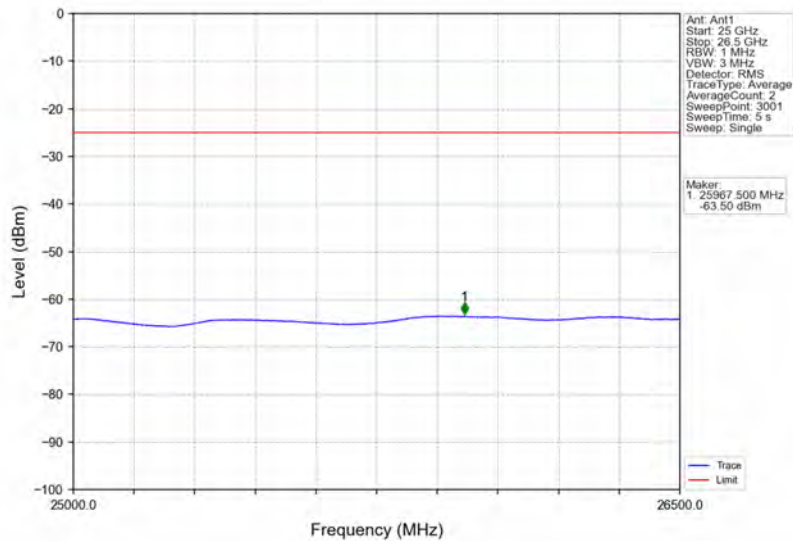
Band7_20MHz_QPSK_LCH_2510MHz_RB_1_0_NTNV
