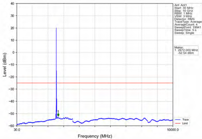
Band7_20MHz_16QAM_HCH_2560MHz_RB_1_0_NTNV
