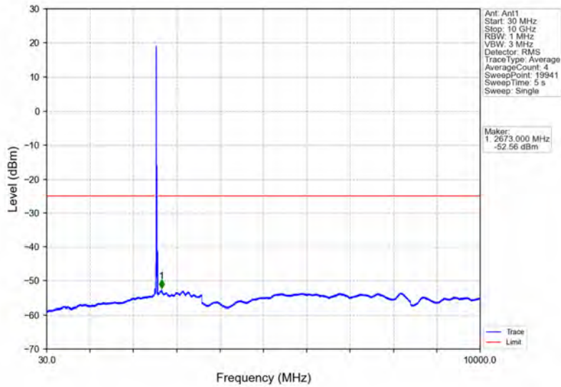
Band7_20MHz_64QAM_HCH_2560MHz_RB_1_0_NTNV
