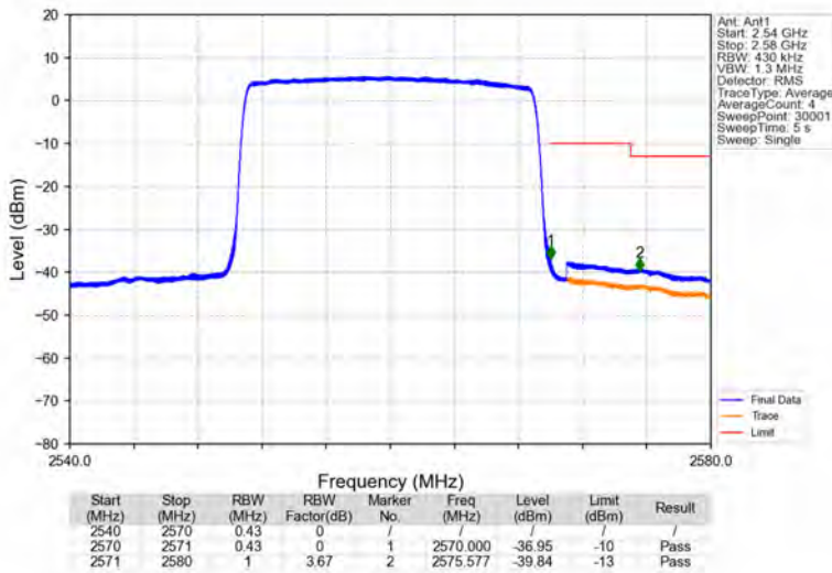
Band7_20MHz_16QAM_HCH_2560MHz_RB_100_0_NTNV
