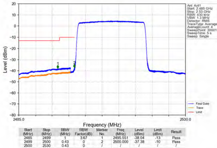
Band7_20MHz_64QAM_LCH_2510MHz_RB_100_0_NTNV
