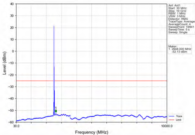
Band7_20MHz_QPSK_MCH_2535MHz_RB_1_0_NTNV
