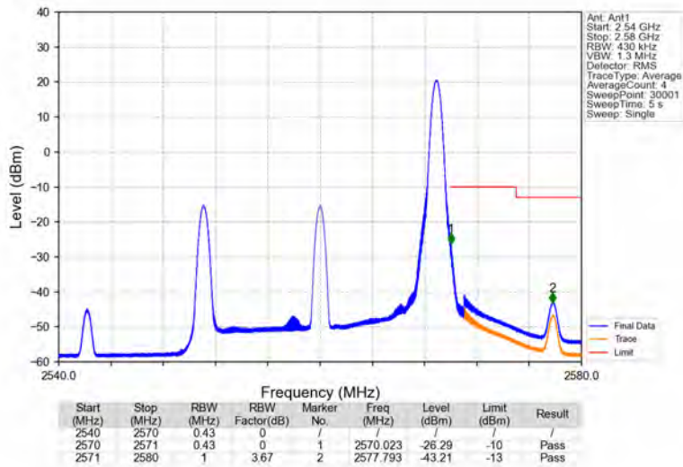
Band7_20MHz_QPSK_HCH_2560MHz_RB_1_99_NTNV
