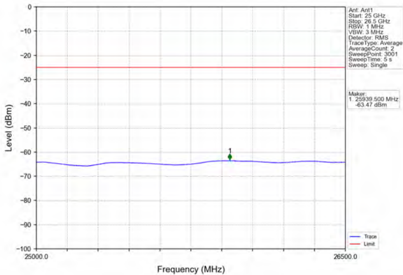
Band7_20MHz_QPSK_MCH_2535MHz_RB_1_0_NTNV
