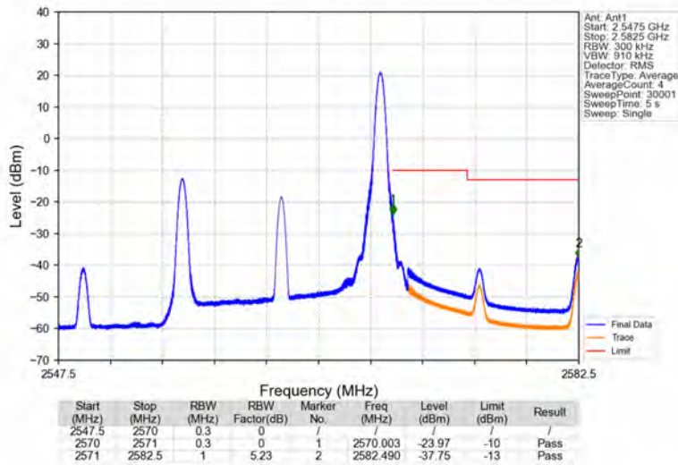
Band7_15MHz_QPSK_HCH_2562.5MHz_RB_1_74_NTNV
