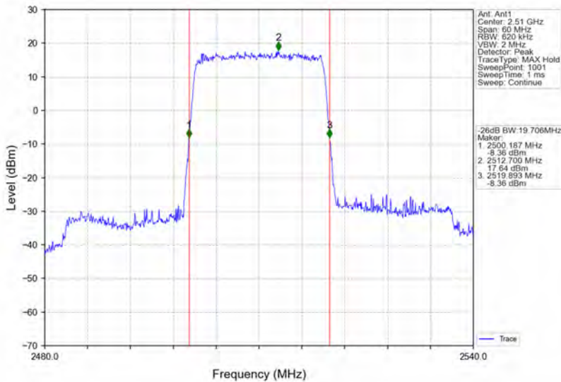
Band7_20MHz_QPSK_LCH_2510MHz_RB_100_0_NTNV
