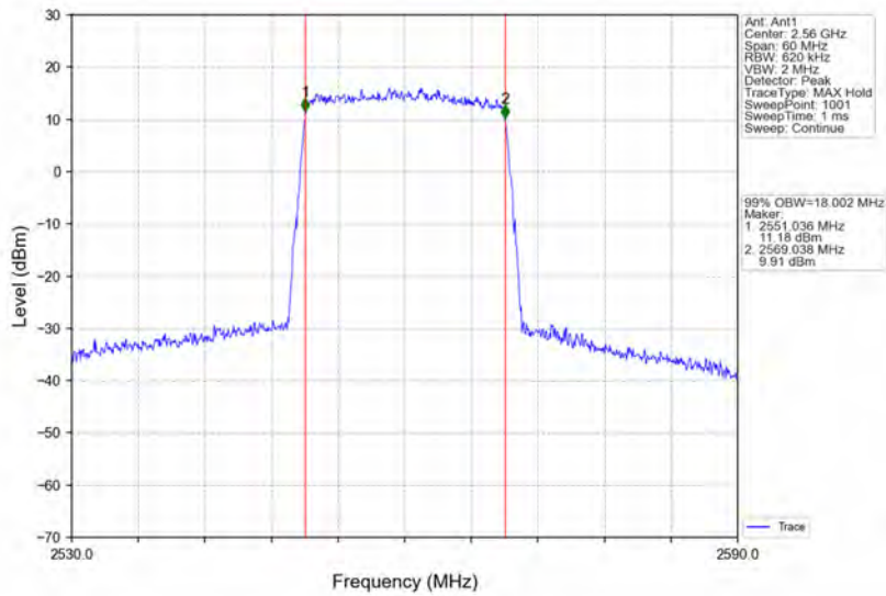
Band7_20MHz_64QAM_HCH_2560MHz_RB_100_0_NTNV
