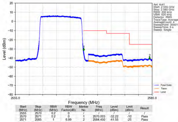
Band7_10MHz_QPSK_HCH_2565MHz_RB_50_0_NTNV
