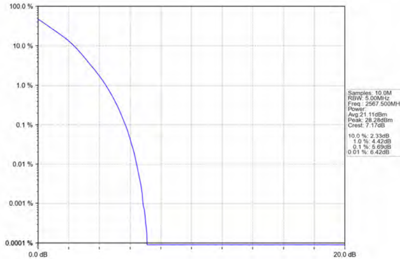
Band7_5MHz_QPSK_HCH_2567.5MHz_RB_25_0_NTNV
