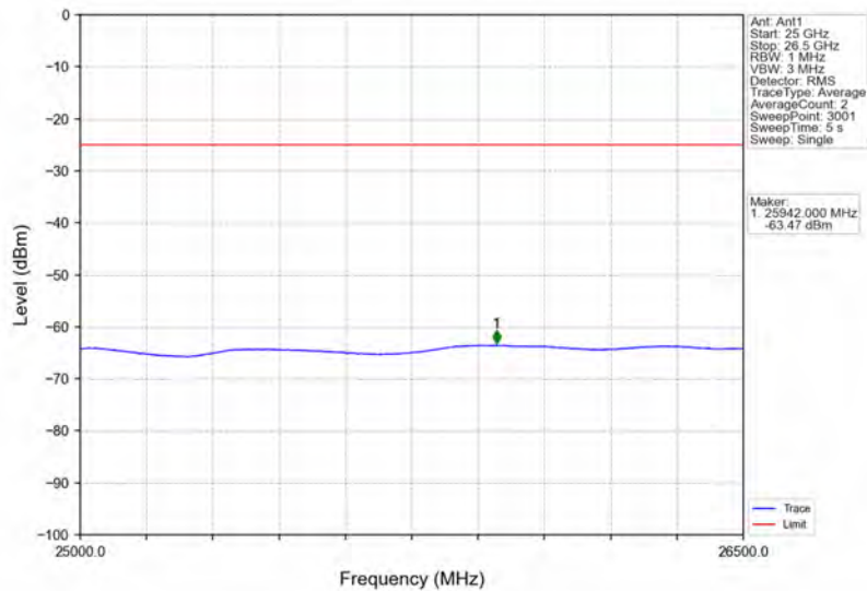
Band7_5MHz_QPSK_MCH_2535MHz_RB_1_0_NTNV
