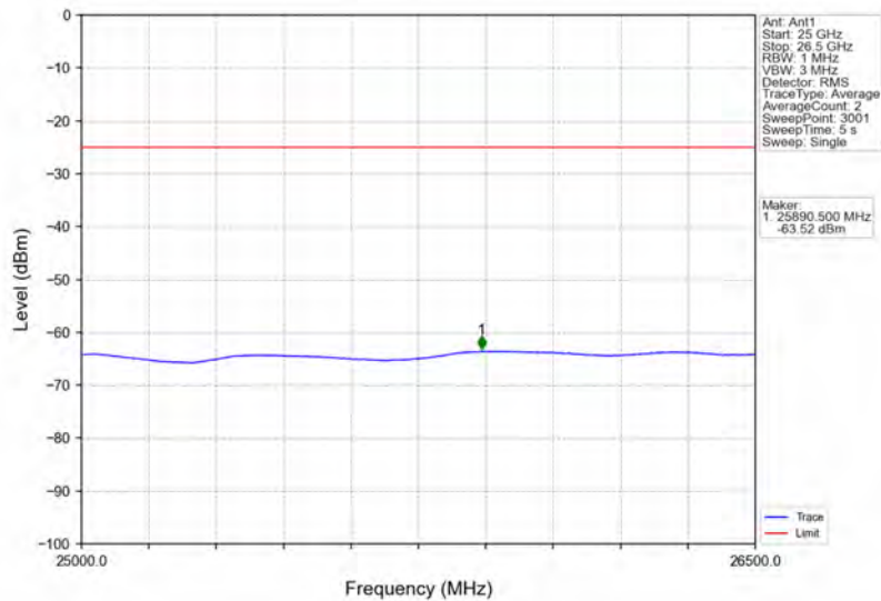
Band7_10MHz_QPSK_LCH_2505MHz_RB_1_0_NTNV
