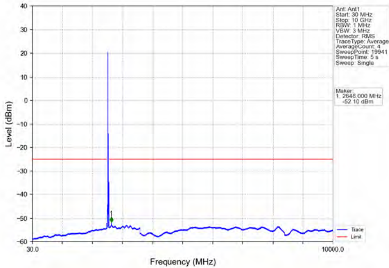
Band7_20MHz_16QAM_MCH_2535MHz_RB_1_0_NTNV
