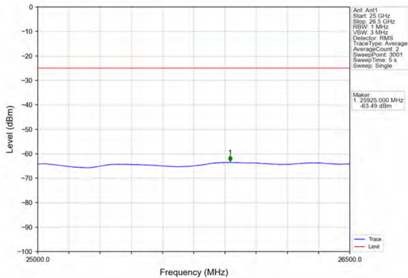
Band7_5MHz_QPSK_LCH_2502.5MHz_RB_1_0_NTNV
