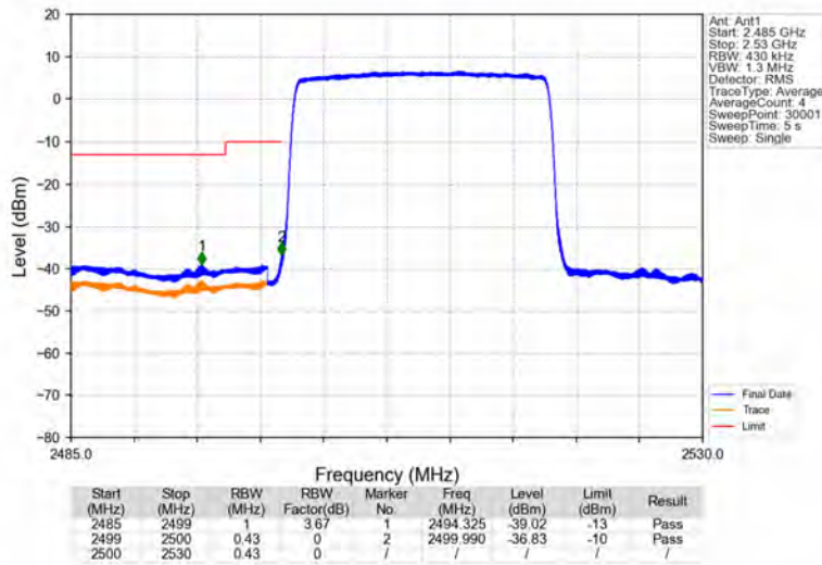
Band7_20MHz_QPSK_LCH_2510MHz_RB_100_0_NTNV
