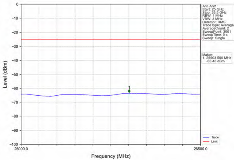
Band7_20MHz_16QAM_LCH_2510MHz_RB_100_0_NTNV
