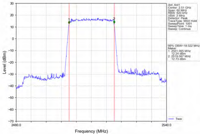
Band7_20MHz_QPSK_LCH_2510MHz_RB_100_0_NTNV
