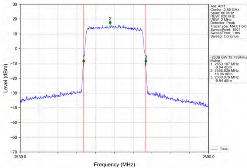
Band7_20MHz_64QAM_HCH_2560MHz_RB_100_0_NTNV
