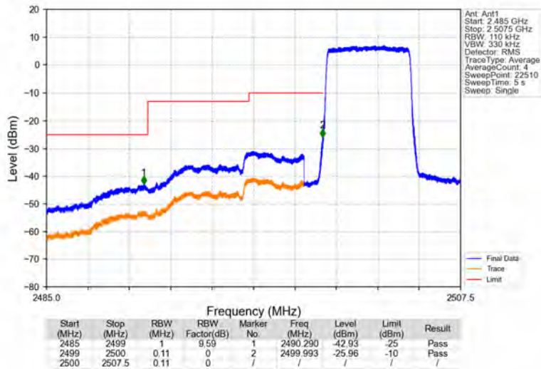
Band7_5MHz_QPSK_LCH_2502.5MHz_RB_25_0_NTNV
