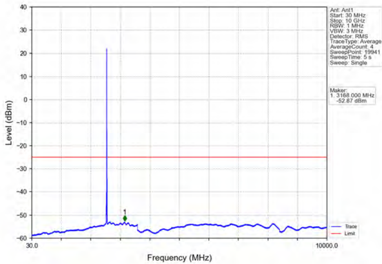
Band7_10MHz_QPSK_HCH_2565MHz_RB_1_0_NTNV
