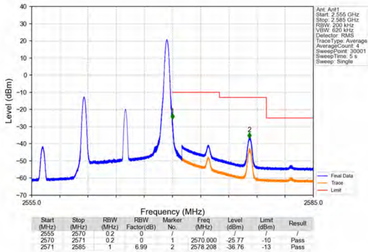
Band7_10MHz_QPSK_HCH_2565MHz_RB_1_49_NTNV
