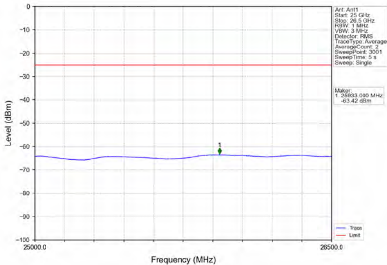
Band7_20MHz_64QAM_LCH_2510MHz_RB_1_0_NTNV
