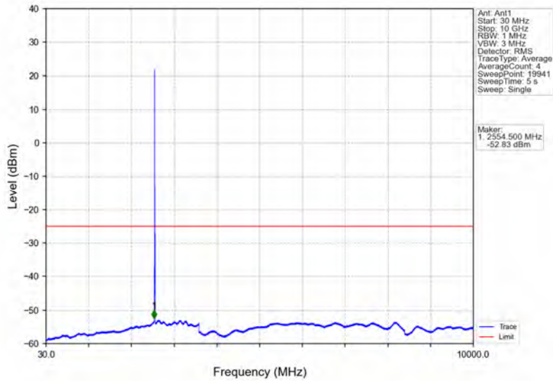
Band7_5MHz_QPSK_HCH_2567.5MHz_RB_1_0_NTNV
