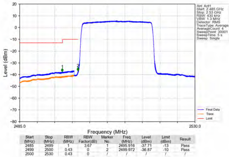
Band7_20MHz_16QAM_LCH_2510MHz_RB_100_0_NTNV
