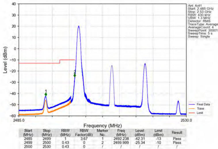
Band7_20MHz_16QAM_LCH_2510MHz_RB_1_0_NTNV
