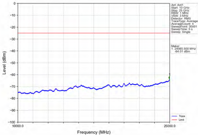
Band7_20MHz_16QAM_MCH_2535MHz_RB_1_0_NTNV
