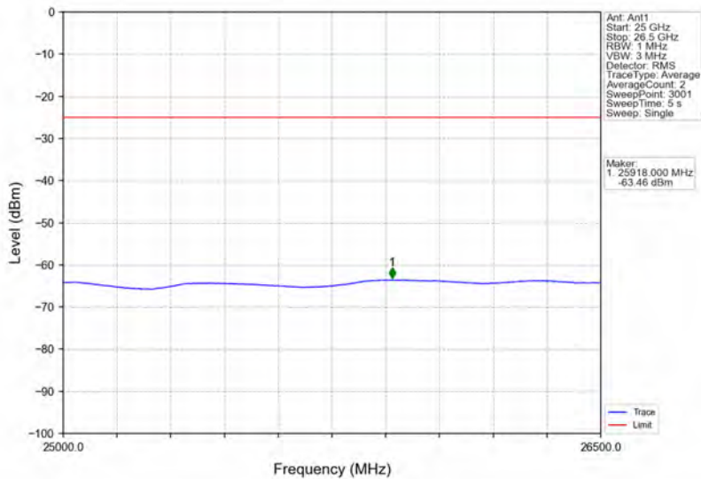
Band7_10MHz_QPSK_MCH_2535MHz_RB_1_0_NTNV
