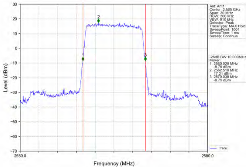
Band7_10MHz_QPSK_HCH_2565MHz_RB_50_0_NTNV
