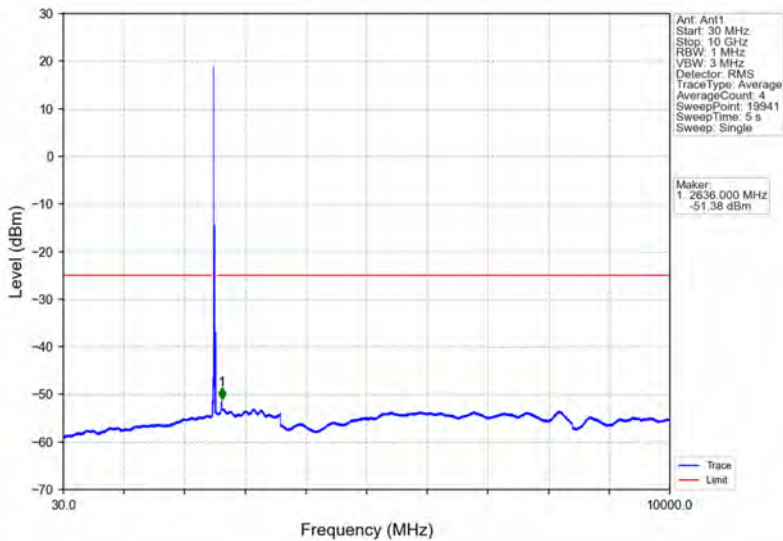
Band7_20MHz_64QAM_LCH_2510MHz_RB_1_0_NTNV
