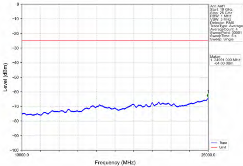
Band7_20MHz_QPSK_HCH_2560MHz_RB_1_0_NTNV
