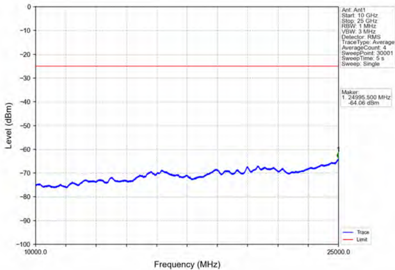
Band7_20MHz_64QAM_HCH_2560MHz_RB_1_0_NTNV
