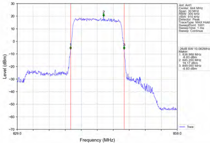
Band5_10MHz_QPSK_HCH_844MHz_RB_50_0_NTNV
