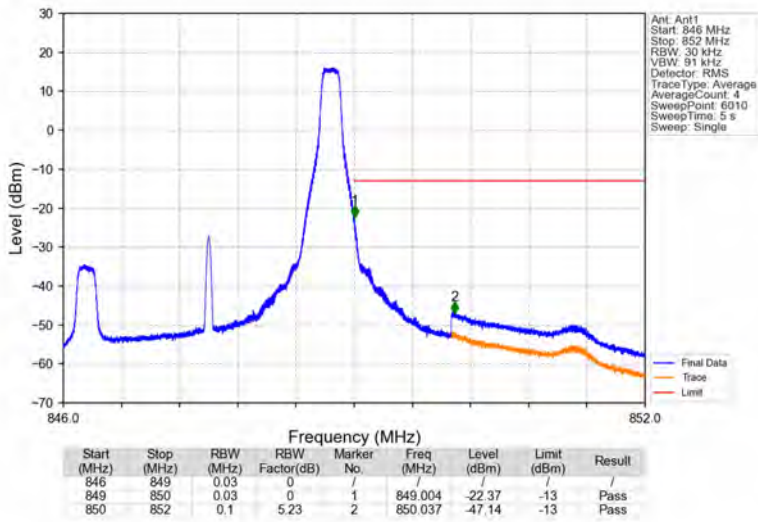
Band5_3MHz_QPSK_HCH_847.5MHz_RB_1_14_NTNV
