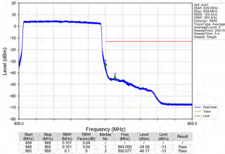
Band5_10MHz_QPSK_HCH_844MHz_RB_50_0_NTNV
