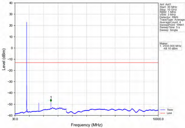
Band5_5MHz_QPSK_HCH_846.5MHz_RB_1_24_NTNV
