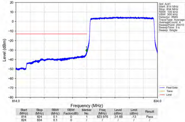
Band5_10MHz_QPSK_LCH_829MHz_RB_50_0_NTNV
