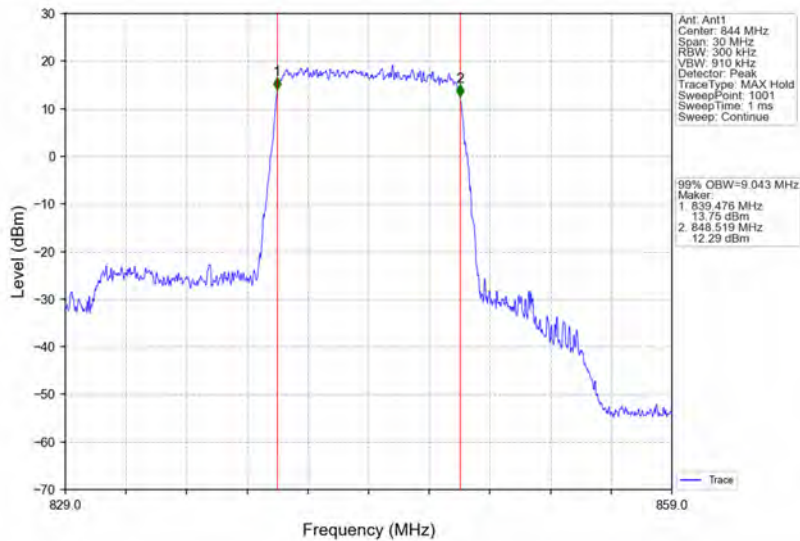
Band5_10MHz_QPSK_HCH_844MHz_RB_50_0_NTNV
