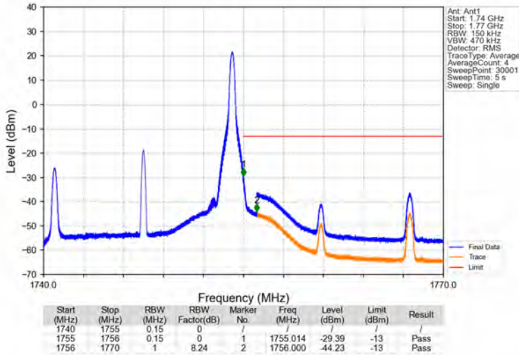
Band4_15MHz_QPSK_HCH_1747.5MHz_RB_1_74_NTNV
