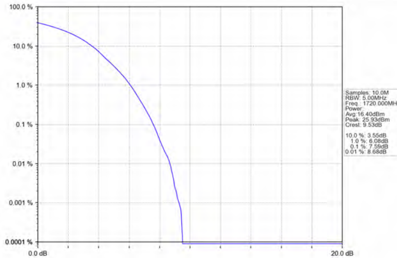
Band4_20MHz_16QAM_LCH_1720MHz_RB_100_0_NTNV
