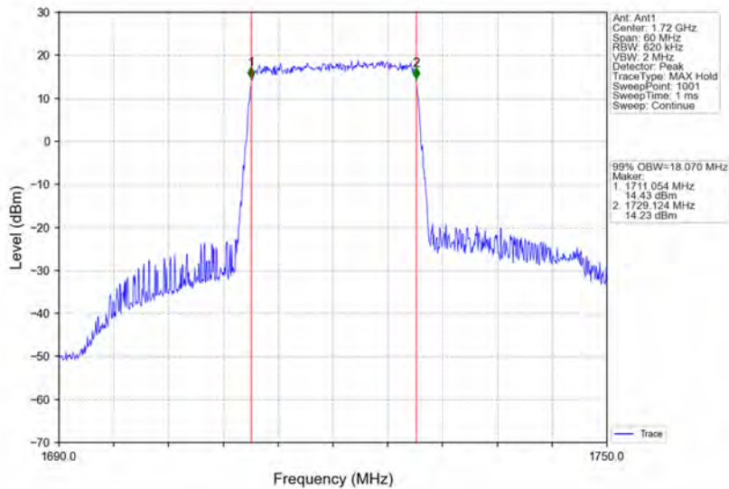
Band4_20MHz_QPSK_LCH_1720MHz_RB_100_0_NTNV
