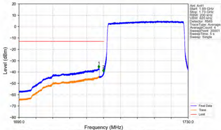
Band4_20MHz_QPSK_LCH_1720MHz_RB_100_0_NTNV
