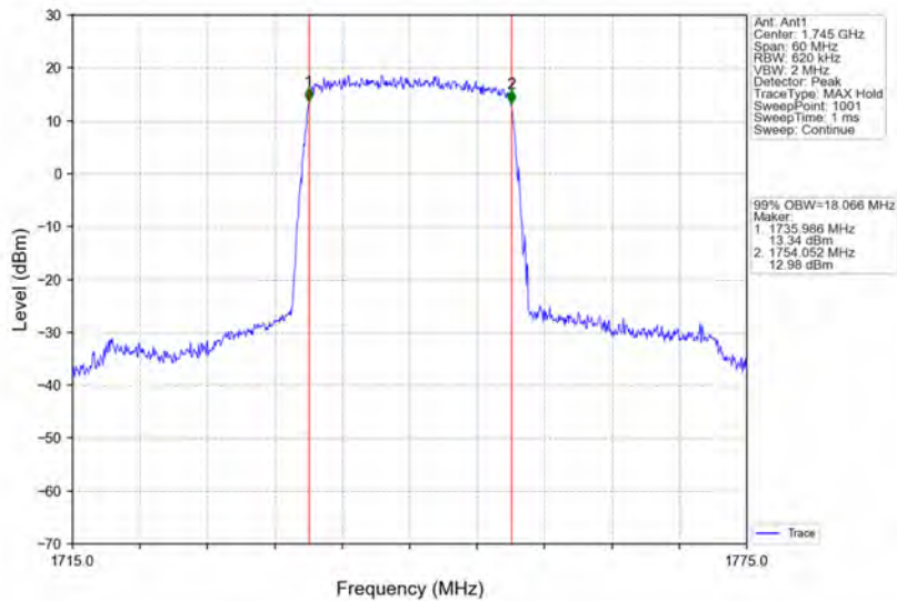
Band4_20MHz_QPSK_HCH_1745MHz_RB_100_0_NTNV
