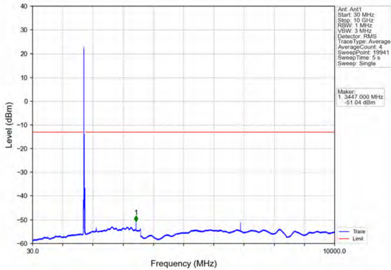
Band4_20MHz_QPSK_MCH_1732.5MHz_RB_1_0_NTNV
