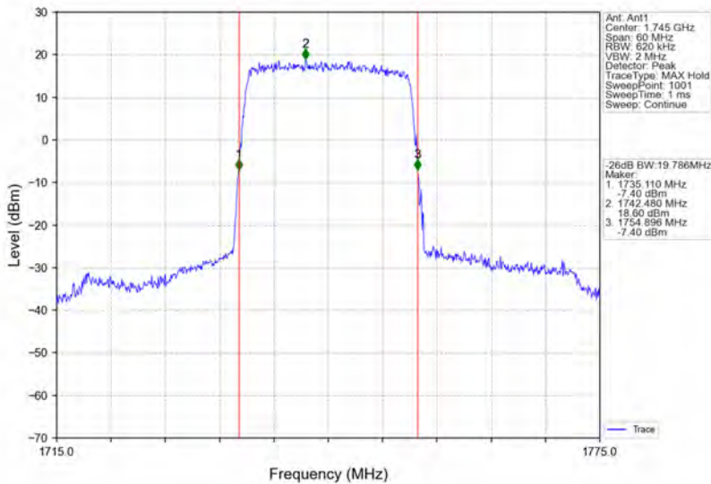
Band4_20MHz_QPSK_HCH_1745MHz_RB_100_0_NTNV
