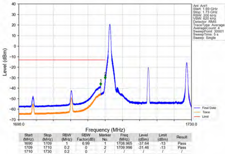
Band4_20MHz_16QAM_LCH_1720MHz_RB_1_0_NTNV
