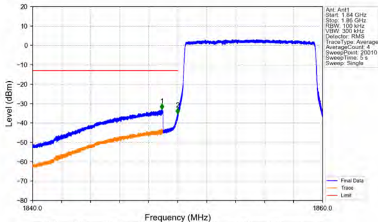
Band2_10MHz_16QAM_LCH_1855MHz_RB_50_0_NTNV
