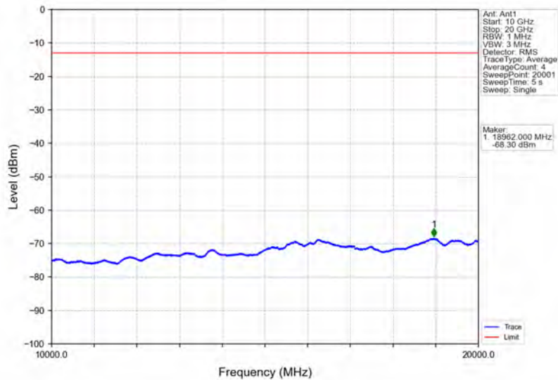
Band2_3MHz_QPSK_MCH_1880MHz_RB_1_0_NTNV
