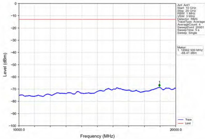
Band2_3MHz_16QAM_MCH_1880MHz_RB_1_0_NTNV
