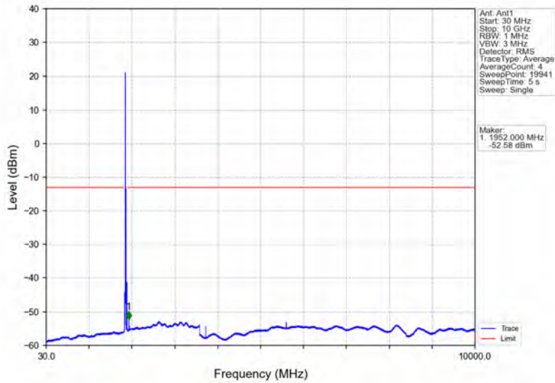
Band2_20MHz_64QAM_MCH_1880MHz_RB_1_0_NTNV
