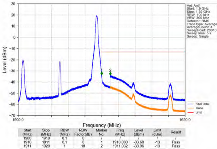
Band2_10MHz_16QAM_HCH_1905MHz_RB_1_49_NTNV
