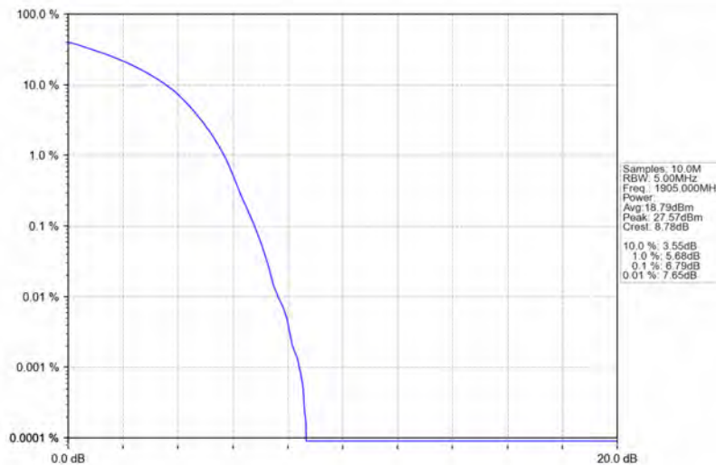
Band2_10MHz_16QAM_HCH_1905MHz_RB_50_0_NTNV
