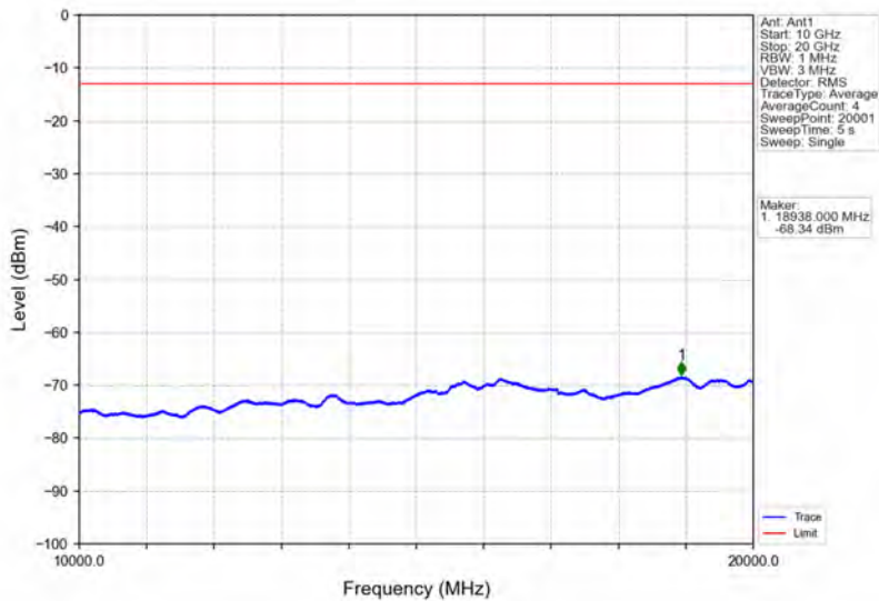
Band2_20MHz_QPSK_MCH_1880MHz_RB_1_0_NTNV
