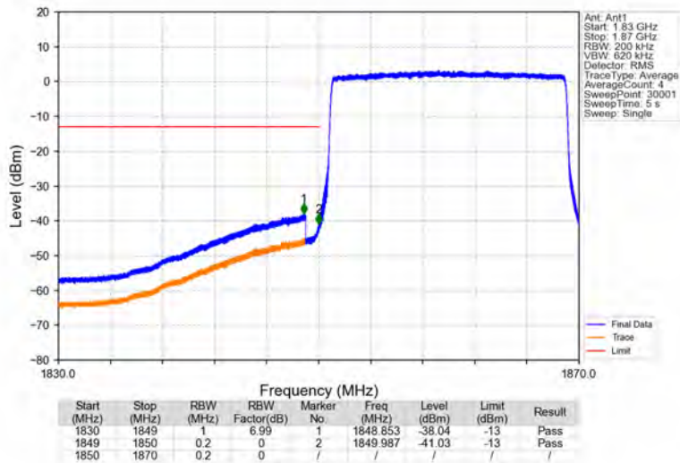
Band2_20MHz_16QAM_LCH_1860MHz_RB_100_0_NTNV
