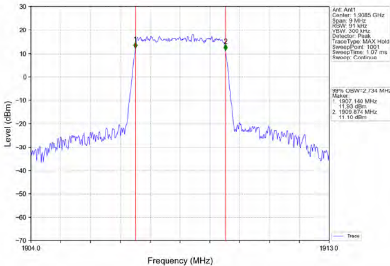
Band2_3MHz_QPSK_HCH_1908.5MHz_RB_15_0_NTNV
