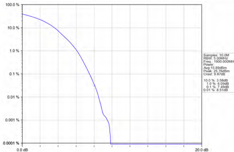
Band2_20MHz_16QAM_HCH_1900MHz_RB_100_0_NTNV
