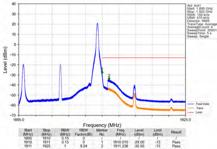
Band2_15MHz_16QAM_HCH_1902.5MHz_RB_1_74_NTNV
