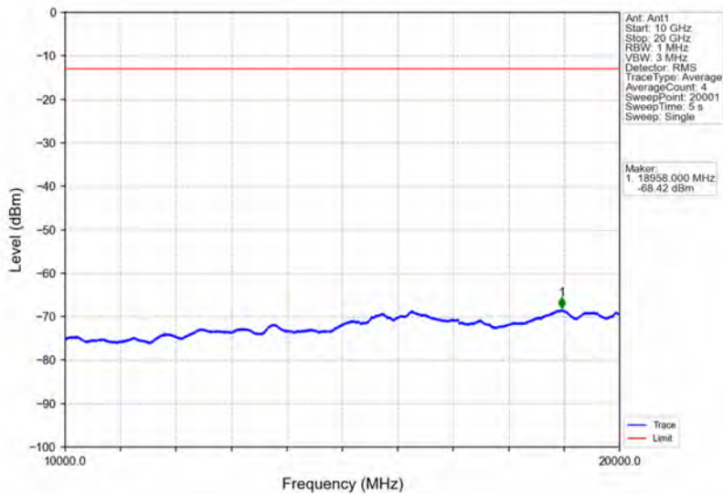
Band2_10MHz_QPSK_MCH_1880MHz_RB_1_0_NTNV
