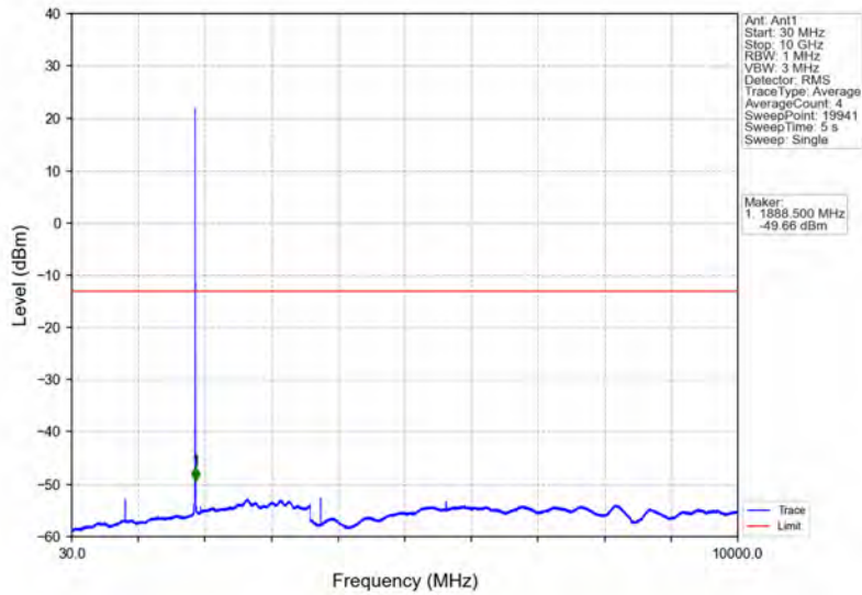
Band2_3MHz_QPSK_MCH_1880MHz_RB_1_0_NTNV
