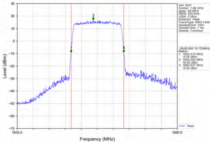
Band2_20MHz_64QAM_LCH_1860MHz_RB_100_0_NTNV
