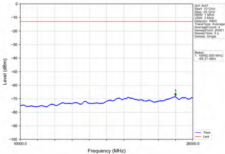
Band2_20MHz_QPSK_HCH_1900MHz_RB_1_0_NTNV
