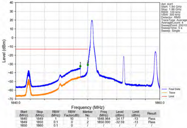
Band2_10MHz_16QAM_LCH_1855MHz_RB_1_0_NTNV
