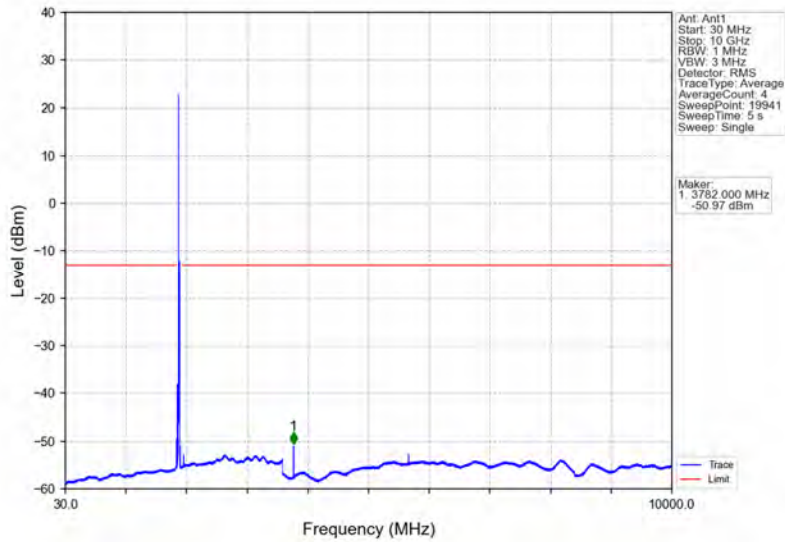
Band2_20MHz_QPSK_HCH_1900MHz_RB_1_0_NTNV
