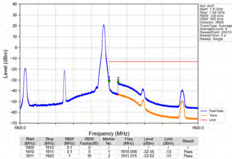
Band2_10MHz_QPSK_HCH_1905MHz_RB_1_49_NTNV
