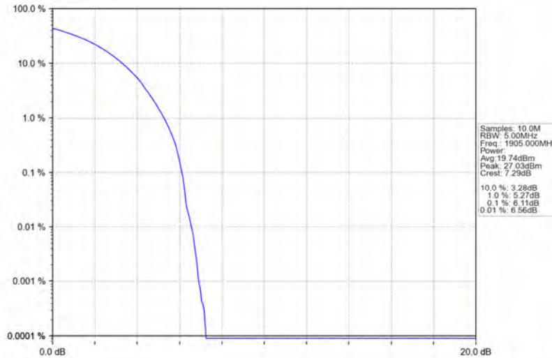
Band2_10MHz_QPSK_HCH_1905MHz_RB_50_0_NTNV
