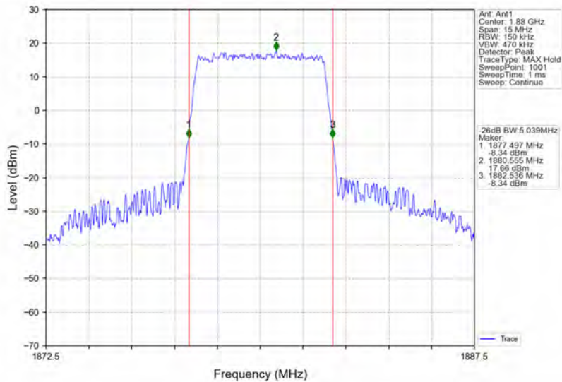
Band2_5MHz_QPSK_MCH_1880MHz_RB_25_0_NTNV
