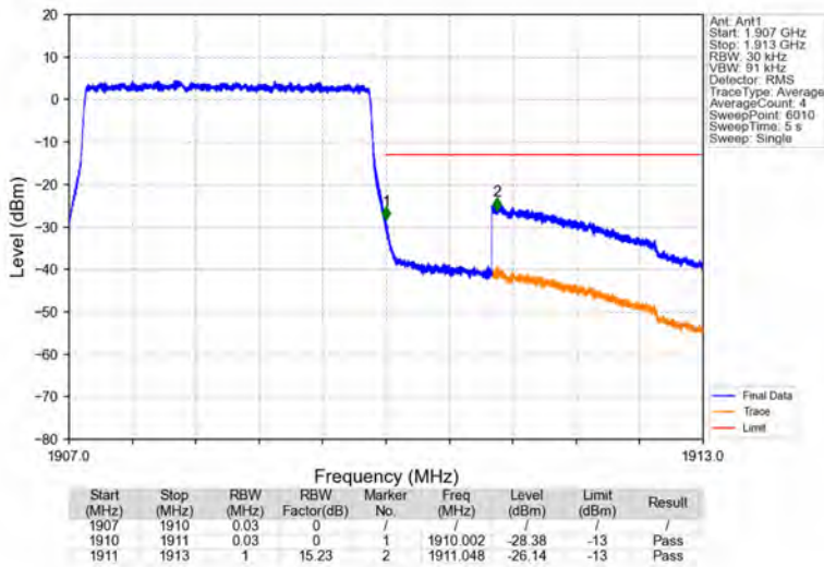
Band2_3MHz_QPSK_HCH_1908.5MHz_RB_15_0_NTNV
