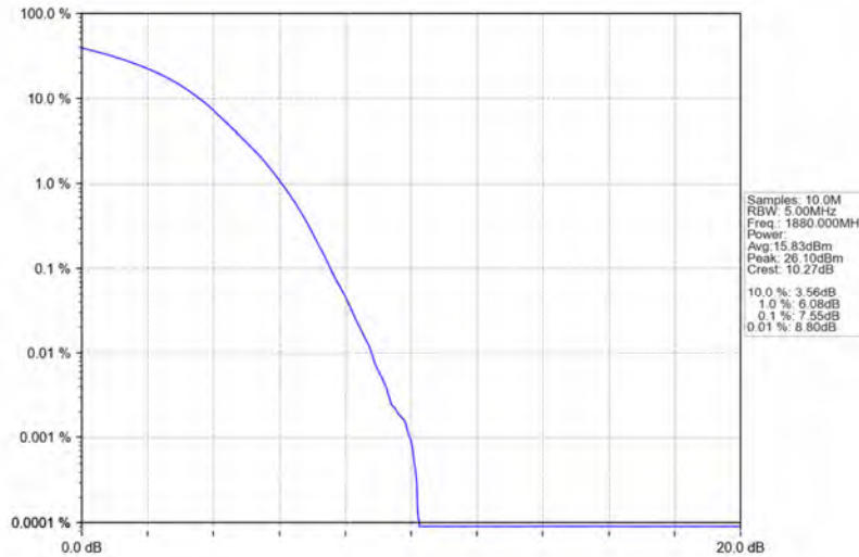
Band2_20MHz_16QAM_MCH_1880MHz_RB_100_0_NTNV
