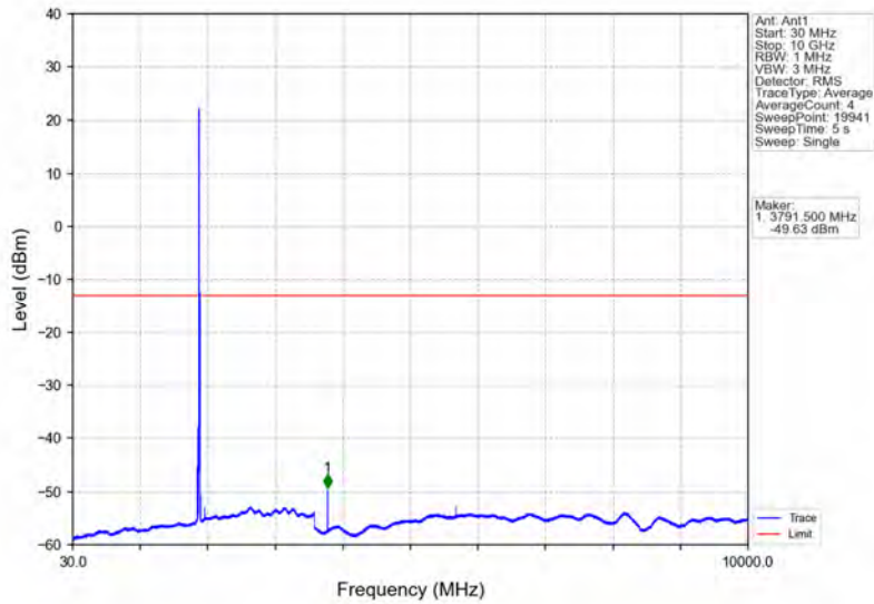
Band2_15MHz_QPSK_HCH_1902.5MHz_RB_1_0_NTNV
