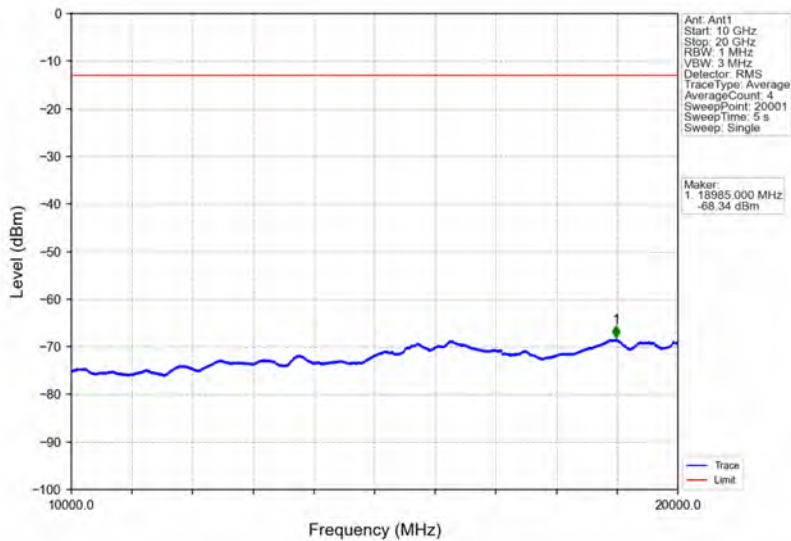
Band2_10MHz_16QAM_MCH_1880MHz_RB_1_0_NTNV
