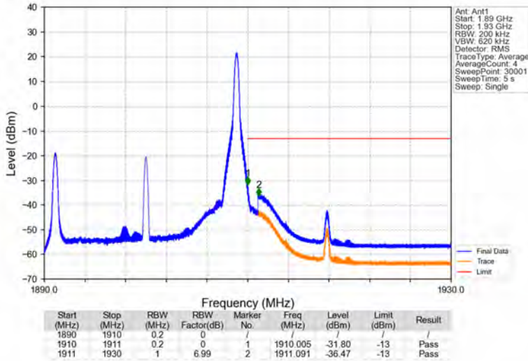
Band2_20MHz_16QAM_HCH_1900MHz_RB_1_99_NTNV
