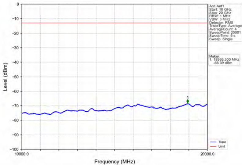
Band2_1.4MHz_QPSK_HCH_1909.3MHz_RB_1_0_NTNV
