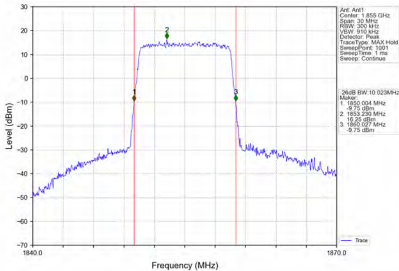
Band2_10MHz_64QAM_LCH_1855MHz_RB_50_0_NTNV
