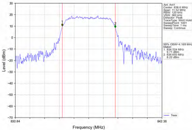
Band5_HSUPA_MCH_836.6MHz_Subtest 1_NTNV
