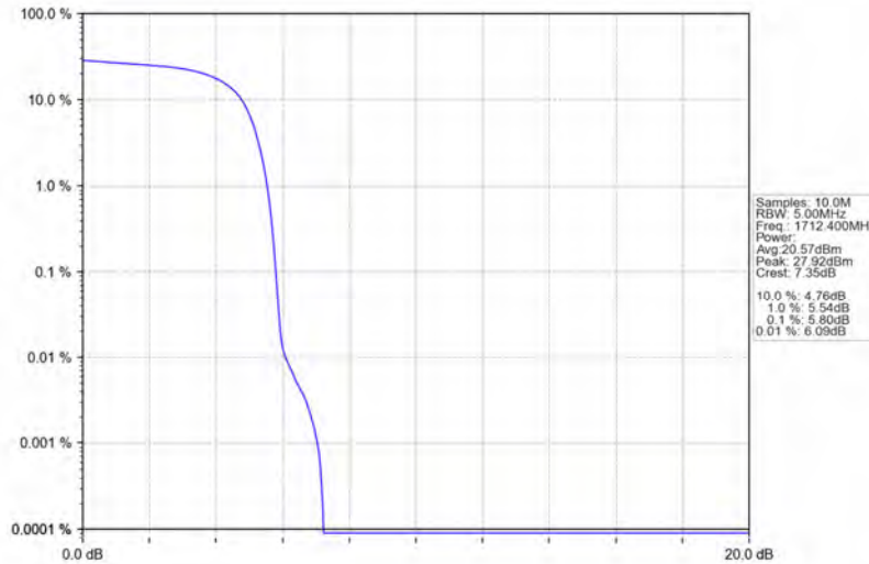
Band4_HSUPA_LCH_1712.4MHz_Subtest 1_NTNV
