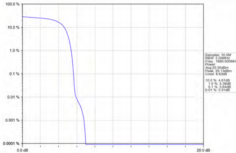
Band2_HSUPA_MCH_1880MHz_Subtest 1_NTNV
