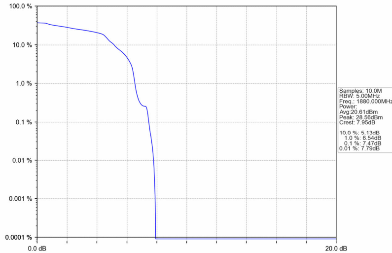
PCS1900_EGPRS_MCH_1880MHz_4 TX Slots_NTNV
