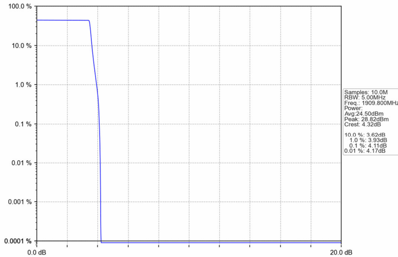
PCS1900_GPRS_HCH_1909.8MHz_4 TX Slots_NTNV
