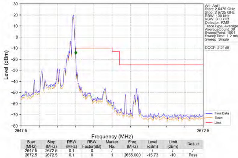
Band41_5MHz_QPSK_HCH_2652.5MHz_RB_1_24_NTNV
