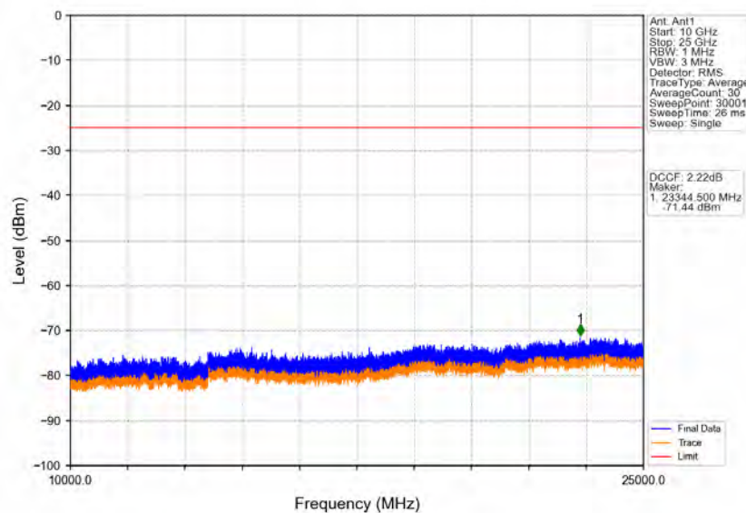
Band41_5MHz_QPSK_HCH_2652.5MHz_RB_1_0_NTNV
