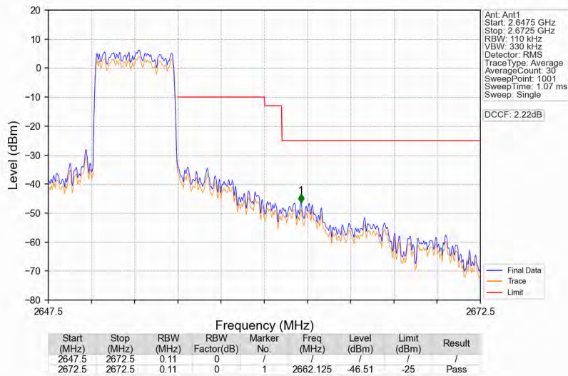
Band41_5MHz_QPSK_HCH_2652.5MHz_RB_25_0_NTNV
