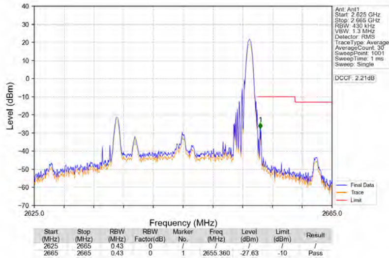
Band41_20MHz_QPSK_HCH_2645MHz_RB_1_99_NTNV
