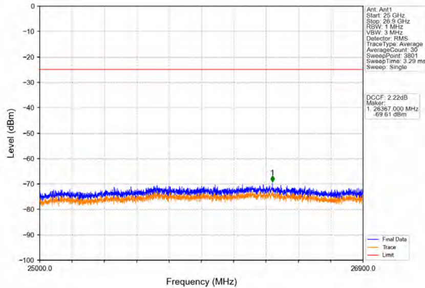
Band41_5MHz_QPSK_HCH_2652.5MHz_RB_1_24_NTNV
