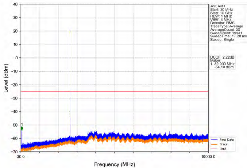
Band41_5MHz_QPSK_HCH_2652.5MHz_RB_1_0_NTNV
