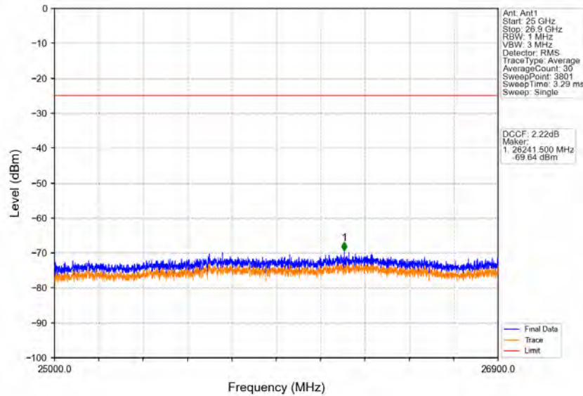
Band41_10MHz_QPSK_HCH_2650MHz_RB_1_49_NTNV
