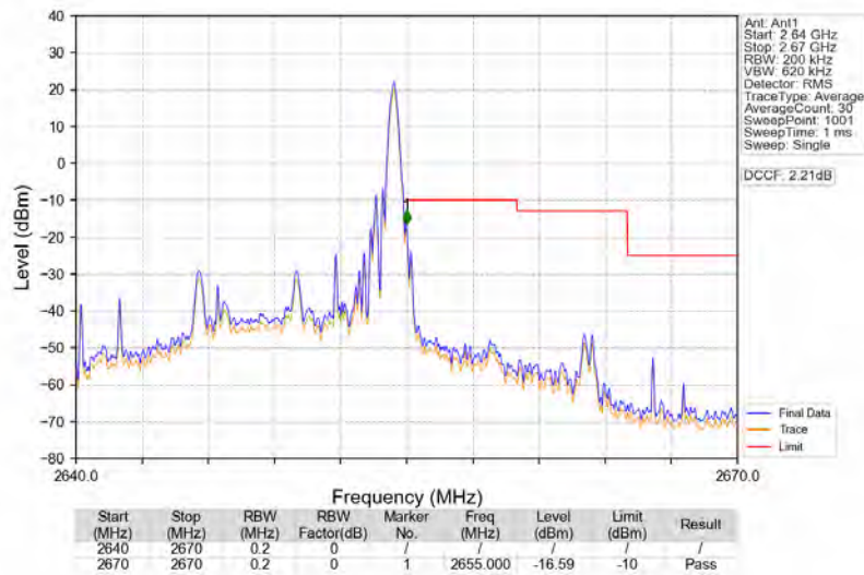
Band41_10MHz_QPSK_HCH_2650MHz_RB_1_49_NTNV
