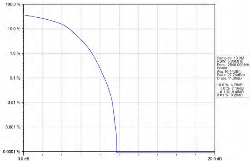
Band41_10MHz_16QAM_LCH_2540MHz_RB_50_0_NTNV
