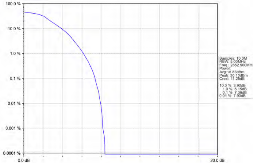
Band41_5MHz_QPSK_HCH_2652.5MHz_RB_25_0_NTNV
