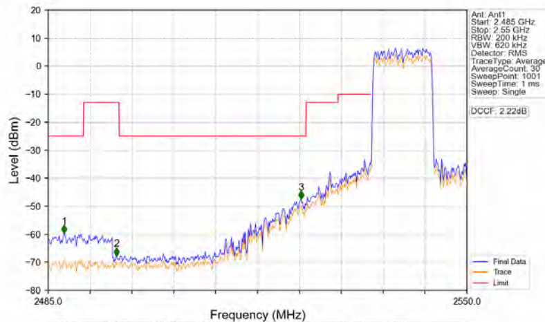
Band41_10MHz_16QAM_LCH_2540MHz_RB_50_0_NTNV
