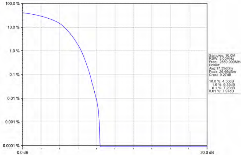
Band41_10MHz_QPSK_HCH_2650MHz_RB_50_0_NTNV
