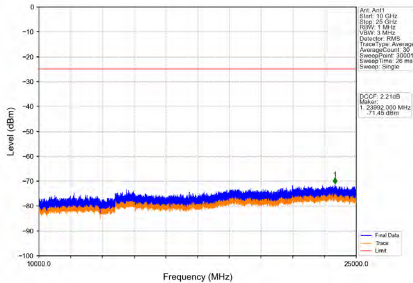
Band41_20MHz_QPSK_HCH_2645MHz_RB_1_0_NTNV
