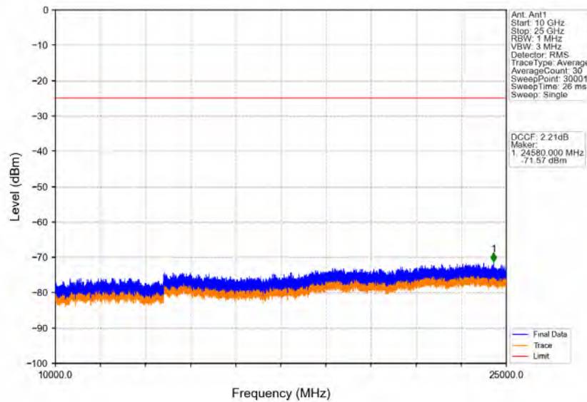
Band41_20MHz_16QAM_MCH_2595MHz_RB_1_0_NTNV
