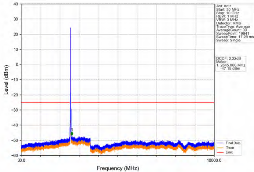
Band38_20MHz_16QAM_LCH_2580MHz_RB_1_0_NTV
