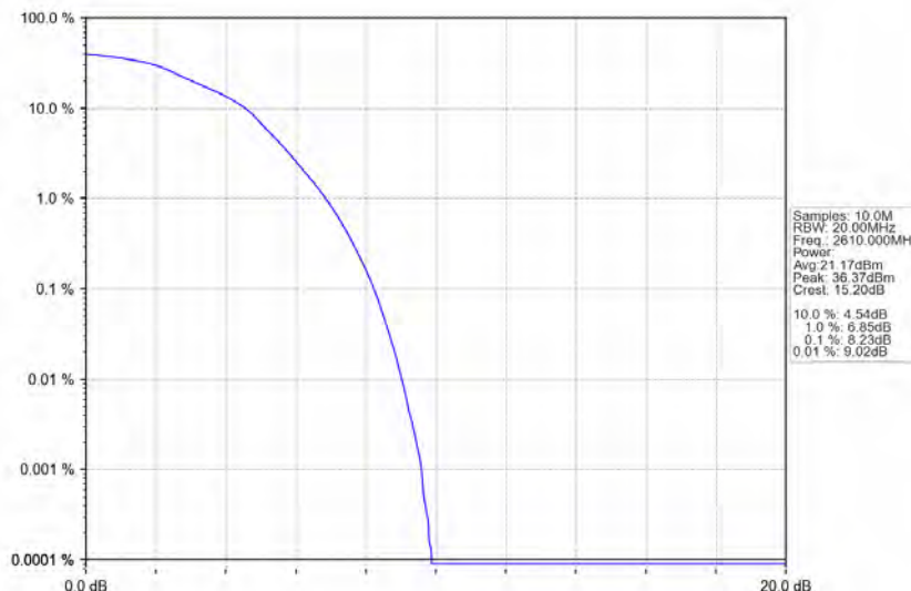
Band38_20MHz_16QAM_HCH_2610MHz_RB_100_0_NTNV
