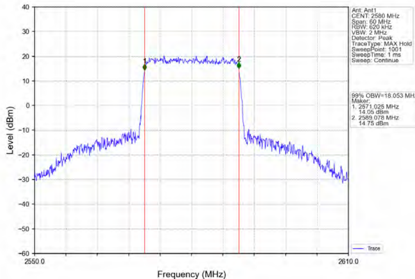
Band38_20MHz_16QAM_LCH_2580MHz_RB_100_0_NTNV
