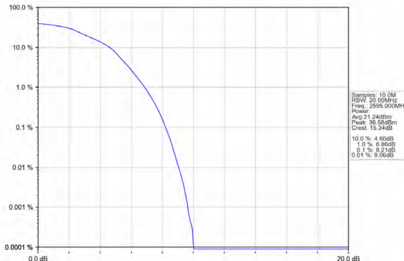
Band38_20MHz_16QAM_MCH_2595MHz_RB_100_0_NTNV
