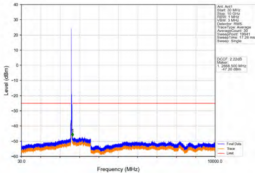
Band38_20MHz_QPSK_HCH_2610MHz_RB_1_0_NTNV
