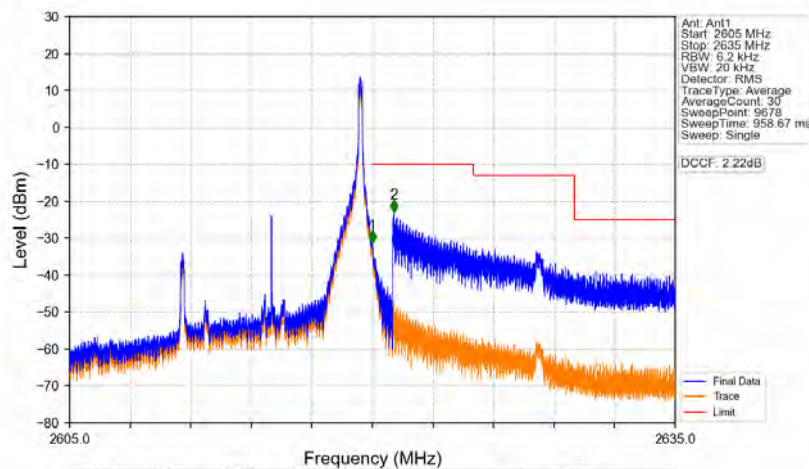
Band38_10MHz_QPSK_HCH_2615MHz_RB_1_49_NTNV
