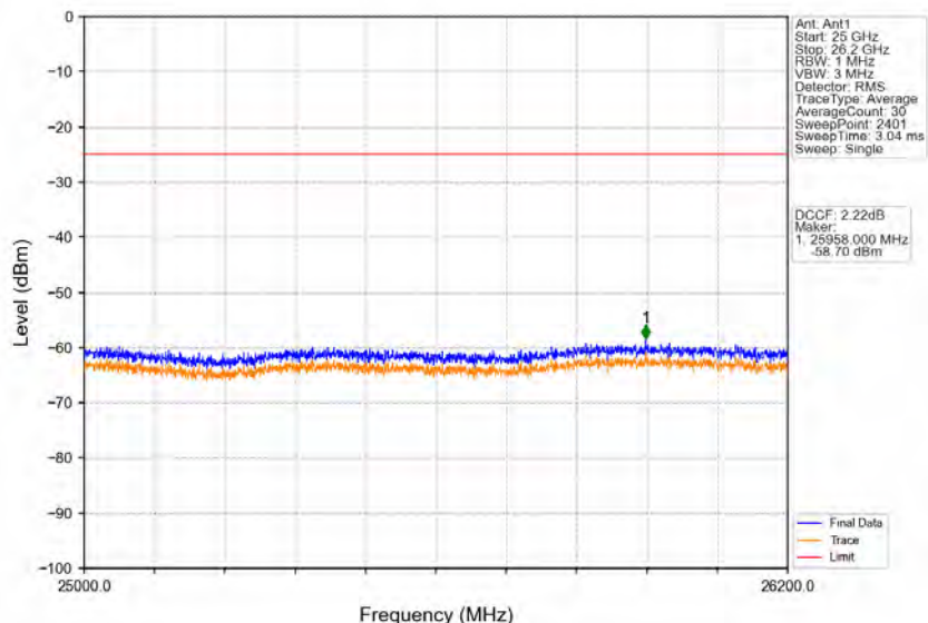
Band38_5MHz_QPSK_HCH_2617.5MHz_RB_1_24_NTNV
