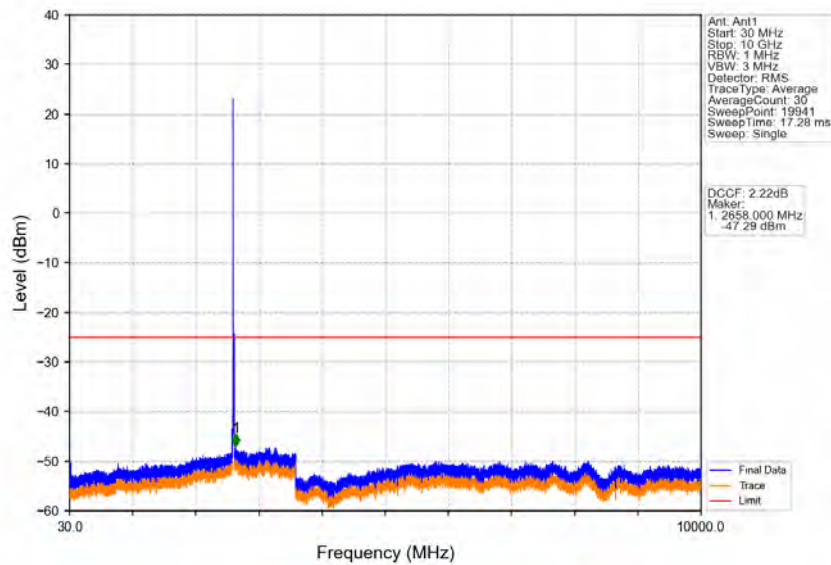
Band38_10MHz_QPSK_HCH_2615MHz_RB_1_0_NTNV
