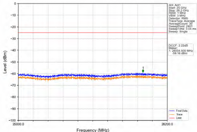
Band38_20MHz_QPSK_HCH_2610MHz_RB_1_99_NTNV
