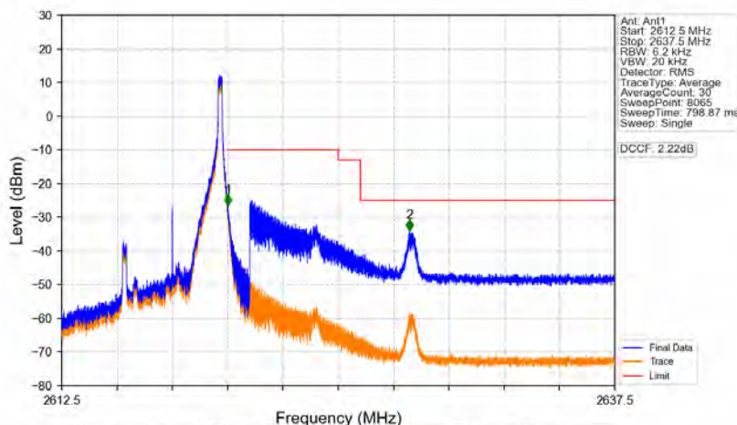
Band38_5MHz_QPSK_HCH_2617.5MHz_RB_1_24_NTNV
