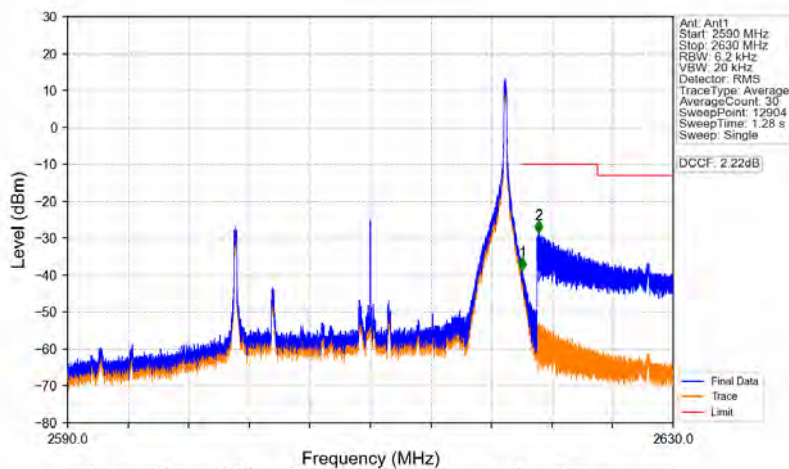
Band38_20MHz_QPSK_HCH_2610MHz_RB_1_99_NTNV
