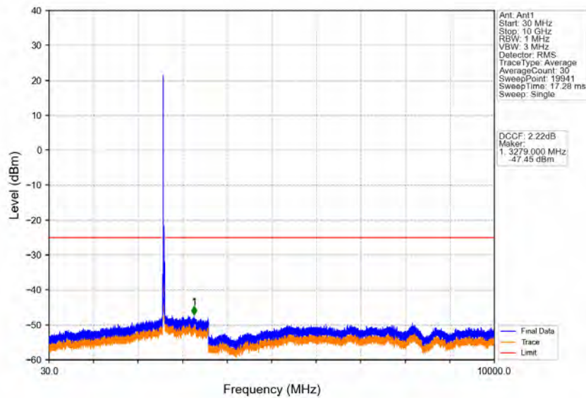
Band38_20MHz_16QAM_MCH_2595MHz_RB_1_0_NTNV
