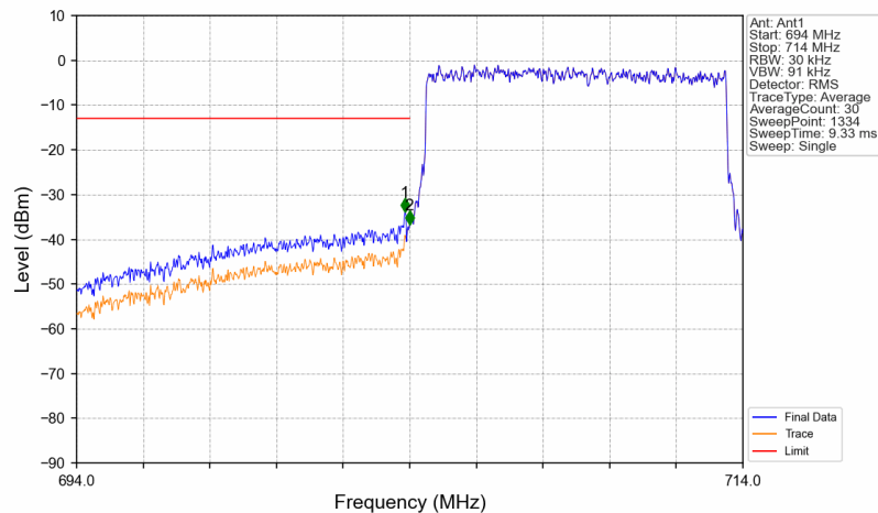
Band17_10MHz_QPSK_LCH_709MHz_RB_50_0_NTNV
