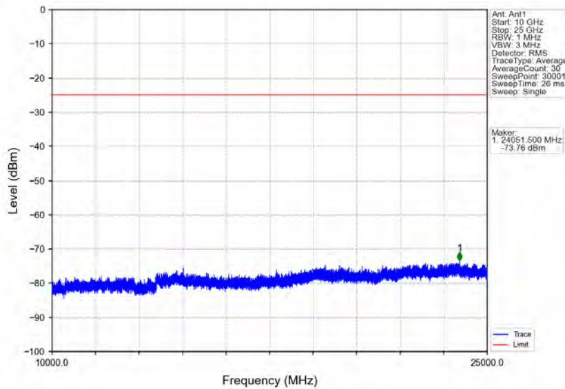
Band7_5MHz_QPSK_LCH_2502.5MHz_RB_1_0_NTNV
