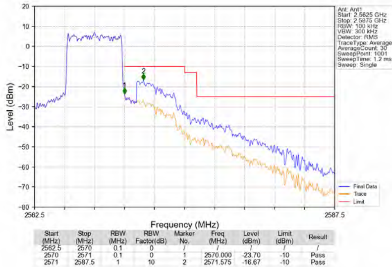
Band7_5MHz_QPSK_HCH_2567.5MHz_RB_25_0_NTNV
