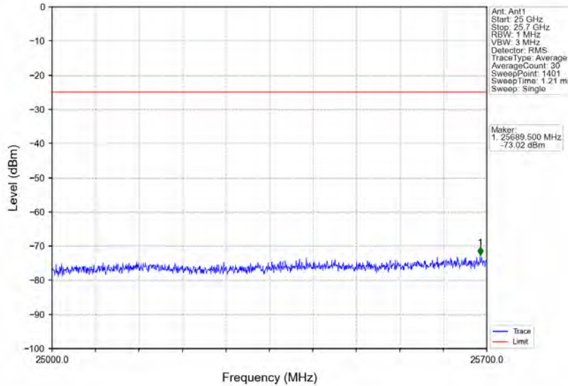
Band7_20MHz_QPSK_HCH_2560MHz_RB_1_99_NTNV
