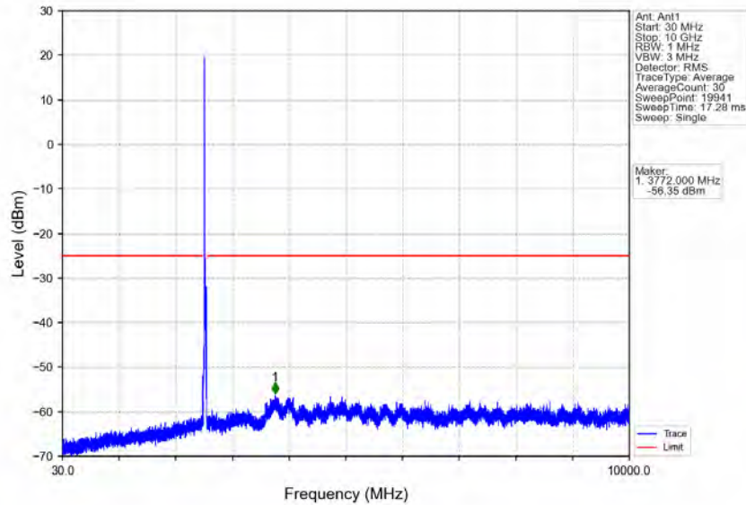
Band7_20MHz_16QAM_MCH_2535MHz_RB_1_0_NTNV
