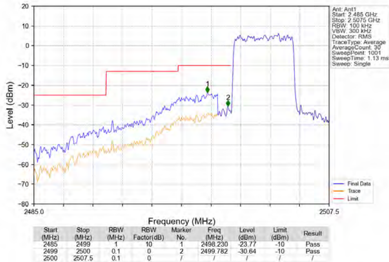
Band7_5MHz_QPSK_LCH_2502.5MHz_RB_25_0_NTNV
