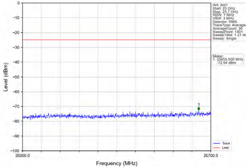
Band7_20MHz_16QAM_LCH_2510MHz_RB_100_0_NTNV
