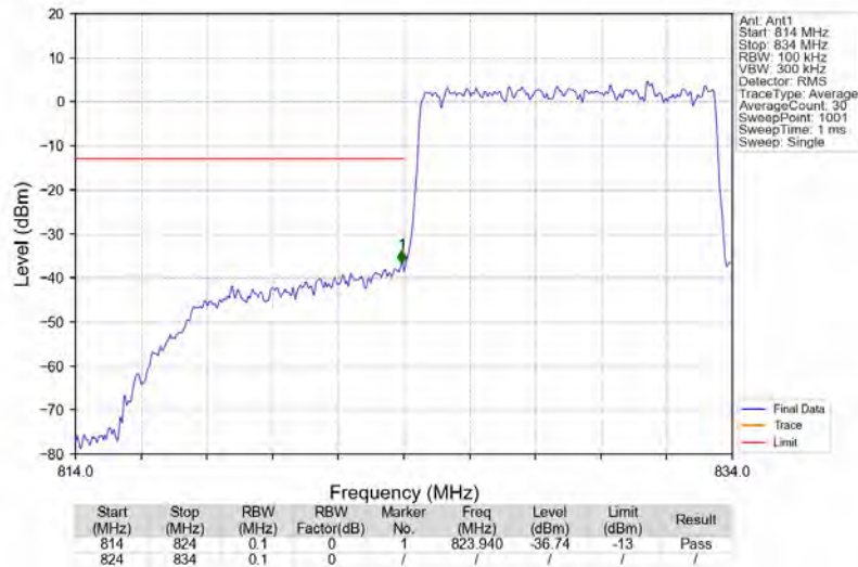
Band5_10MHz_QPSK_LCH_829MHz_RB_50_0_NTNV
