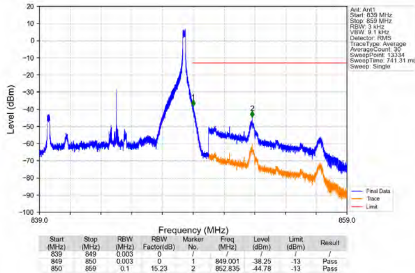
Band5_10MHz_QPSK_HCH_844MHz_RB_1_49_NTNV
