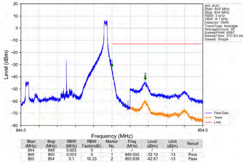
Band5_5MHz_QPSK_HCH_846.5MHz_RB_1_24_NTNV
