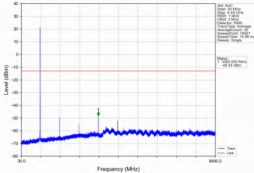
Band5_3MHz_QPSK_HCH_847.5MHz_RB_1_14_NTNV
