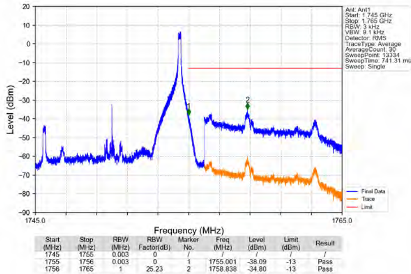
Band4_10MHz_QPSK_HCH_1750MHz_RB_1_49_NTNV
