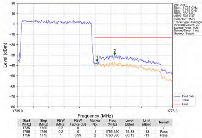
Band4_20MHz_QPSK_HCH_1745MHz_RB_100_0_NTNV
