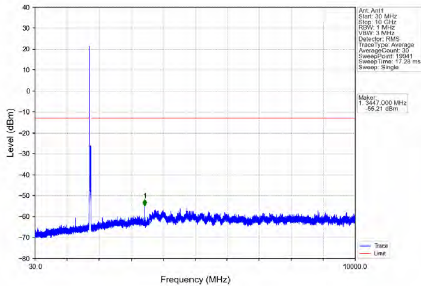
Band4_20MHz_QPSK_MCH_1732.5MHz_RB_1_0_NTV
