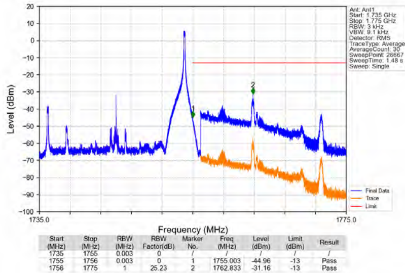
Band4_20MHz_QPSK_HCH_1745MHz_RB_1_99_NTNV
