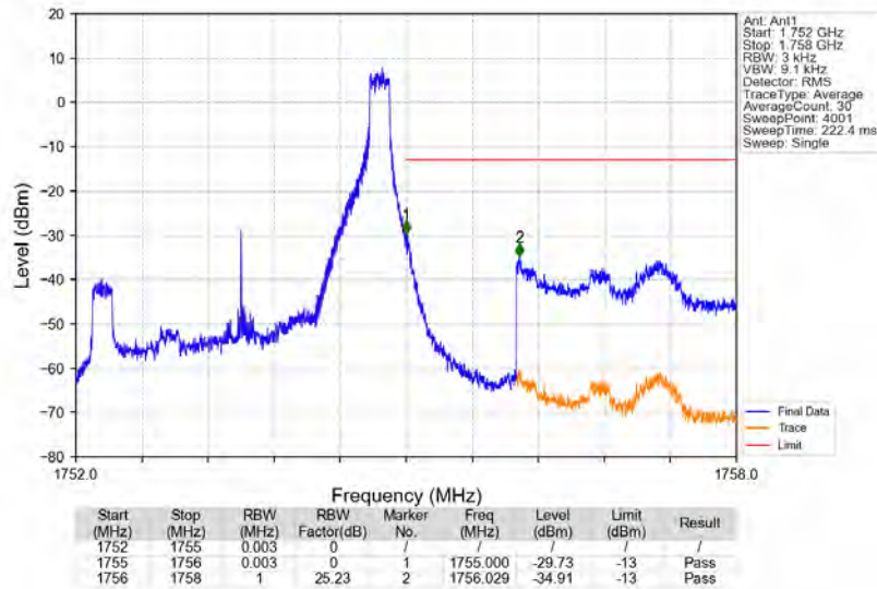
Band4_3MHz_QPSK_HCH_1753.5MHz_RB_1_14_NTNV
