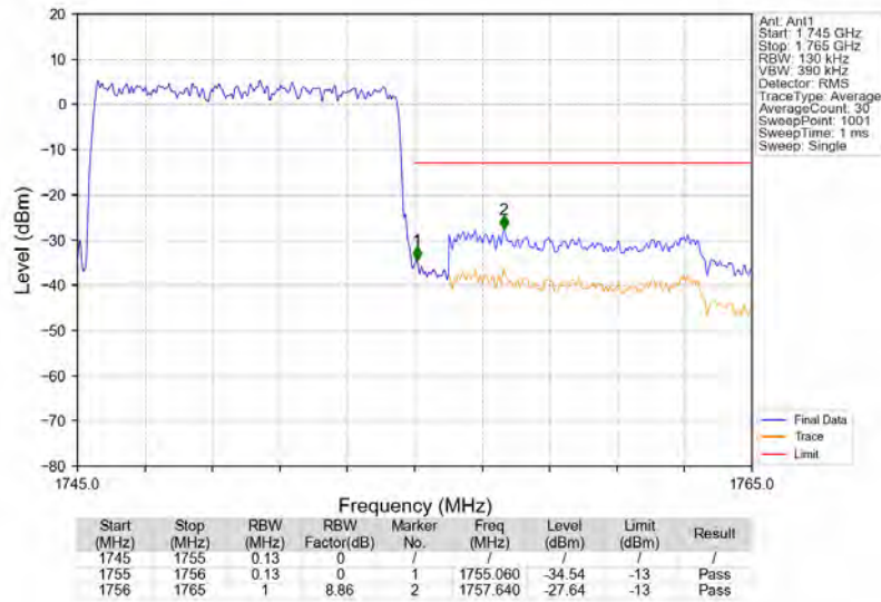
Band4_10MHz_QPSK_HCH_1750MHz_RB_50_0_NTNV
