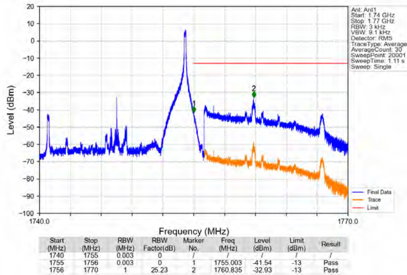
Band4_15MHz_QPSK_HCH_1747.5MHz_RB_1_74_NTNV
