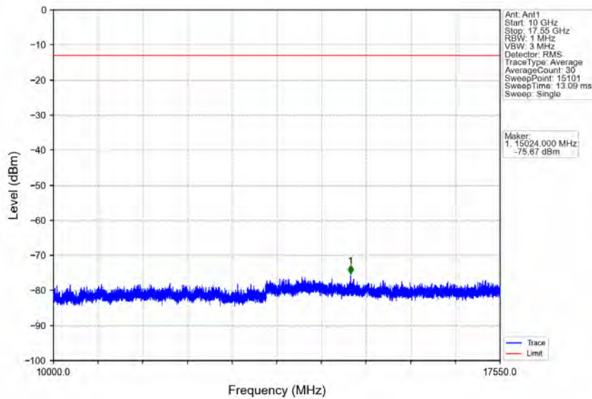
Band4_20MHz_16QAM_LCH_1720MHz_RB_100_0_NTNV
