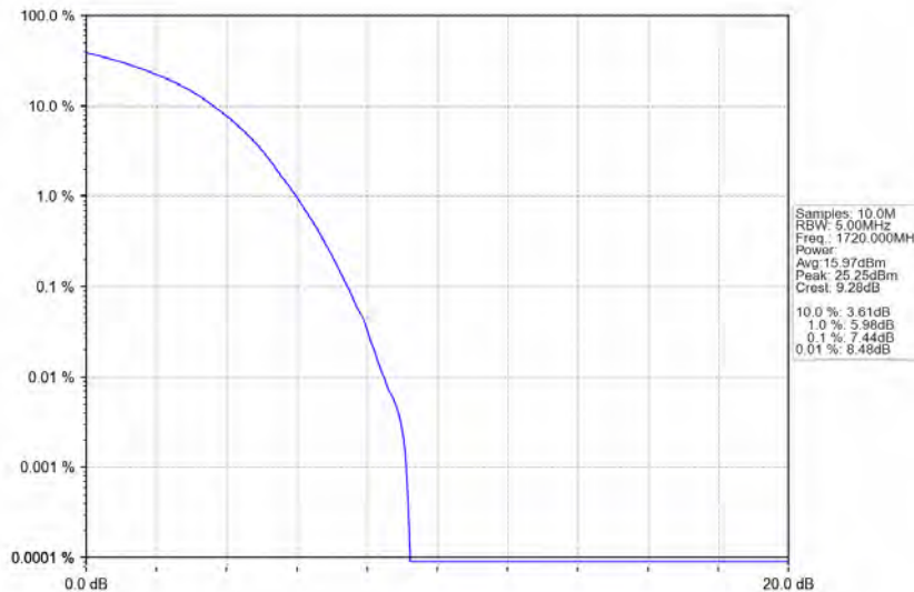
Band4_20MHz_16QAM_LCH_1720MHz_RB_100_0_NTNV
