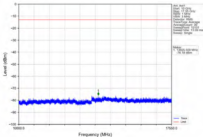
Band4_20MHz_QPSK_MCH_1732.5MHz_RB_1_0_NTV
