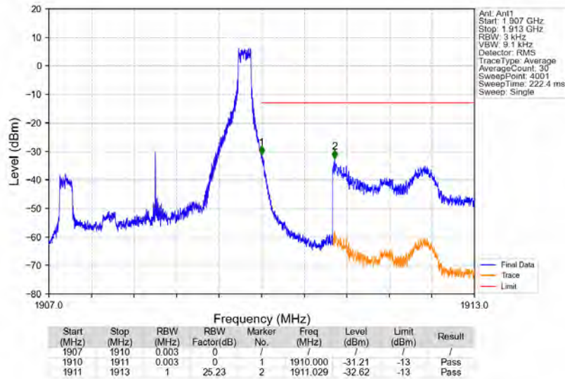
Band2_3MHz_QPSK_HCH_1908.5MHz_RB_1_14_NTNV
