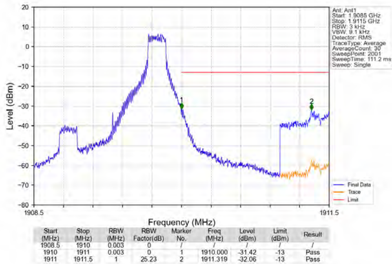
Band2_1.4MHz_QPSK_HCH_1909.3MHz_RB_1_5_NTV
