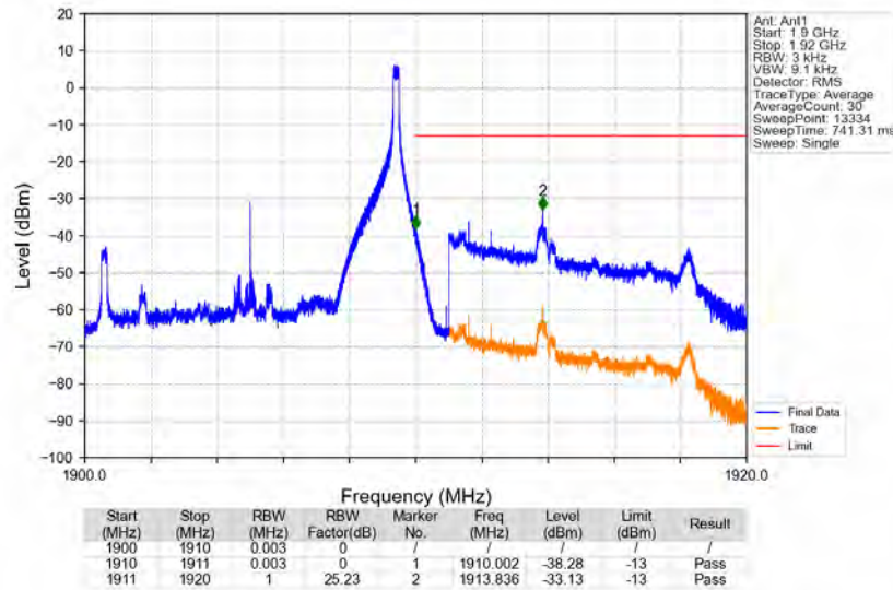
Band2_10MHz_QPSK_HCH_1905MHz_RB_1_49_NTNV
