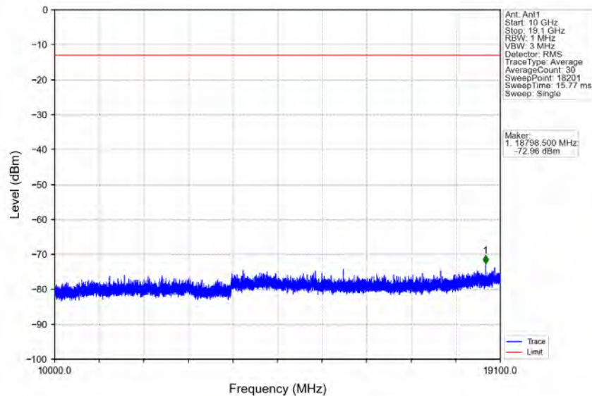
Band2_3MHz_16QAM_MCH_1880MHz_RB_1_0_NTNV
