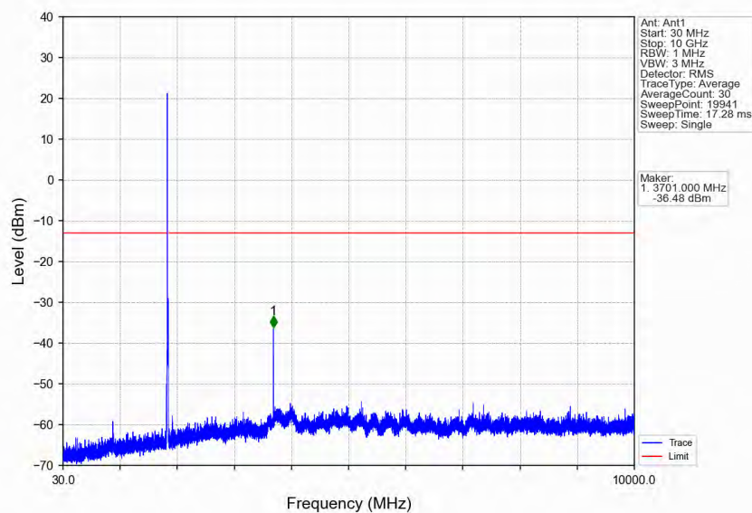
Band2_10MHz_16QAM_LCH_1855MHz_RB_1_0_NTNV
