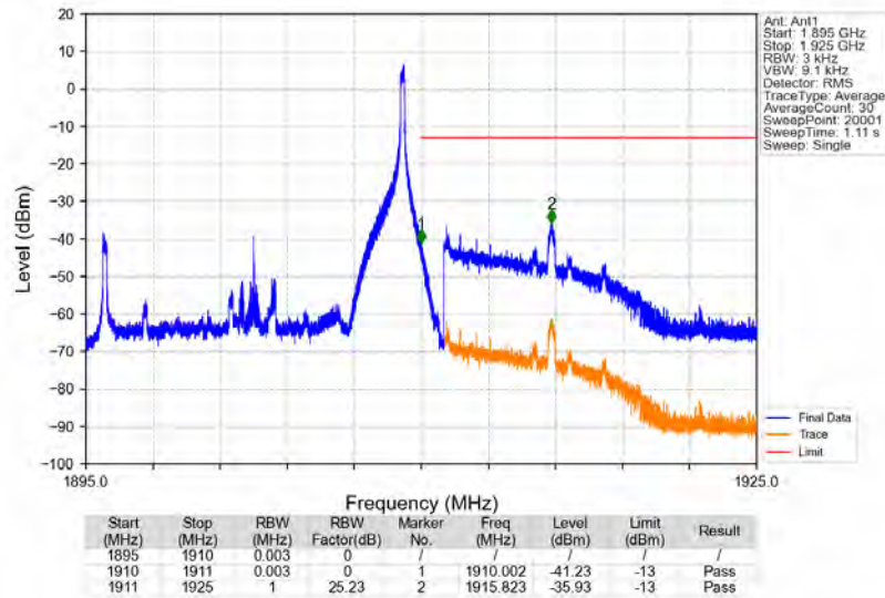
Band2_15MHz_16QAM_HCH_1902.5MHz_RB_1_74_NTNV
