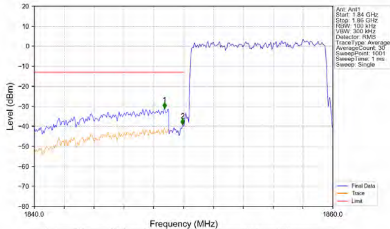
Band2_10MHz_16QAM_LCH_1855MHz_RB_50_0_NTNV
