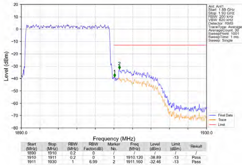
Band2_20MHz_QPSK_HCH_1900MHz_RB_100_0_NTNV
