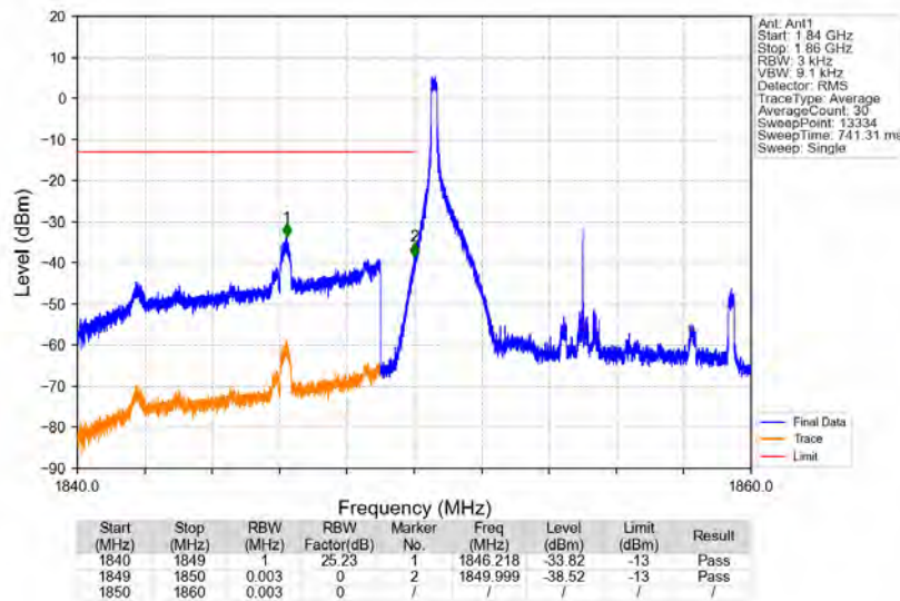
Band2_10MHz_16QAM_LCH_1855MHz_RB_1_0_NTNV
