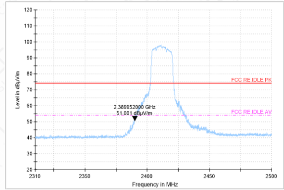
AV detector
