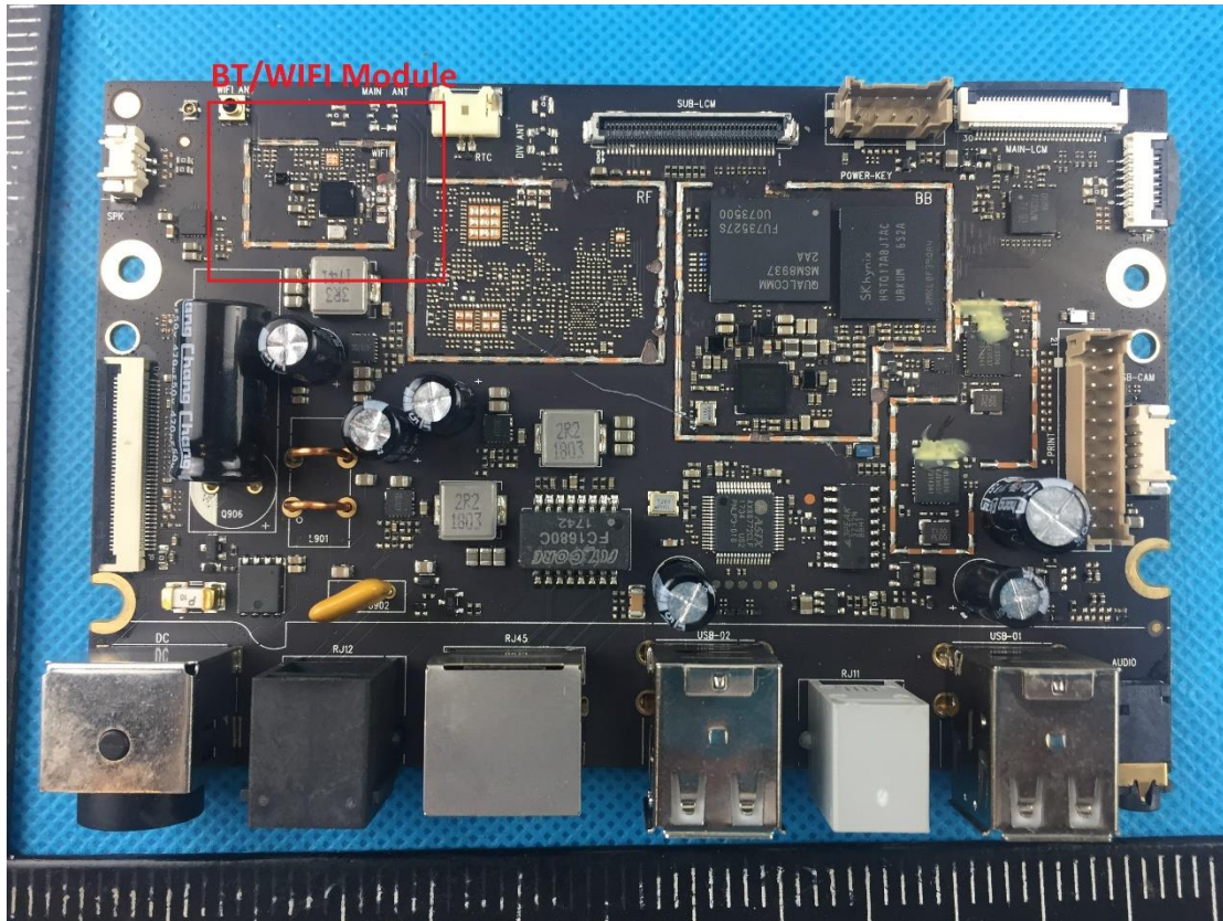
BT/WIFI Module: WCN3660B
