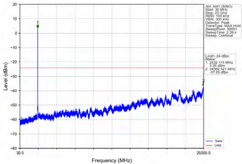
802.11g MCH 2437MHz Ant1 (SISO) NTVN
