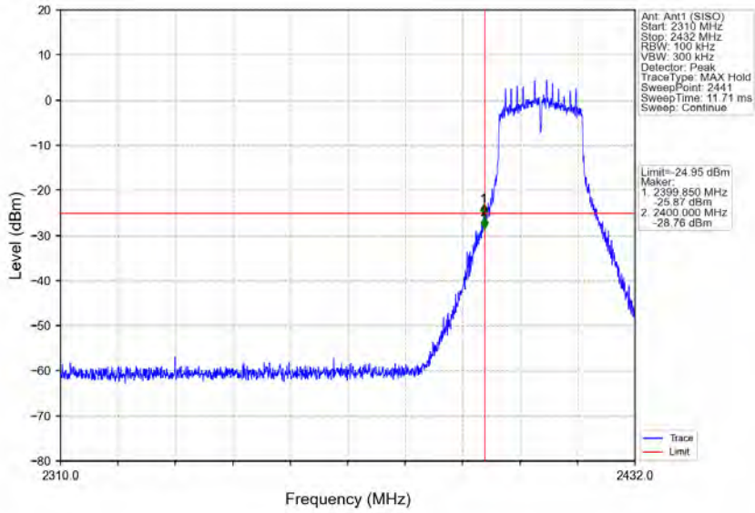
802.11n(HT20) LCH 2412MHz Ant1 (SISO) NTVN
