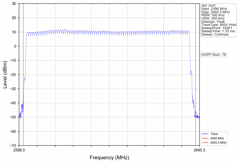
8DPSK_3DH5_HOPP_Ant1_NTNV
