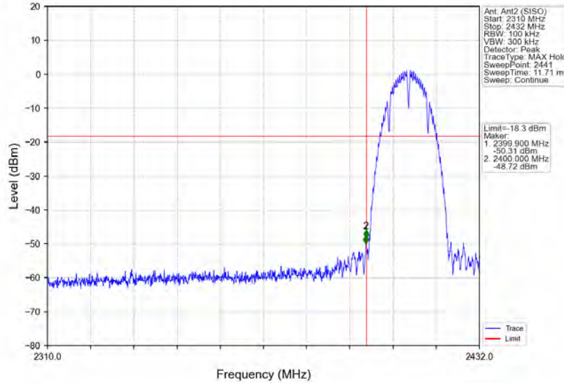
802.11b_LCH_2412MHz_Ant2 (SISO)_NTNV
