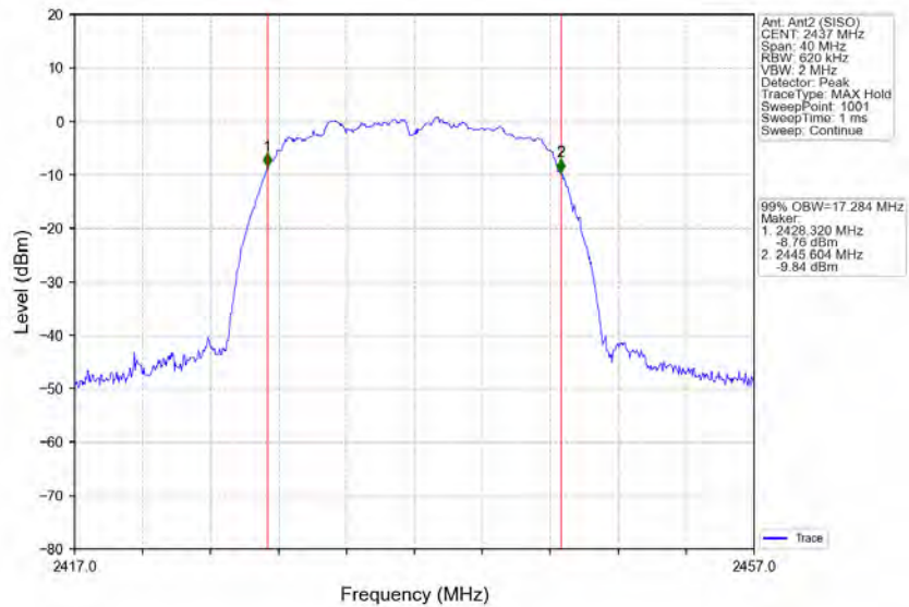
802.11g_MCH_2437MHz_Ant2 (SISO)_NTNV
