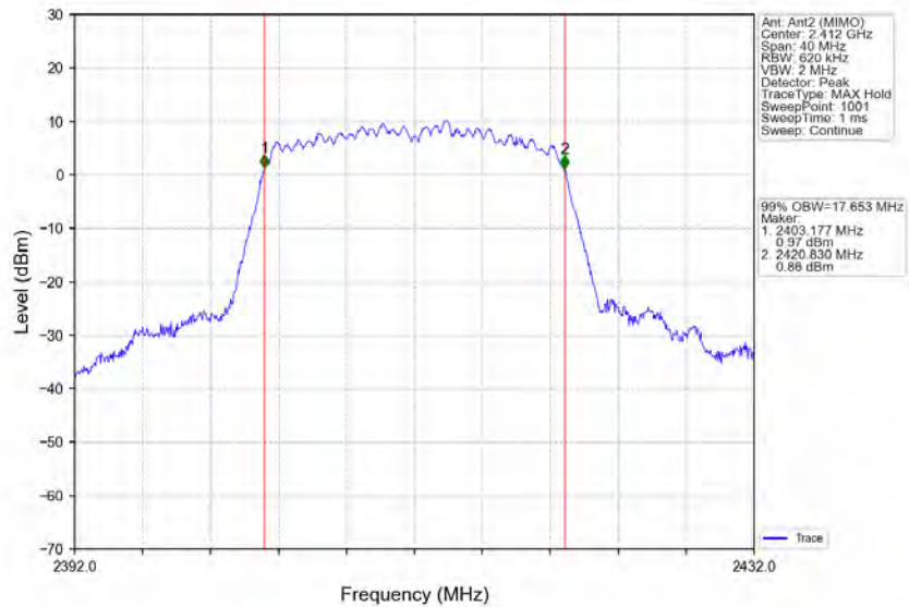
802.11n(HT20)_LCH_2412MHz_Ant2 (MIMO)_NTNV
