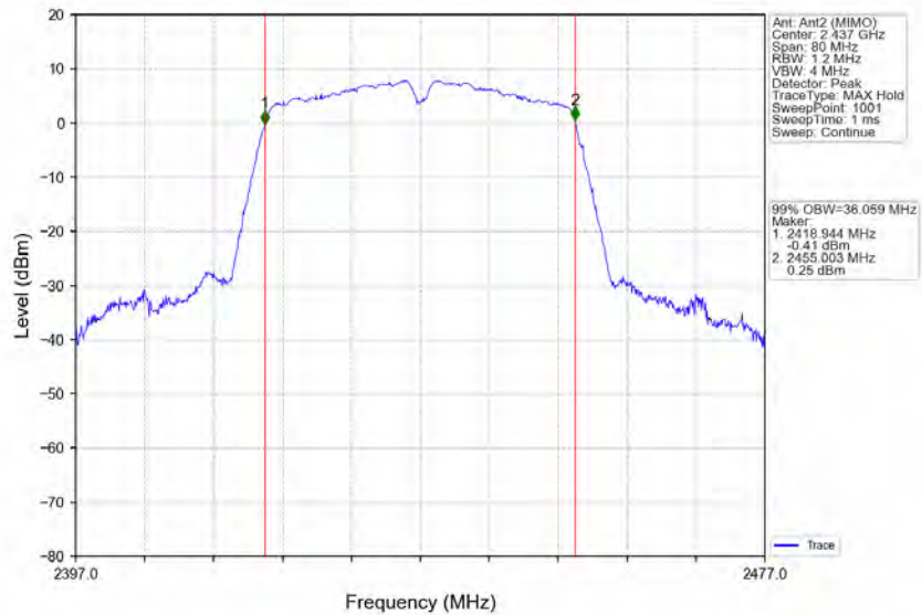
802.11n(HT40)_MCH_2437MHz_Ant2 (MIMO)_NTNV
