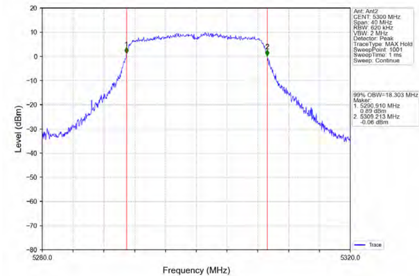
802.11n(HT20)_MCH_5300MHz_Ant2_NTNV
