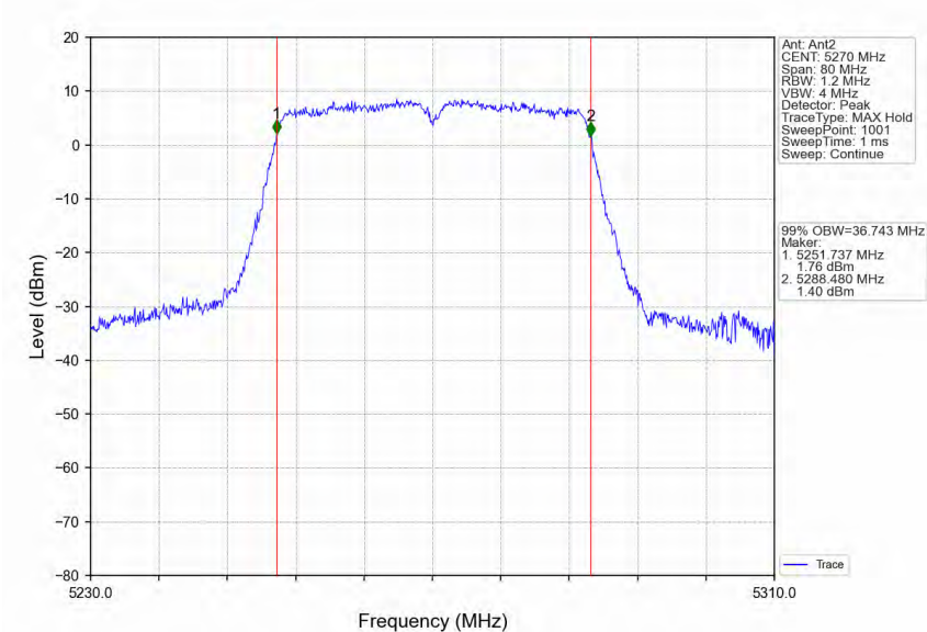
802.11n(HT40)_LCH_5270MHz_Ant2_NTNV
