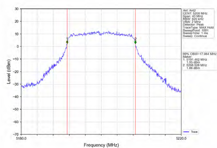
802.11a_MCH_5200MHz_Ant2_NTNV
