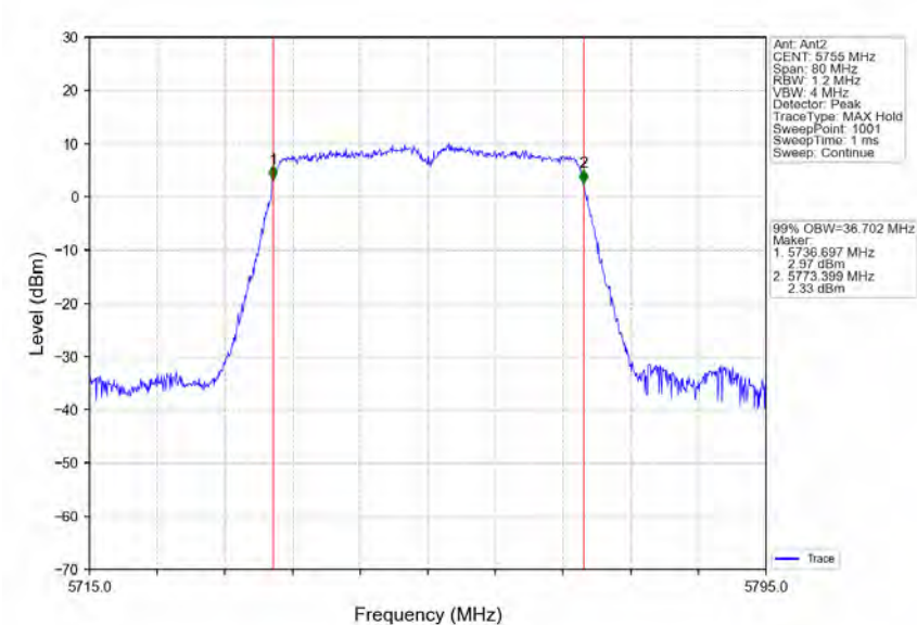
802.11n(HT40)_LCH_5755MHz_Ant2_NTNV
