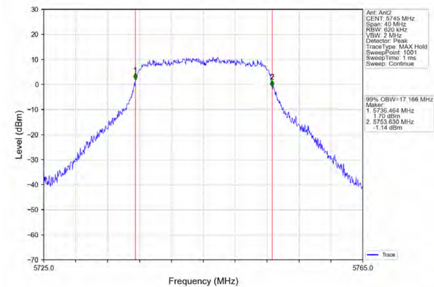
802.11a_LCH_5745MHz_Ant2_NTNV
