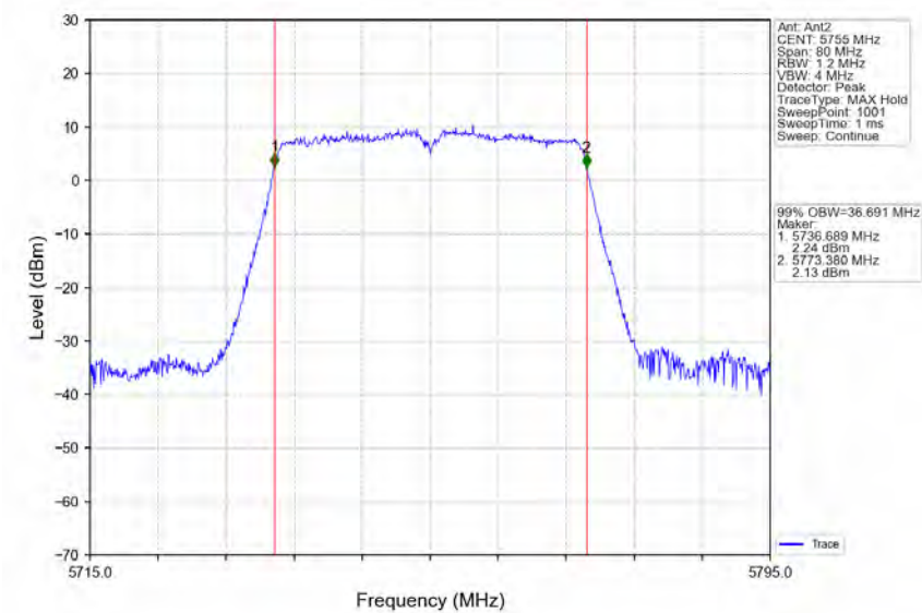
802.11n(HT40)_LCH_5755MHz_Ant2_NTNV
