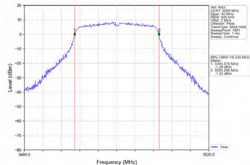
802.11n(HT20)_LCH_5500MHz_Ant2_NTNV
