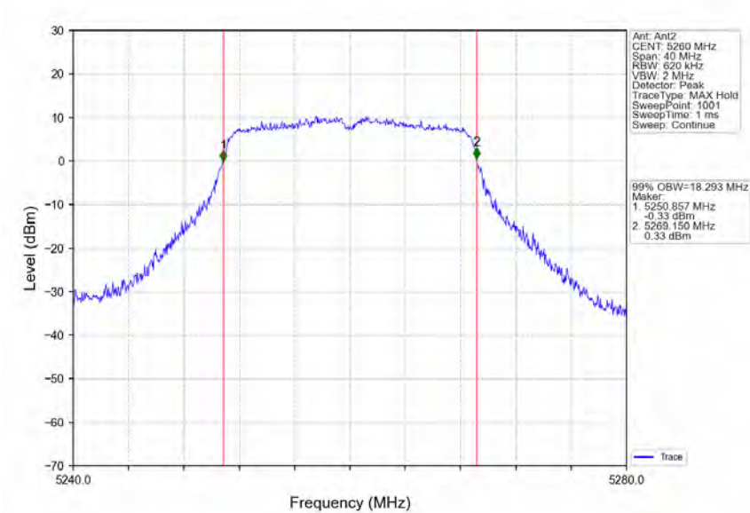
802.11n(HT20)_LCH_5260MHz_Ant2_NTNV
