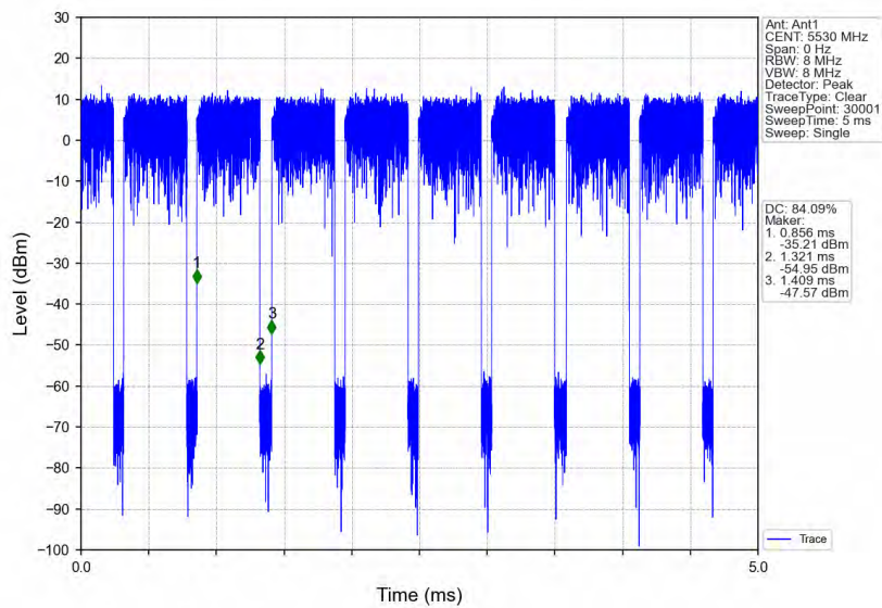
802.11ac(VHT80)_LCH_5530MHz_Ant1_NTNV
