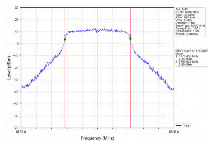
802.11a_MCH_5785MHz_Ant2_NTNV
