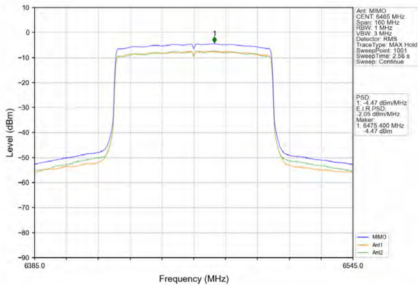
802.11ax(HEW80)_LCH_6465MHz_RU996_Left_MIMO_NTNV
