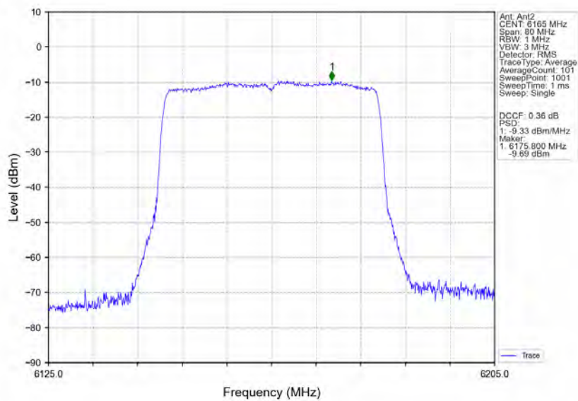
802.11ax(HEW40)_MCH_6165MHz_RU484_Left_Ant2_NTNV
