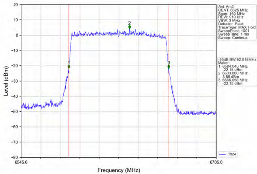
802.11ax(HEW80)_LCH_6625MHz_RU996_Left_Ant2_NTNV
