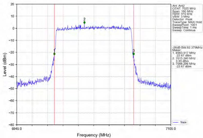
802.11ax(HEW80)_HCH_7025MHz_RU996_Left_Ant2_NTNV
