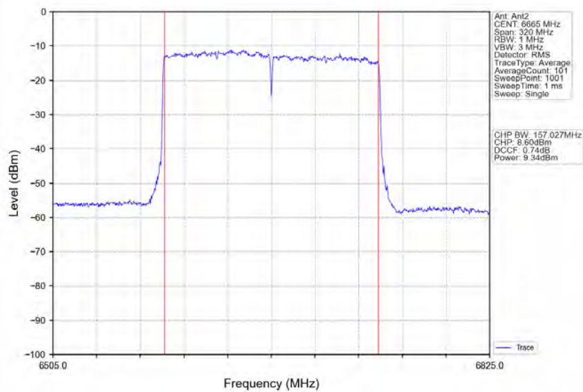
802.11ax(HEW160) MCH_6665MHz_2xRU996_Left_Ant2_NTNV
