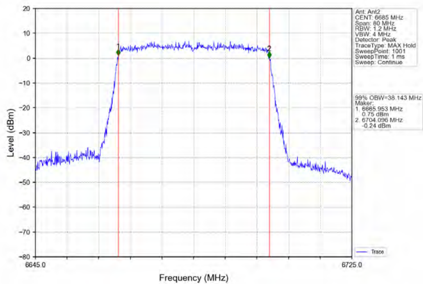
802.11ax(HEW40)_MCH_6685MHz_RU484_Left_Ant2_NTNV
