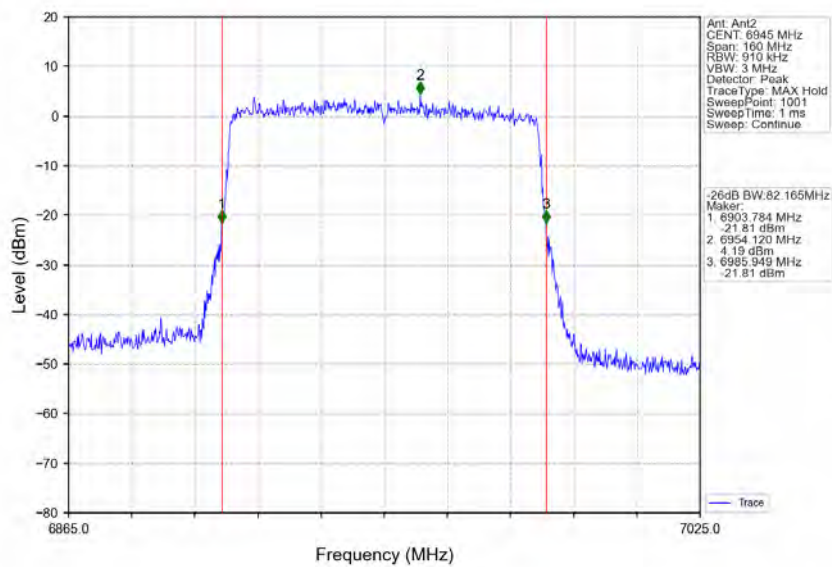
802.11ax(HEW80)_LCH_6945MHz_RU996_Left_Ant2_NTNV
