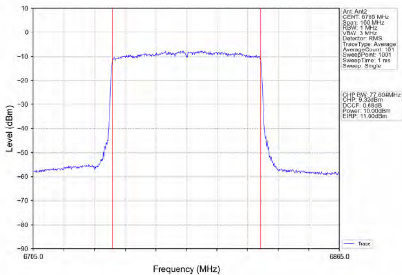
802.11ax(HEW80)_HCH_6785MHz_RU996_Left_Ant2_NTNV
