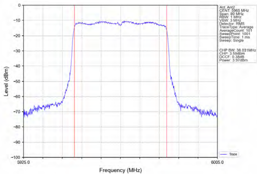
802.11ax(HEW40)_LCH_5965MHz_RU484_Left_Ant2_NTNV
