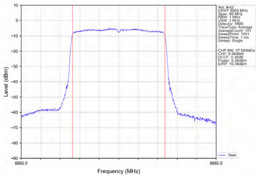
802.11ax(HEW40)_LCH_6925MHz_RU484_Left_Ant2_NTNV
