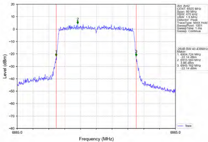
802.11ax(HEW40)_LCH_6925MHz_RU484_Left_Ant2_NTNV
