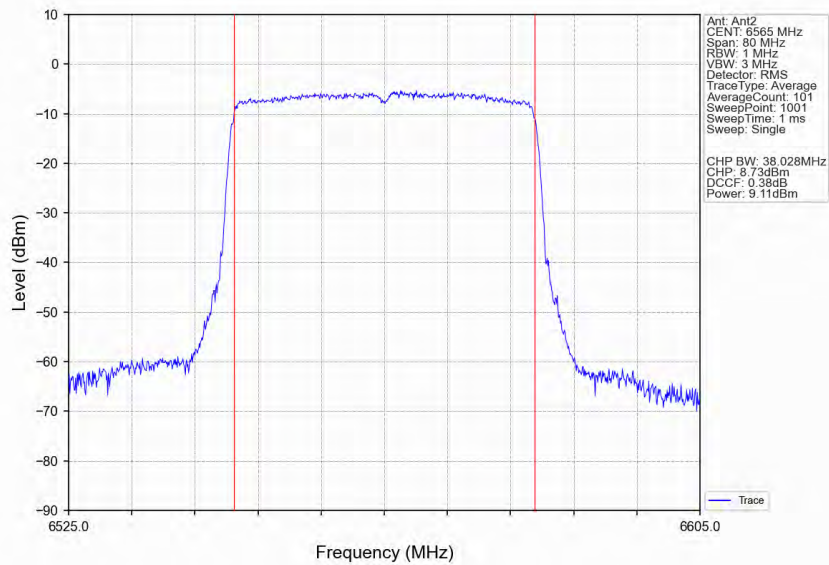
802.11ax(HEW40)_LCH_6565MHz_RU484_Left_Ant2_NTNV
