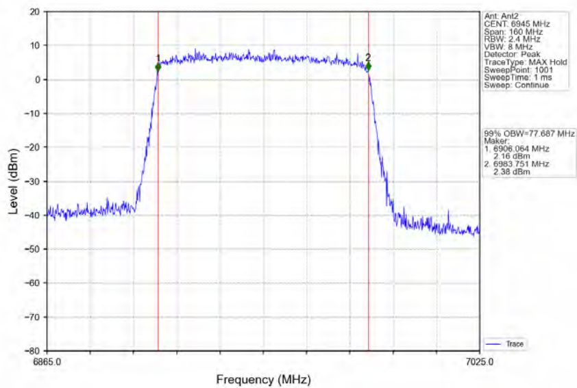
802.11ax(HEW80)_LCH_6945MHz_RU996_Left_Ant2_NTNV
