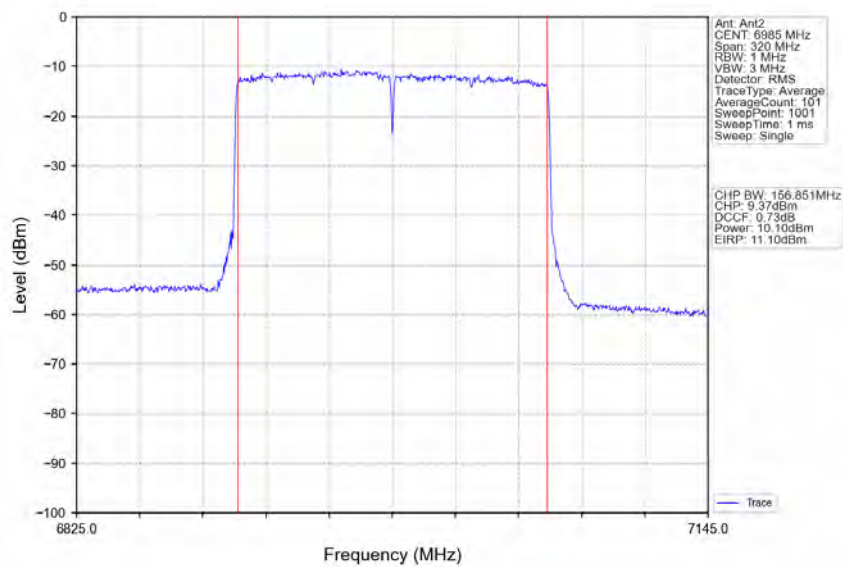
802.11ax(HEW160) MCH_6985MHz_2xRU996_Left_Ant2_NTNV
