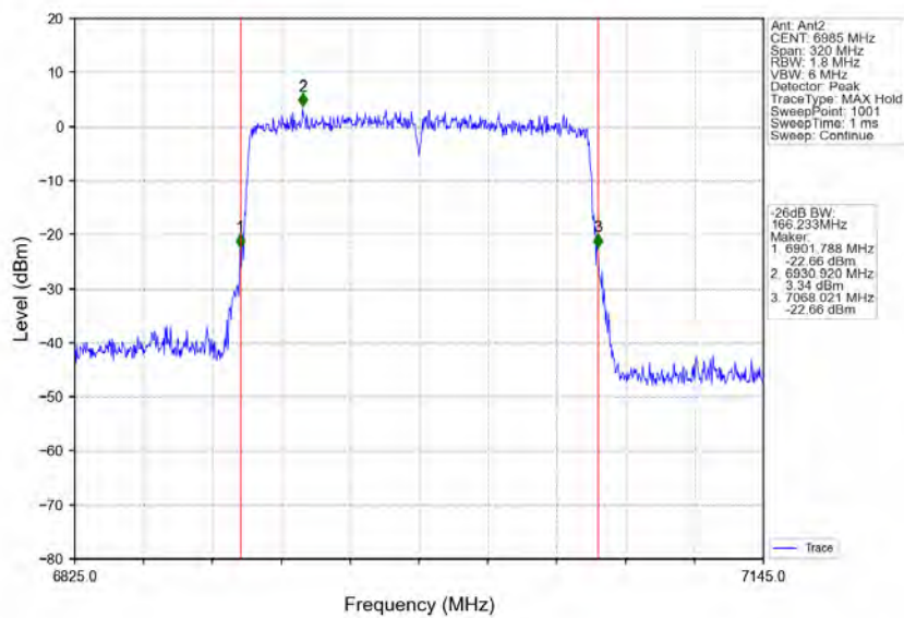
802.11ax(HEW160) MCH_6985MHz_2xRU996_Left_Ant2_NTNV
