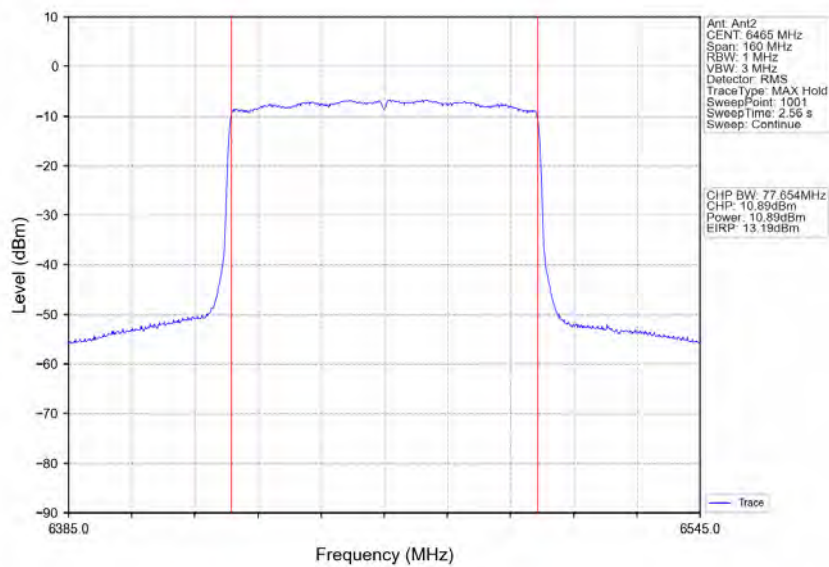
802.11ax(HEW80)_LCH_6465MHz_RU996_Left_Ant2_NTNV
