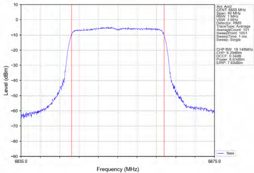
802.11ax(HEW20)_HCH_6855MHz_RU242_Left_Ant2_NTNV
