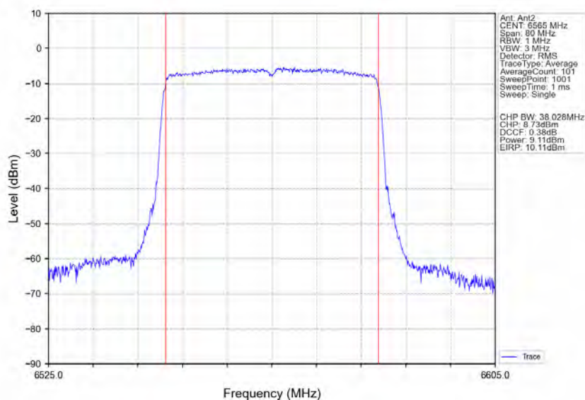
802.11ax(HEW40)_LCH_6565MHz_RU484_Left_Ant2_NTNV
