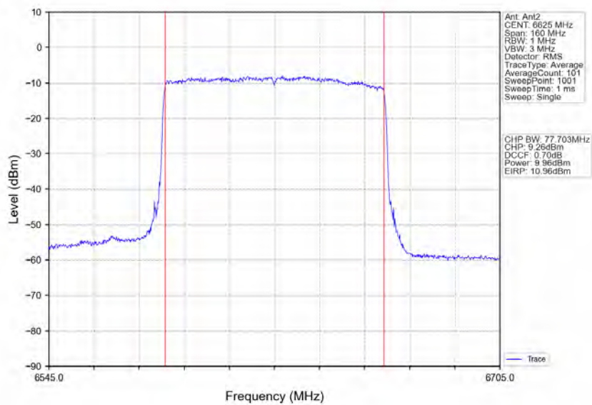
802.11ax(HEW80)_LCH_6625MHz_RU996_Left_Ant2_NTNV
