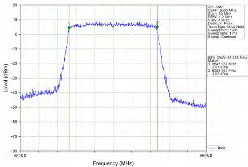
802.11ax(HEW40)_LCH_6565MHz_RU484_Left_Ant2_NTNV
